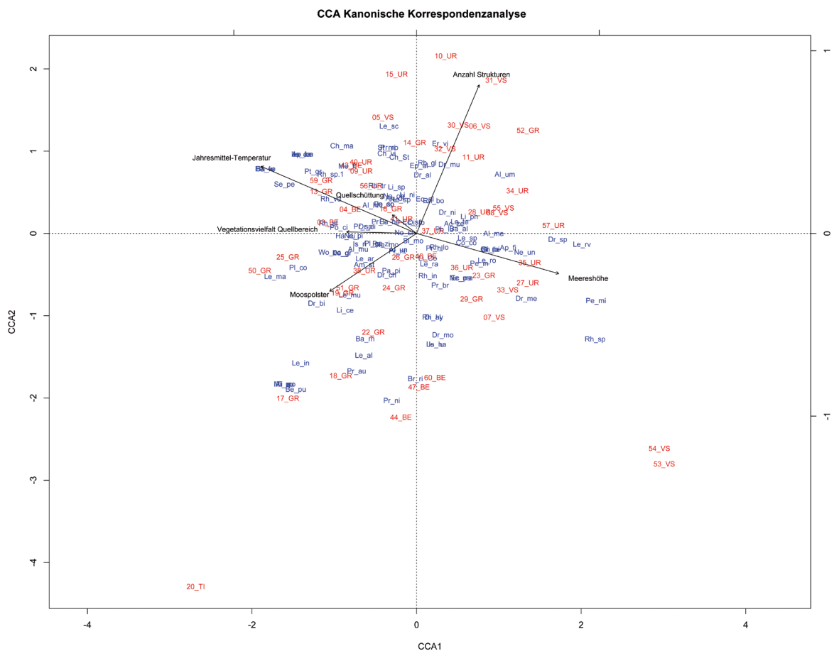
Abb. 5: Kanonische Korrespondenzanalyse (CCA): Triplot der Anzahl EPT-Taxa, der Quellen sowie der Parameter Jahresmittel der Wassertemperatur, Meereshöhe, Quellschüttung, Vegetationsvielfalt, Anzahl Strukturen und Deckung der Moospolster (n=49).
