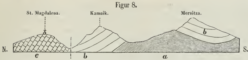
Im Kolkgraben, rechtes Thalgehänge.
