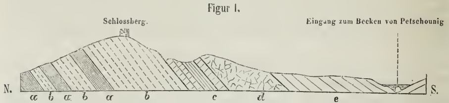
Profil des Schlossberges bei Cilli längs der Eisenbahn.
