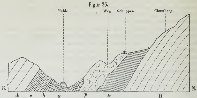
Profil beim Reyer'schen Kohlenbau (hinter Tüffer).
