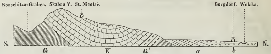
Profil längs des Nikolai-Grabens.
