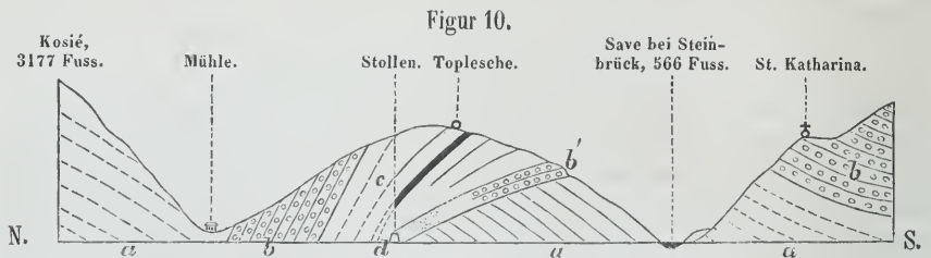
Tertiärgebirge bei Steinbrück.
