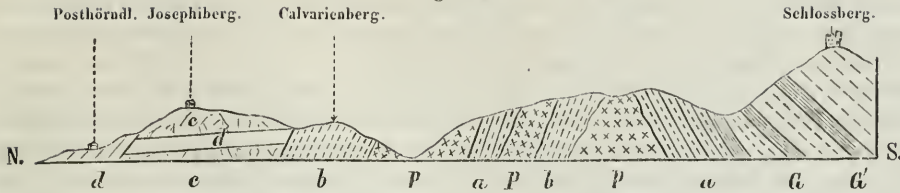
Profil vom Josephberg zum Schlossberg (nördl. Fortsetzung von Fig. 1).
