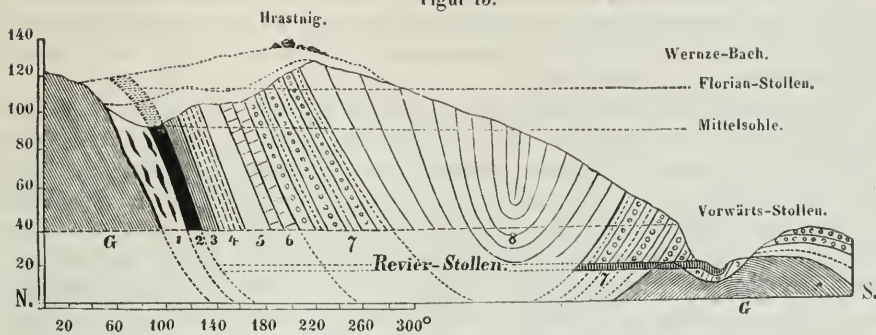
Profil des Kohlenbeckens von Hrastnig.
