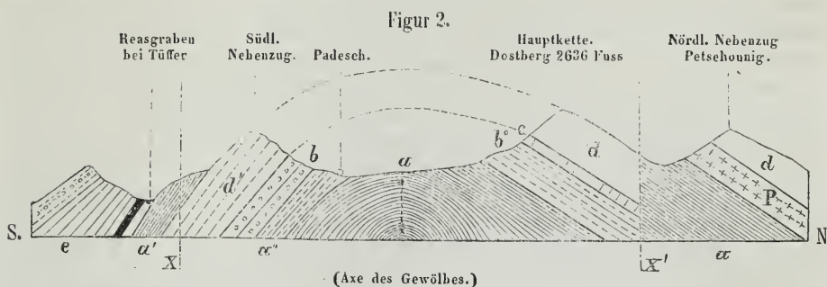
a Gailthaler Schiefer. a Gailthaler Schiefer, dem Dolomit aufgelagert. a° Gailthaler Sandstein mit Bleiglanz. b Werfener Conglomerat. b° Werfener Schiefer. c Guttensteiner Kalk. d Hallstätter Kalk. d° Hallstätter Dolomit. e Tertiärschichten. P Porphy.
