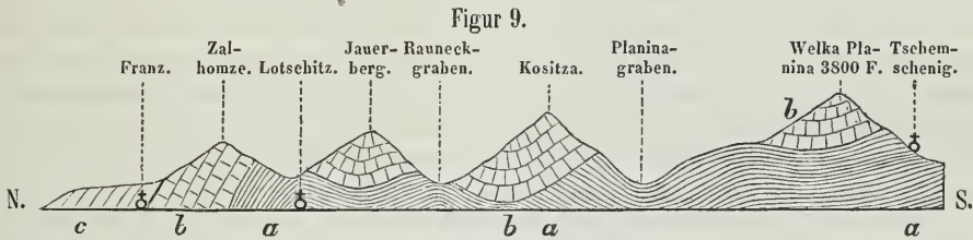
Profil im Meridian von Franz.
