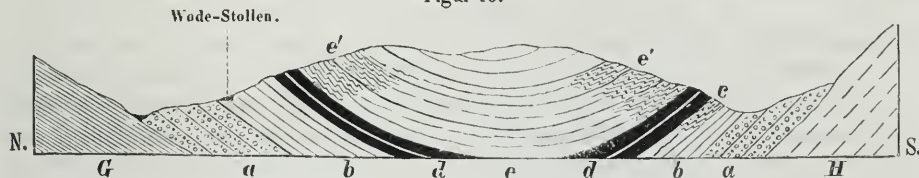
Idealer Durchschnitt des Trifailer Beckens.
