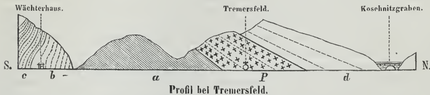
a Gailthaler Schiefer. b Dolomit, Gutensteiner Kalk. c Kalkschiefer, Gutensteiner Kalk. d Hallstätter Dachstein-Kalk. P Porphyre und Tuffsandsteine.
