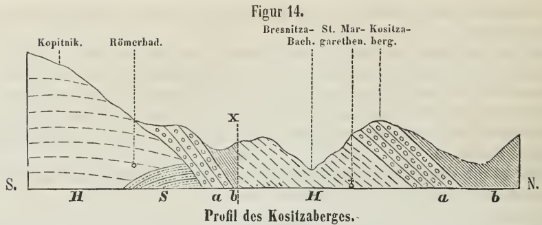
S Werfener und Gailthaler Schichten. H Hallstätter Dolomit, deutlich geschichtet. a Leithakalk. b Mergelschiefer.
