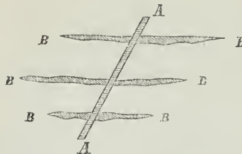
A A Taube Kluft. B Erzlinsen.
