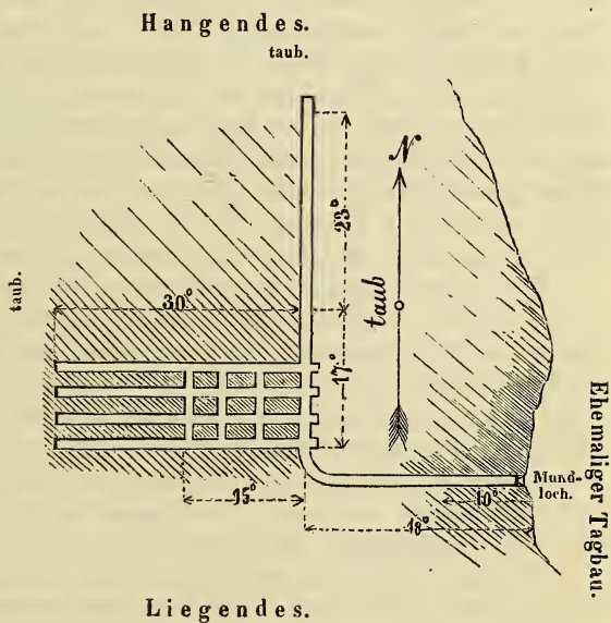
Grundriss des Eisensteinbaues von Olimie bei Windisch-Landsberg.
