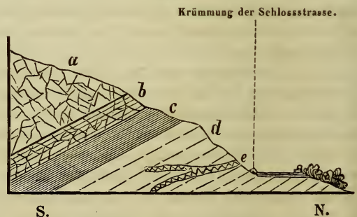
Profil an der Schlossstrasse von Windisch-Landsberg.
