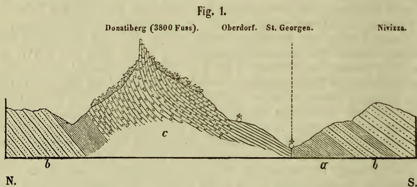
Profil durch die mittlere Kuppe des Donatiberges.
