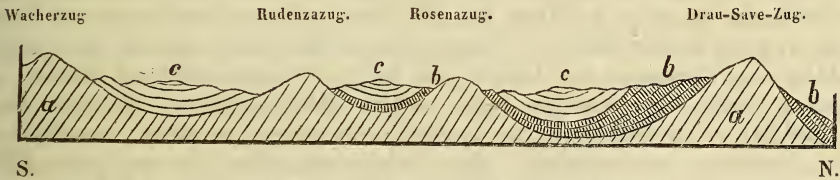
Verbreitung der Eocenformation im Cillier Becken.
