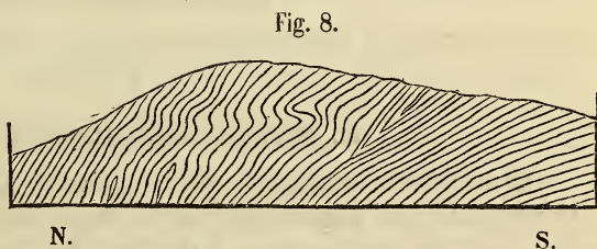
Schichtenwindung der Gailthaler Schiefer bei Laak.
