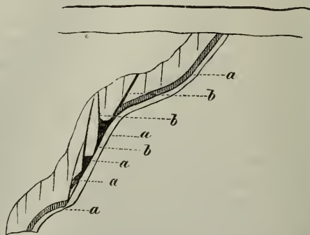
Ansicht des rechten Ulms im Abteufen am Mariengang unter der Pflugenstollensohle.
