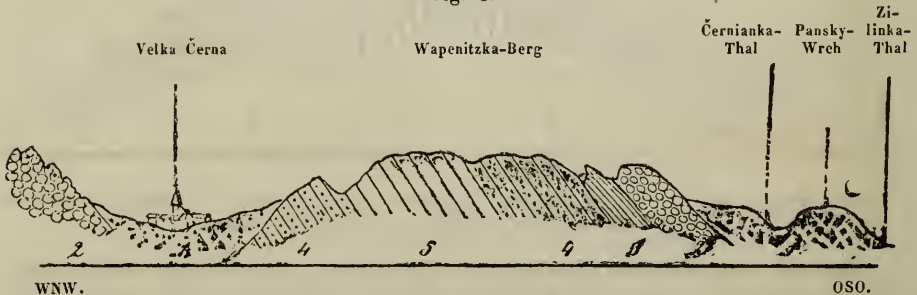
1. Eocenmergel. 2. Eocenconglomerat. 3. Grauer dünngeschichteter Mergelkalk (Neocom). 4. Dolomit. 5. Lichtgrauer Kalk (Jura).
