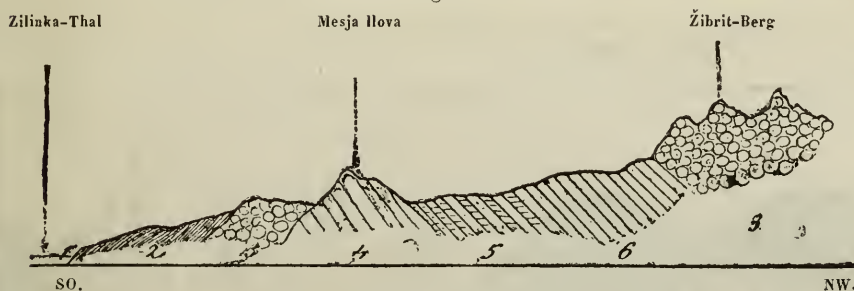
1. Alluvium des Zilinkafusses. 2. Eocenmergel und Sandstein. 3. Eocenconglomerate 4. Neocommergel. 5. Crinoidenführender Kalk und Kalksandstein. 6. Schiefer.
