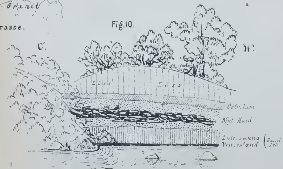
Thal v. Kühlenring, links zweite Entblössung.
