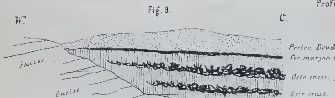
Profil des Judenfriedhofgrabens.
