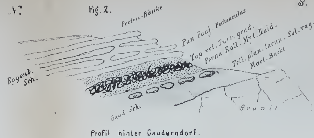
Profil hinter Gauderndorf.
