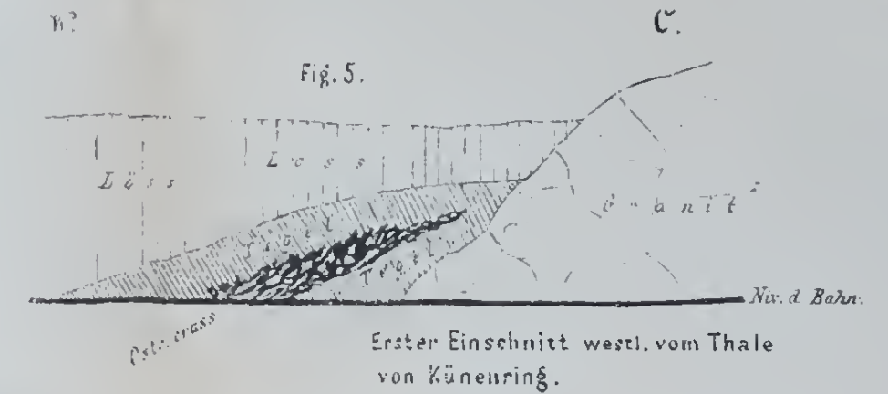
Profil vor Gauderndorf.
