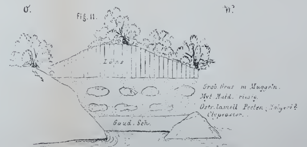
Thal v. Kühlenring, links erste Entblössung.
