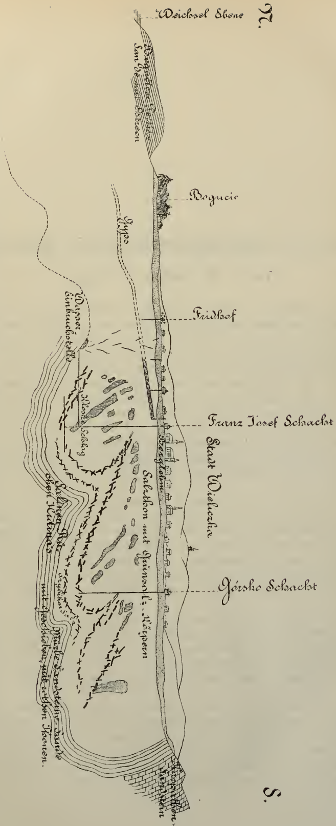
Die Schraffirungen zwischen dem „Salzhon mit Gips und Spathstein“ und dem „Spinasalz“ zeigen die Spinasalzlager an.
