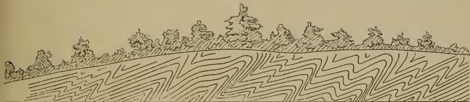
Liegendpartie der Reiflingerkalke an der Strasse von Hafnerberg nach Neuhaus.
