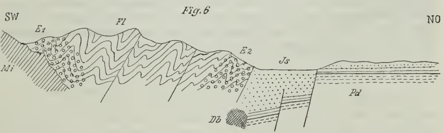
C. Schematisirte Durchschnitte zur Erläuterung der geologischen Geschichte der Ostkarpathen.
