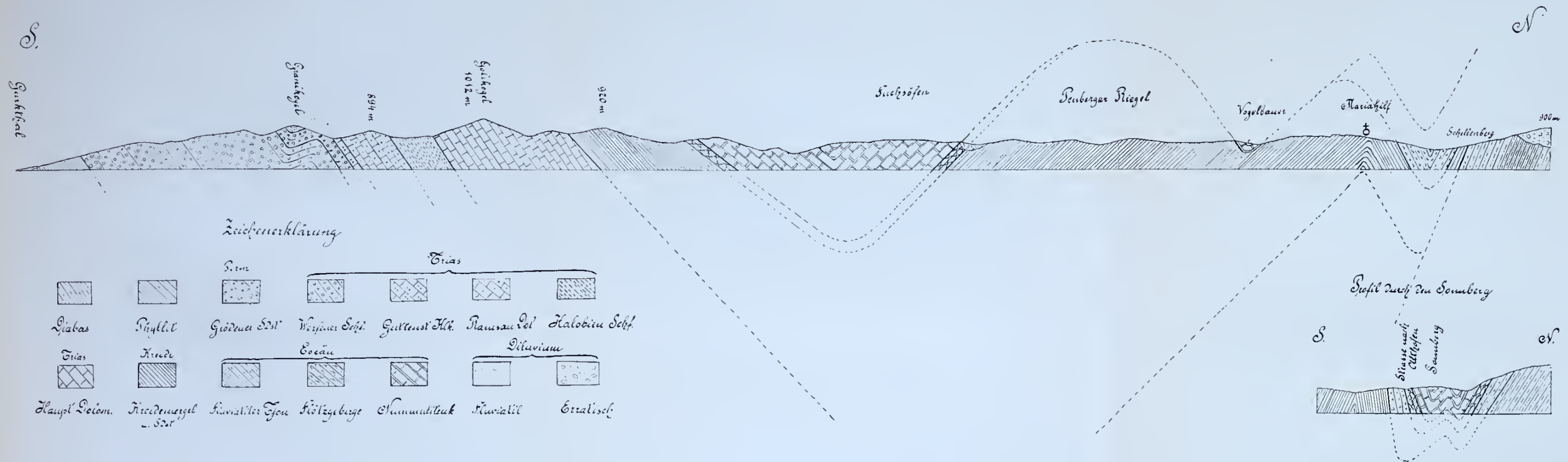
Profil durch die Berge der Westlehn des Görtscitztales.
