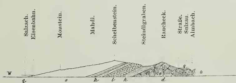
Profil durch den Scheibenstein und das Raucheck.
