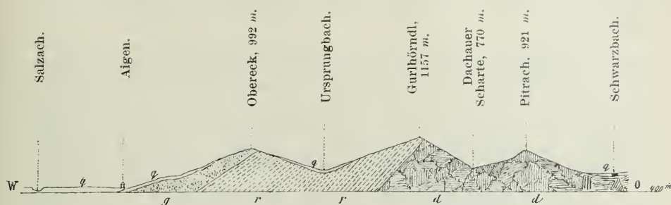
Profil durch Obereck und Gurthörndl.
