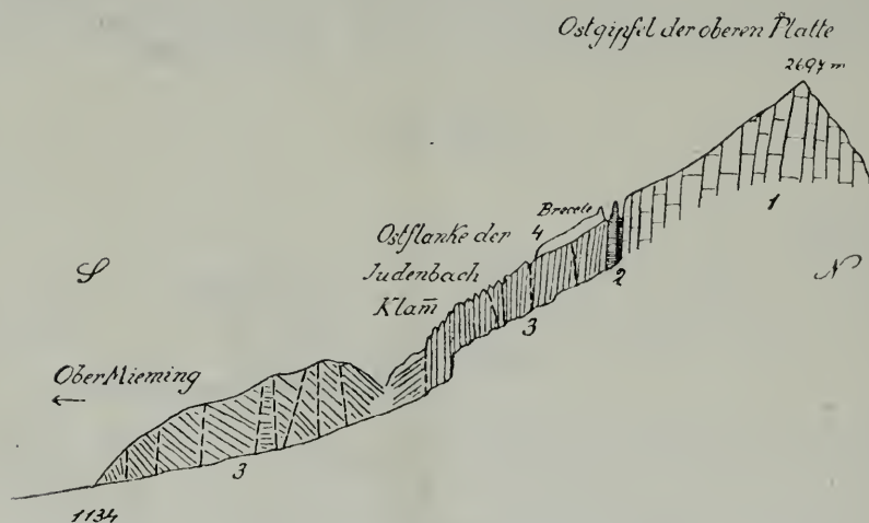
Profil XVII.
