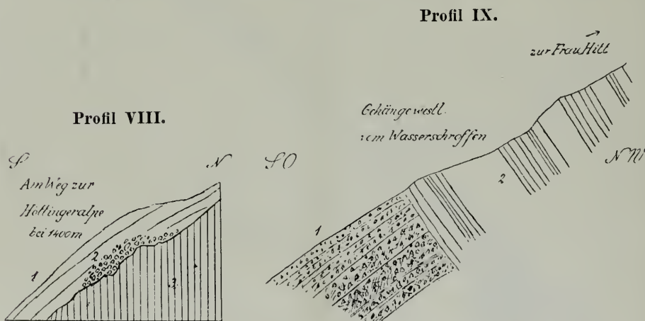
Profil VIII: 1. Höttingerbreccie. — 2. Loses Schuttwerk. — 3. Grundgebirge.
