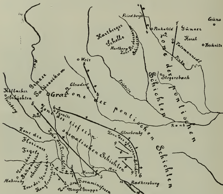
Tektonische Skizze der mittelsteirischen Tertiärbucht.
