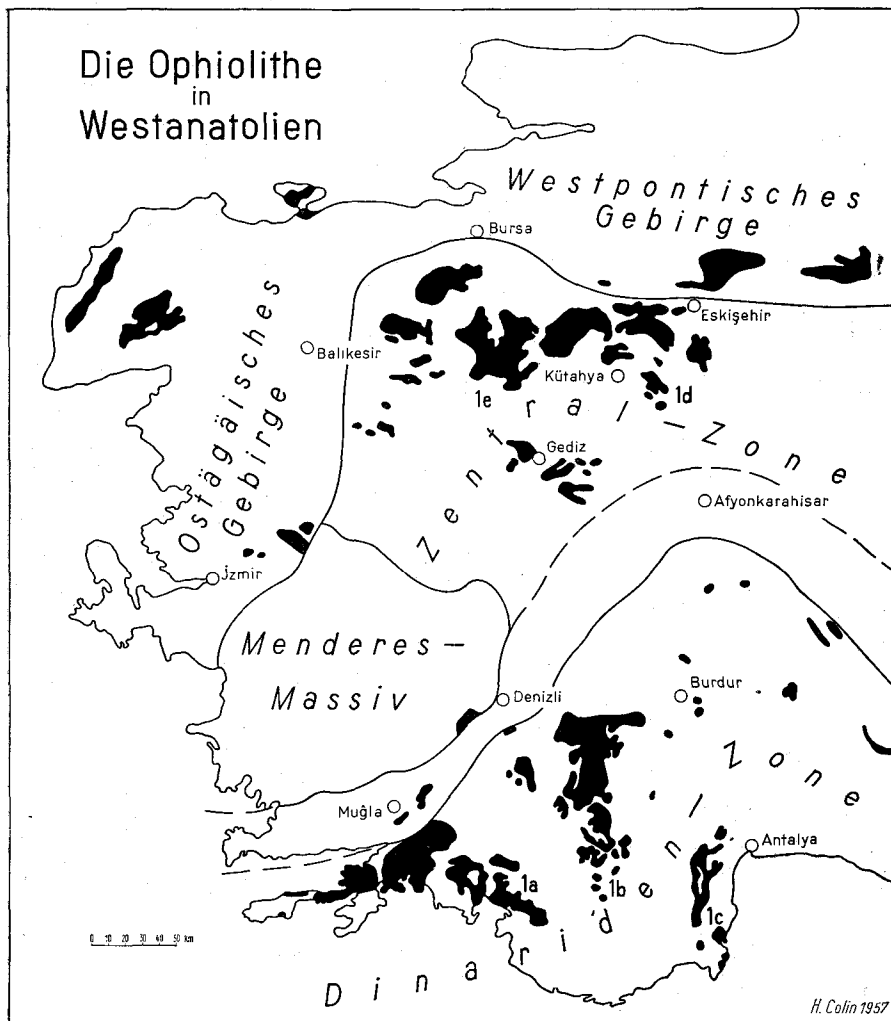
Abb. 2 gibt die Verbreitung der Ophiolithe (schwarz) in Westanatolien. Die Ziffern 1a—1e der Karte beziehen sich auf die entsprechenden Abschnitte im Text. (1a: Fethiy e, 1b: Elmali-Akdağ, 1c: Alakırçay-Tal, 1d: Çekürler-Söğütyaylaköy 1e: westlich Kütahya).
