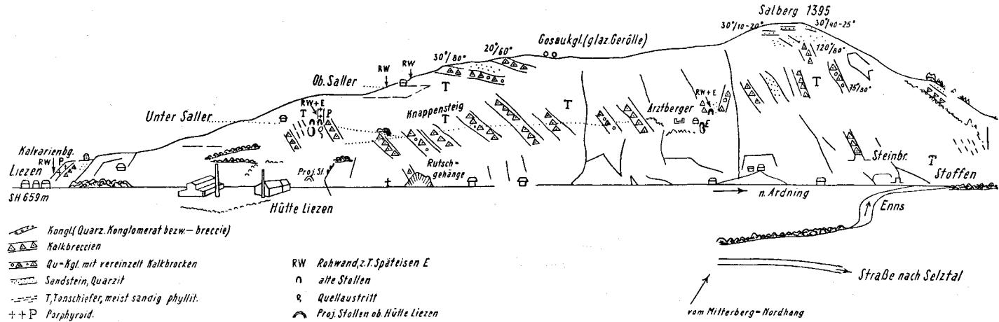
Abb. 6: Geologische Ansicht des Salberges bei Liezen, gesehen vom Mitterberghang aus südlich der Enns.
