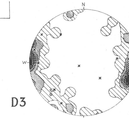
D3 Faltenachendiagramm Hauptquerschlag 110 B-Achsen, Stufen 2-5-8-11-16%, 1 Lineare (a)
