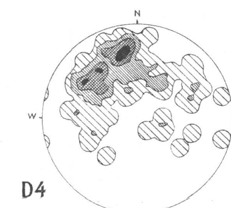
D4 Verwerfendiagramm E-Feld 104 Pole, Stufen 2-5-8-10%
