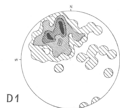
D1 Verwerfendiagramm W-Feld 52 Pole, Stufen 2-5-8-10%
