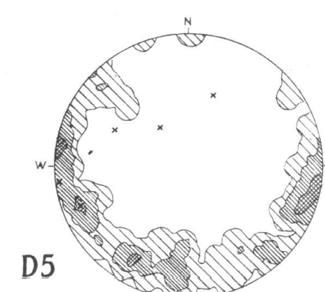
D5 Faltenachendiagramm E-Feld 91 B-Achsen, Stufen 2-5-8%, 1 Lineare (a)
