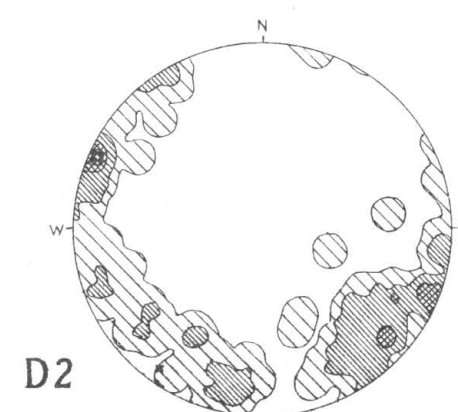
D2 Faltenachendiagramm W-Feld 89 B-Achsen, Stufen 2-5-8-11%, 1 Lineare (a)
