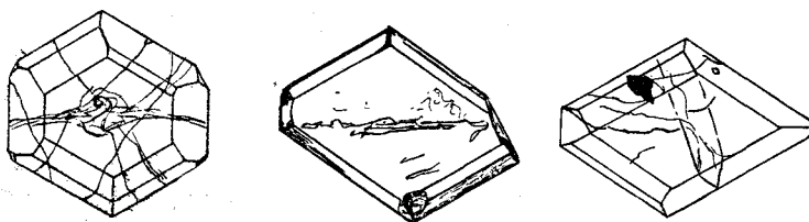
Abb. 6: Tafelige Ausbildung nach a (nach J. SLAVIK)
