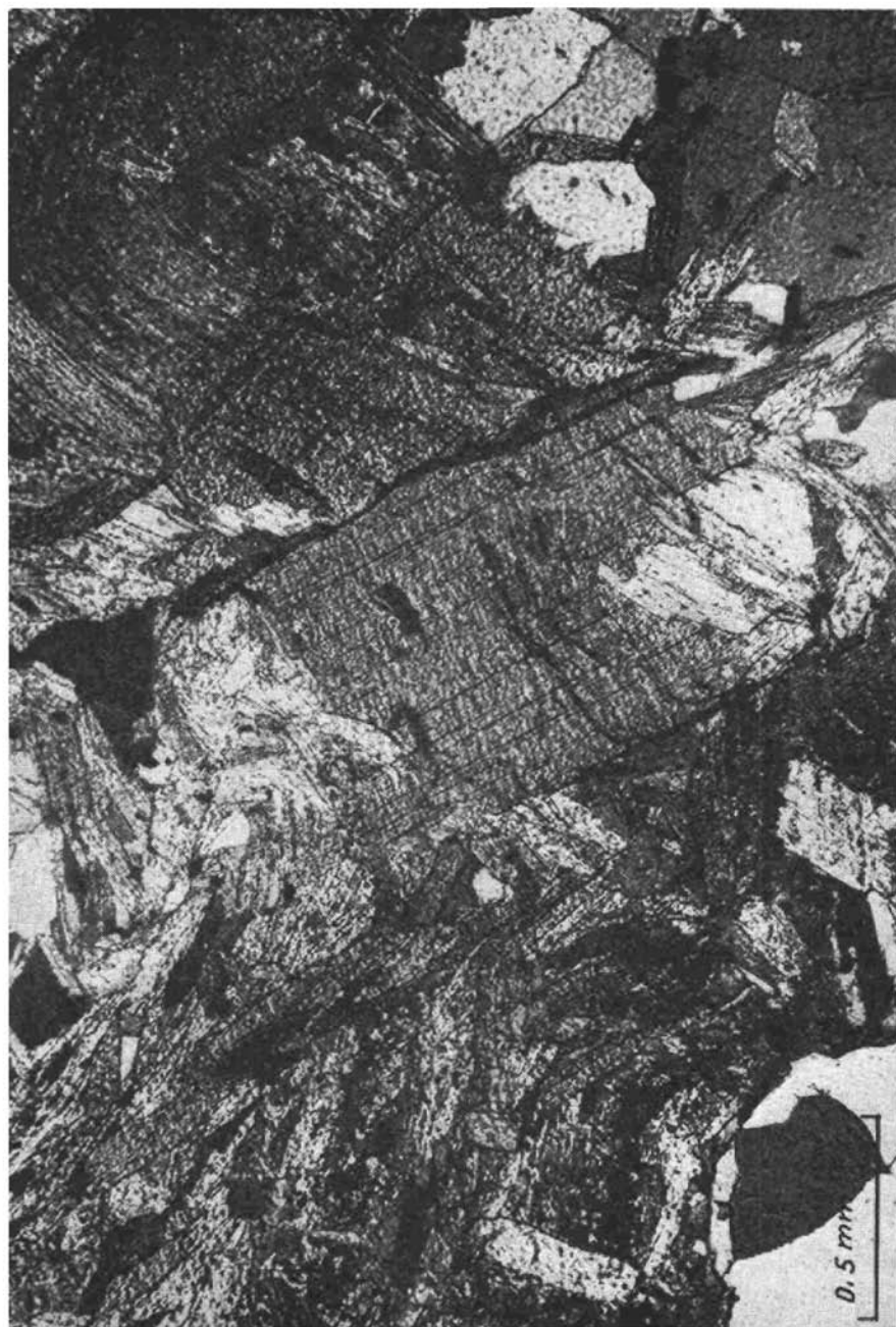
Abb. 4: Quermuskovit mit se -parallelem Interngefüge (Biotit, graphitisches Pigment). Die Muskovitfalten rechts davon sind stetig gekrümmt, in der linken Bildhälfte zeichnen sich dagegen Polygonalbögen ab. Granat-Glimmerschiefer von der Lehnkar-schneide (Höhe 2700 m).
