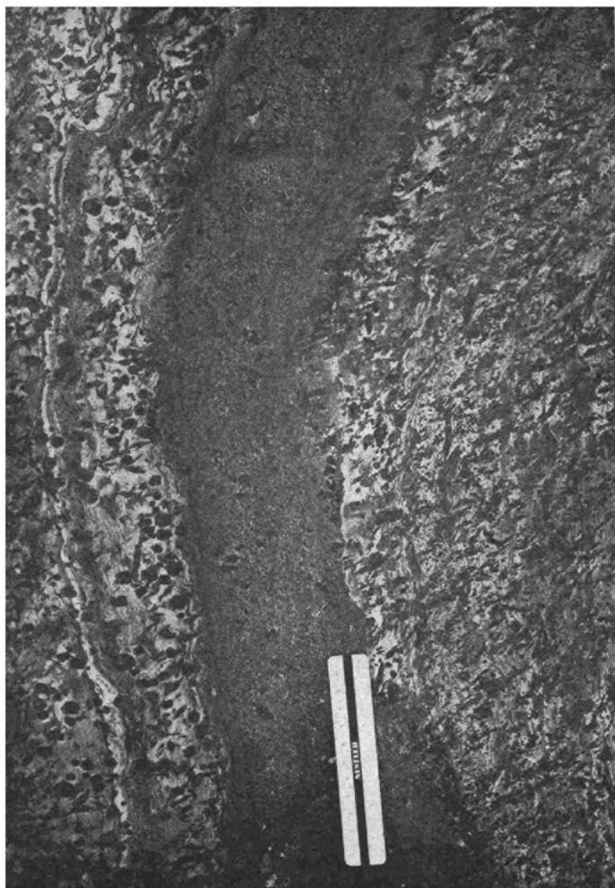
Abb. 7: Amphibolitlager in Gneisglimmerschiefern mit starker Granat- und Hornblendesprossung. Rechte Seite des Niedertales, 100 m nördlich des Schrabächle (Höhe 2412 m).
