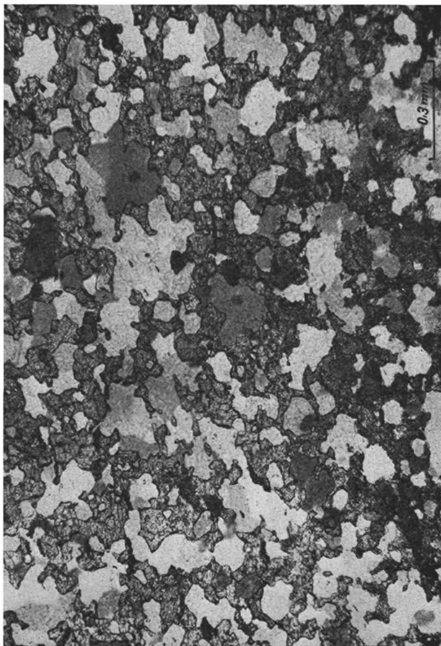
Abb. 6: Heller feinkörniger Kern eines Kalksilikatbandes in Biotit-Muskovit-Plagioklasgneisen an der Straße nördlich Vent, 250 m unterhalb der Mündung des Gießbaches. Die Quarzkörner werden von feinkristallinem Epidot bindemittelartig umgeben, so daß der Eindruck reliktscher Sedimentgefüge entsteht.
