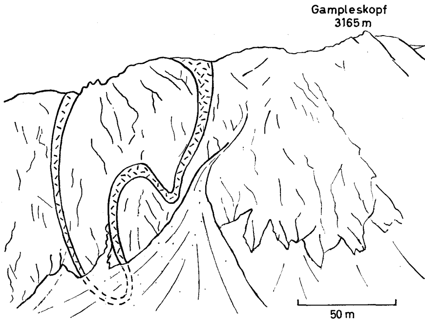
Abb. 11: Flasergranitgneis-Falte am Westgrat des Gampleskopfes ( B_1 = 172^\circ / 12^\circ S ).
