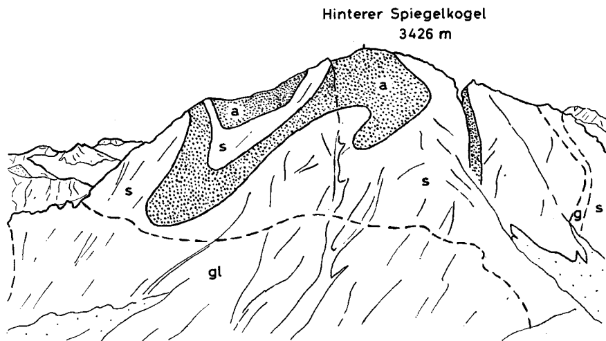
Abb. 10: Amphibolitfalte in der Südwand des Hinteren Spiegelkogels ( B_1 100^\circ / 20 bis 30^\circ NW). a = Amphibolit, s = Schiefergneis, bzw. Gneisglimmerschiefer, gl = graue mineralreiche Glimmerschiefer, g = granitischer Augengneis.
