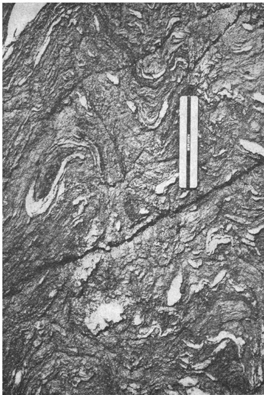
Abb. 8: Gefalteter Biotit-Muskovit-Plagioklasgneis mit s_1 -parallelen Quarzleukosomen. Die Quarzlinsen wurden zusammen mit der Hauptschieferung s_1 gefaltet. Auf dem Halwart, SSE des Weißkarkogels (Höhe 2340 m).
