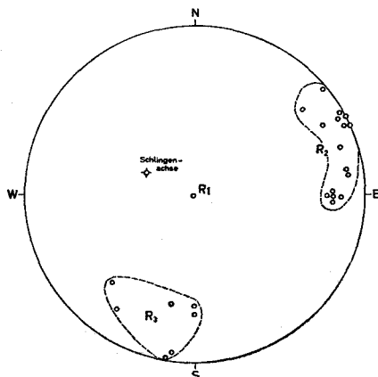
Abb. 13: Rotationsachsen (R) des Faltengefüges.
