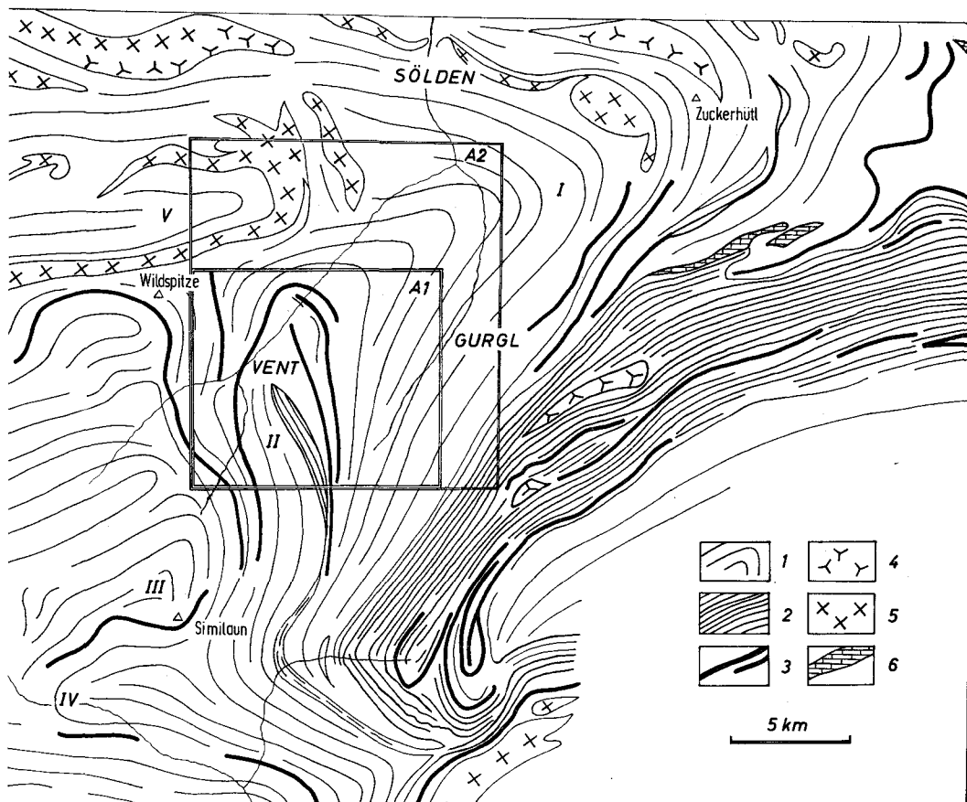
Abb. 1: Tektonische Übersichtskarte nach SCHMIDEGG (1933). 1. Paragneise und Glimmerschiefer. 2. Gesteine des Schneeberger Zuges. 3. Tektonische Leitgesteine (Gneise, Amphibolite, Marmore). 4. Tonalitische Gneise und Orthoamphibolite. 5. Granitgneise. 6. Zentralalpine Trias. I Stubai Schlinge, II Venter Schlinge, III Marzell-Schlinge, IV Schlingenbögen des Schnalstales, V Mittelberg-Schlinge.
