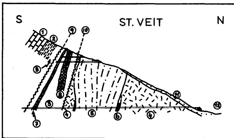
Abb. 35: Schematisches Profil durch die Lagerstätte St. Veit nach E. CLAR (1929). 1 = Wettersteinkalk, 2 = Partnachschichten, 3 = Muschelkalk, 4 = Hauptdolomit, 5 = Jura, 6 = Kössener Schichten, 7 = Spatgang, 8 = Haupterzzone, 9 = Hangender „Ablöser“, 10 = Hauptüberschiebungsfläche, 11 = Hangschutt, 12 = Schweinsteinjoch.
