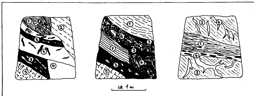
Abb. 6: Ortsbilder aus dem Bergbau Kelchalpe, nach Zeichnungen von W. OPPEL (1883), östl. Feldort; 1 = Schwarzer Tonschiefer, 2 = Grauer Hangendschiefer, 3 = Kupferkiesderberz, 4 = Gangquarz mit Erznestern, 5 = Grauer Liegendtonschiefer mit Quarzlinsen und Kupferkies, 7 = Grauer Tonschiefer.
