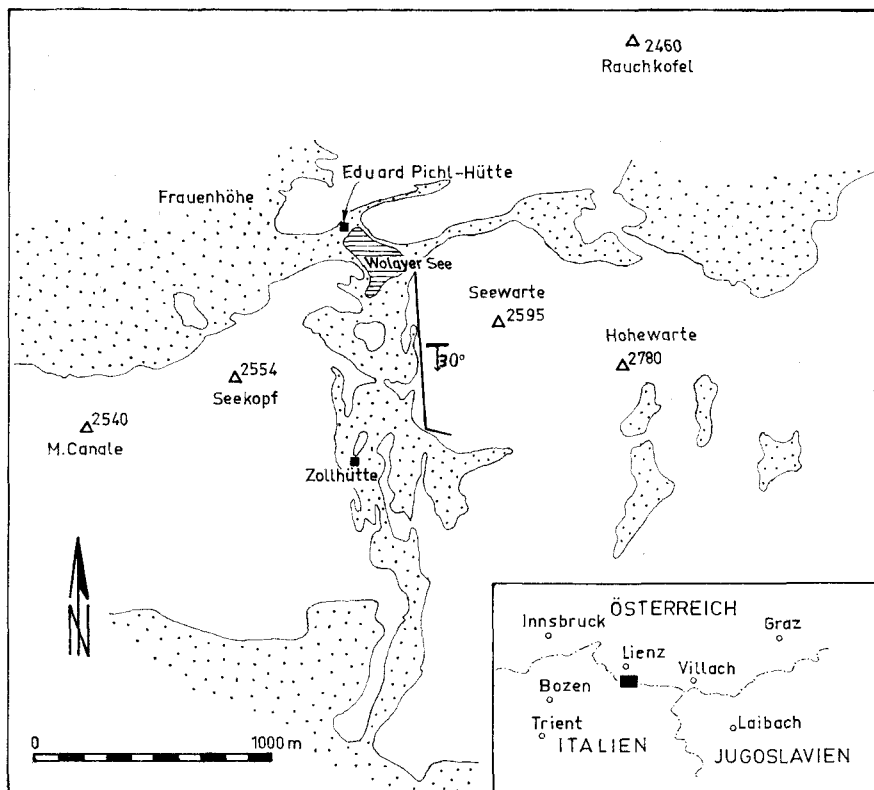
Abb. 1. Übersichtskarte; weiß = anstehendes Gestein, punktiert = Halde
