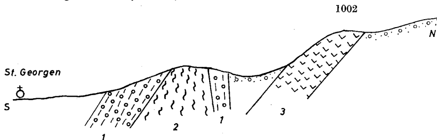
Abb. 3 1 Quarzit, 2 Serizit-Chloritquarzphyllit, 3 Prasinit
