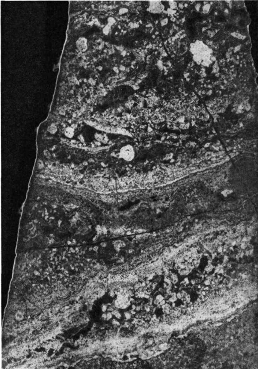
Abb. 3: Stromatolith, Wettersteinkalk; mm -rhythmische Wechsellagerung von dolomitischen Feinschichten (Algenmatten) und aufgearbeitetem Stromatolithmaterial; Dolomit weiß, Kalk grau. Fundort: Petzen N-Seite. Vergrößerung vierfach.
