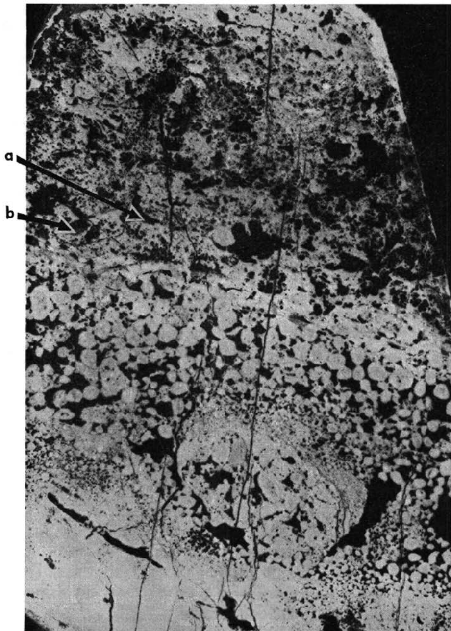
Abb. 7: Stromatolith, Wettersteinkalk; unterer Teil mit inverser Gradierung des aufgearbeiteten Algensedimentes, Übergang nach oben in Stromatolith mit laminaem Fenstergefüge Typ B; fossile Wasserwaagen (siehe Pfeile); Dolomit weiß, Calcit schwarz. Fundort: Petzen, Kolscha Berghaus. Vergrößerung vierfach.
