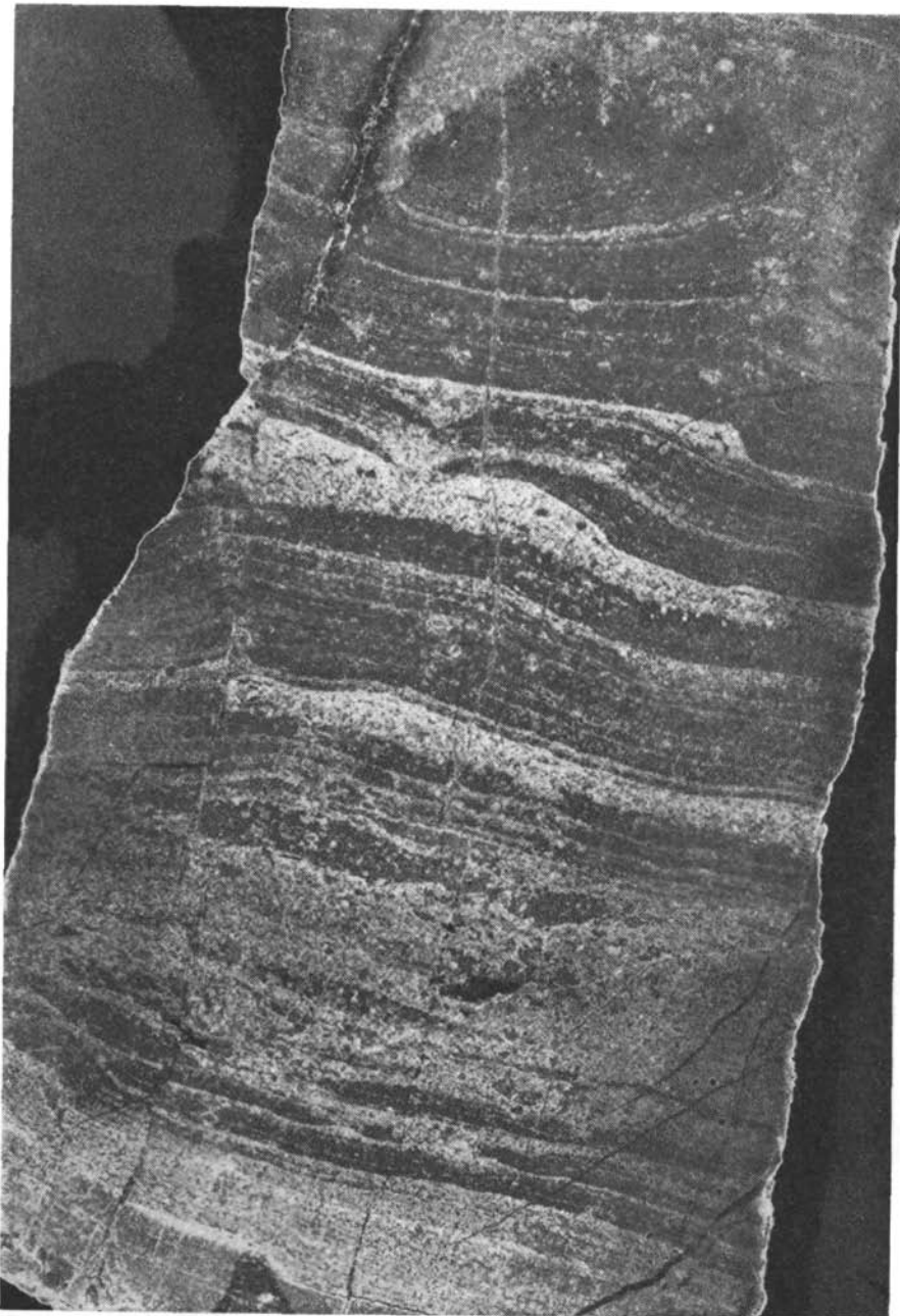
Abb. 2: Stromatolith, Wettersteinkalk; mm -Rhythmik, sehr feine Wechsellagerung von Kalk und Dolomit (Algenmatten); Dolomit weiß, Kalk grau. Fundort: Petzen N-Seite. Vergrößerung vierfach.
