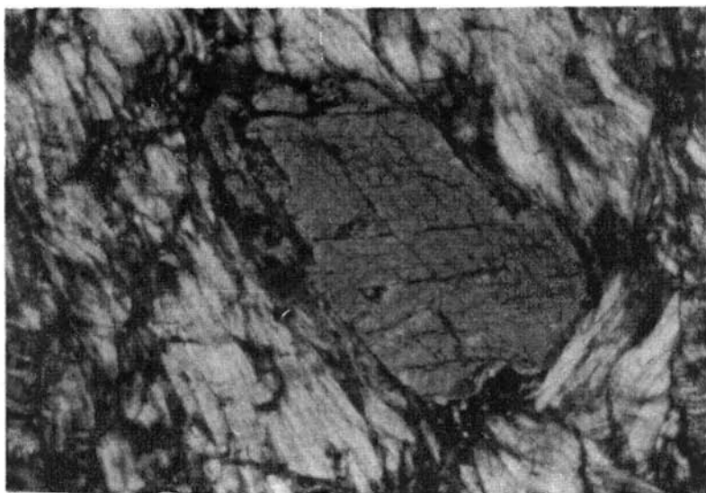
Abb. 12. In einem Gewebe aus retromorph gebildetem Chlorit liegt ein völlig unzerstört erhaltener Hornblende-xx. Amphibolit. X Nicols, Obj. NPL 6.3, Vergrößerung ca. 225fach.
