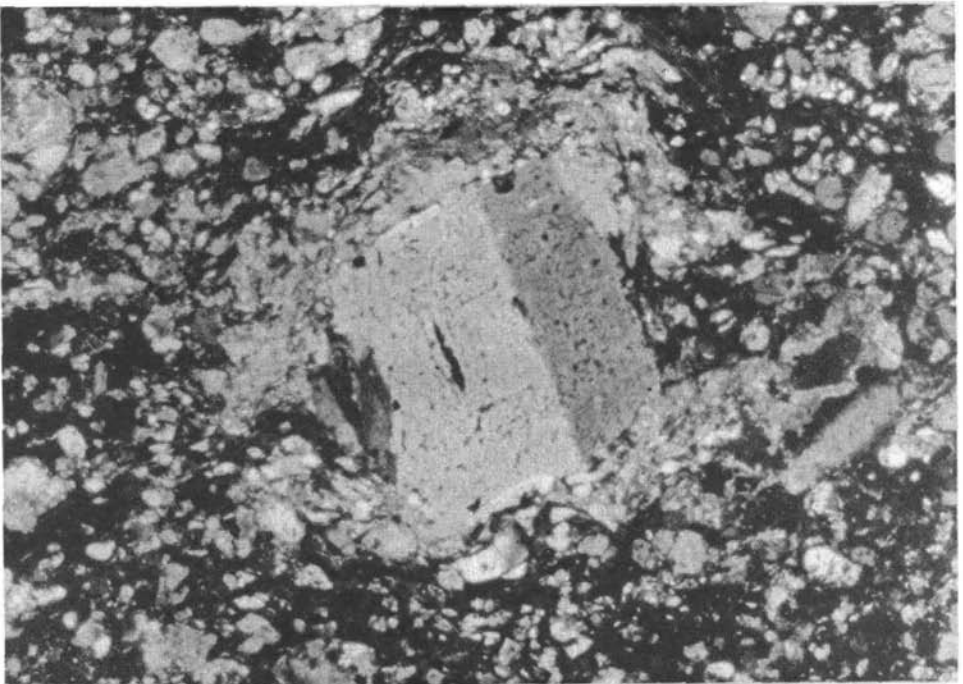
Abb. 5. Oligoklasauswürfling in einem Metakristalltuff. Durch die opaken, regelmäßig angeordneten Einschlüsse sind die Anwachszone rekonstruierbar. X Nicols, Obj. Pl 2.5, Vergrößerung ca. 90fach.
