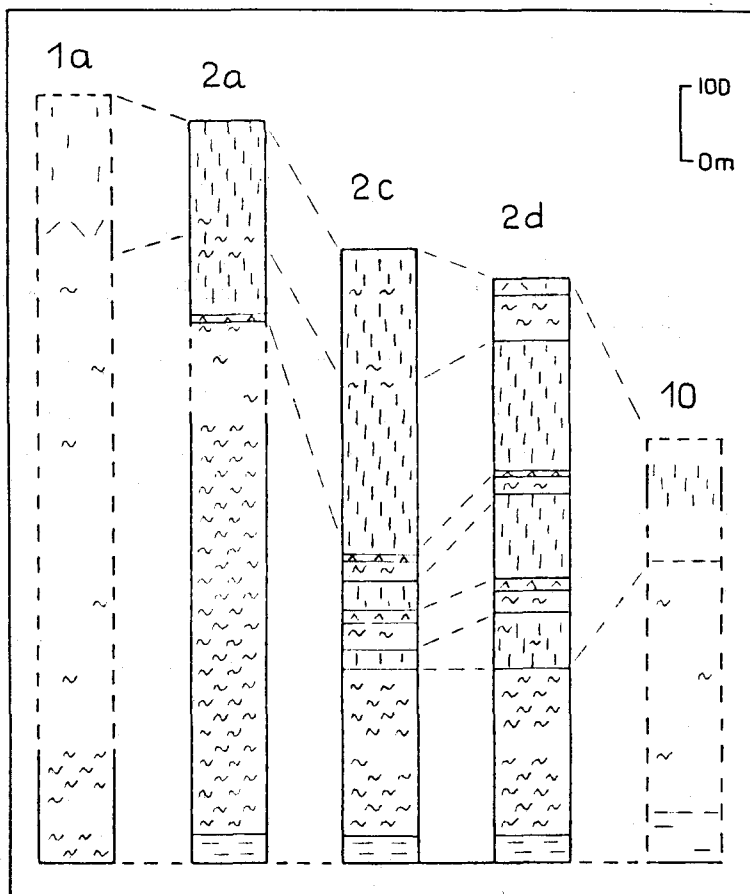
Abb. 18. Stark schematisierte Säulenprofile der Serie der „weißen Wand“. Maßstab 1 : 10.000. Legende wie bei Abb. 16.
