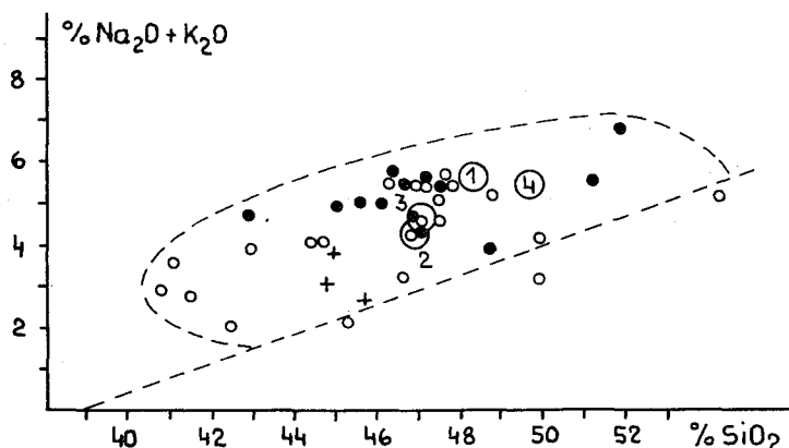
Abb. 2. Verhältnisdiagramm Gew.-% \text{Na}_2\text{O} + \text{K}_2\text{O} gegen \text{SiO}_2 , umgezeichnet nach LOESCHKE (1973). Analysen von drei Metabasiten aus dem Goldeckgebiet (Kreuzsignatur) im Vergleich mit Basalten und Spiliten anderer Lokalitäten.
