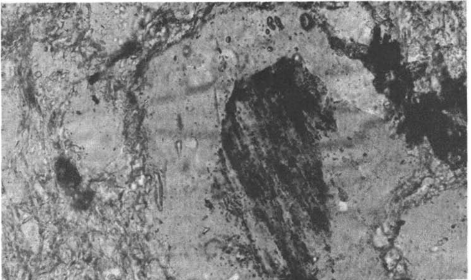
Abb. 6. Albitkorn in einem Metatuffit mit Sedimentvormacht. Der mit Opazit bestäubte Kern gibt die Umrisse des vulkanischen Plagioklases wieder, der einschlufsfreie Rand wird als Anwachsraum gedeutet. // Nicols, Obj. NPl 16, Vergrößerung ca. 580fach.
