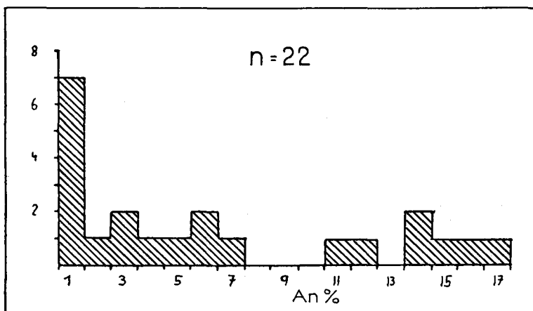
Abb. 14: An-Gehalte von 22 Plagioklasen aus den sauren Orthogneisen.
