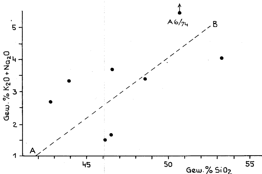
Abb. 9. Gew.-% Alkalioxide gegen Gew.-% SiO 2 , umgezeichnet nach CARMICHAEL et al. (1974). Trennungslinie zwischen Alkali-Basalten (oben) und tholeiitischen Basalten (unterhalb A—B) nach MACDONALD & KATSURA (1964) (referiert in CARMICHAEL et al., 1974). Punkte = Analysen von Hornblendegesteinen aus dem Goldeckgebiet.
