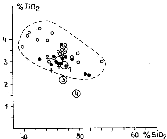
Abb. 3. Verhältnisdiagramm Gew.-% \text{TiO}_2 gegen Gew.-% \text{SiO}_2 , umgezeichnet nach LOESCHEKE (1973). Analysen von drei Metabasiten aus dem Goldeckgebiet (Kreuzsignatur) im Vergleich mit Basalten und Spiliten anderer Lokalitäten. Signaturen wie in Abb. 2.
