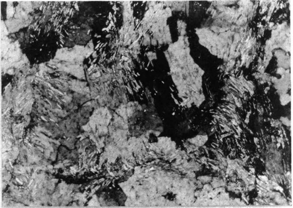
Abb. 7. Plagioklas und Quarz überwachsen Faltenzüge aus Hellglimmer in einem Zweiglimmerquarzit. X Nicols, Obj. NPl 6.3, Vergrößerung ca. 225fach.
