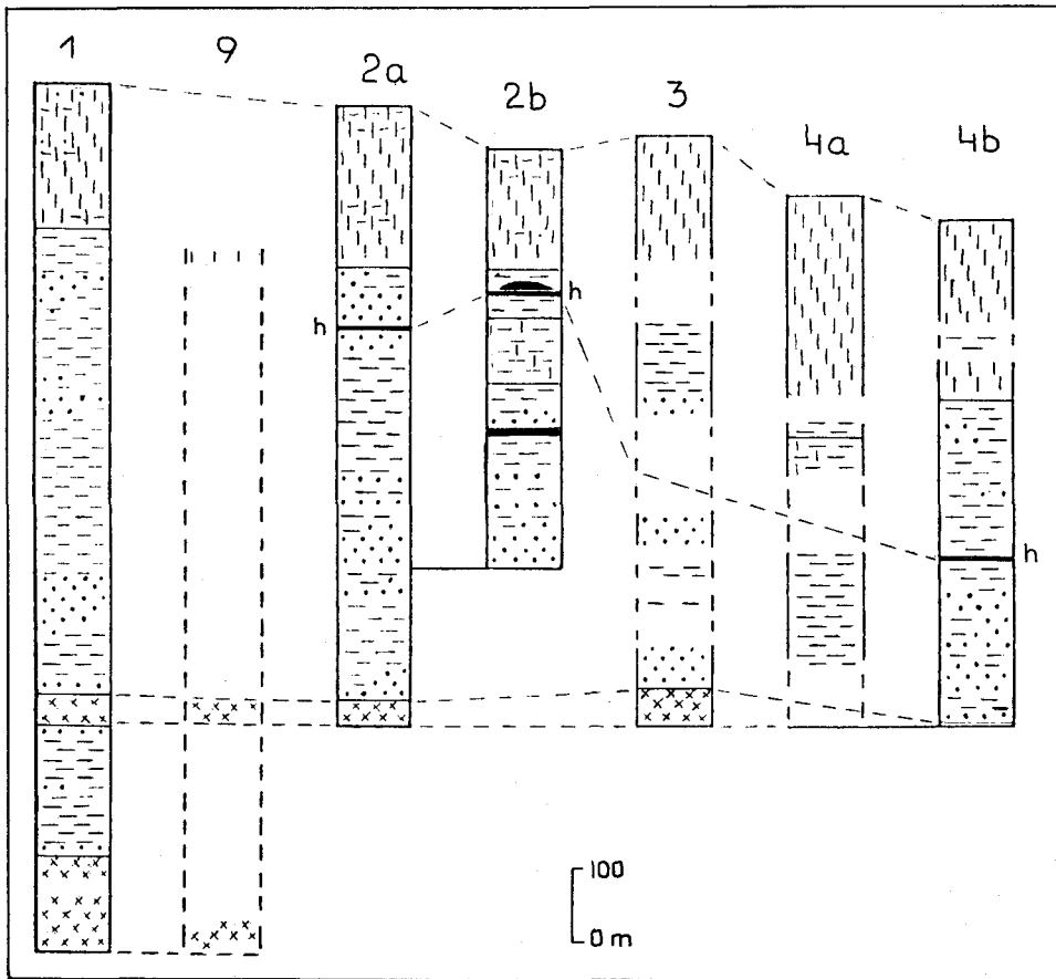
Abb. 17. Stark schematisierte Säulenprofile der Serie oberhalb der sauren Orthogneise. Maßstab ca. 1 : 10.000. Legende wie bei Abb. 16.
