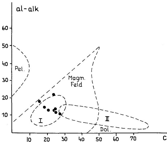
Abb. 10. NIGGLI-Werte (al—alk) gegen c, umgezeichnet nach WEBER-DIEFENBACH (1976). Die analysierten Hornblendegesteine des Goldeckgebietes (Punkte) liegen alle im magmatischen Feld. Bereich I = Orthoamphibolite, Bereich II = Paraamphibolite.
