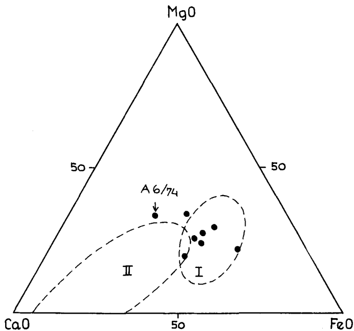
Abb. 11: Konzentrationsdreieck MgO—FeO (Gesamteisen)—CaO, umgezeichnet nach WEBER-DIEFENBACH (1976). Signaturen wie bei Abb. 10. Mit Ausnahme des Hornblendegarbenschiefers liegen alle Punkte im orthogenen Bereich.
