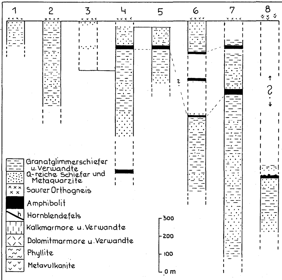
Abb. 16. Stark schematisierte Säulenprofile der Serie unterhalb der sauren Orthogneise. Maßstab ca. 1 : 10.000. 1 = Einödgraben, 1a = Nase oberhalb Einödgraben zur Kote 1830, 2 = Schreigraben, 2a = Schreigraben E-Ast, 2b = Schreigraben W-Ast, 2c = Schreigraben, 3. Ast von E, 2d = Schreigraben, 2. Ast von W, 3 = Raunachgraben E-Ast, 4 = Raunachgraben Hauptast, 4a = Raunachgraben Ast parallel Liftseil, 4b = Raunachgraben W-Ast, 5 = Weg von Schwaig zum Raunachgraben Höhe 1000 m, 6 = Graben vom Leitner über die Kote 957 zur Schwaiger Alm, 7 = Unterhauser Bach, 8 = Baldramsdorfer Bach, 9 = Fahrweg zur Bergerhütt., 10 = Nase vom Matzenkofel in Richtung Goldeckhütt.
