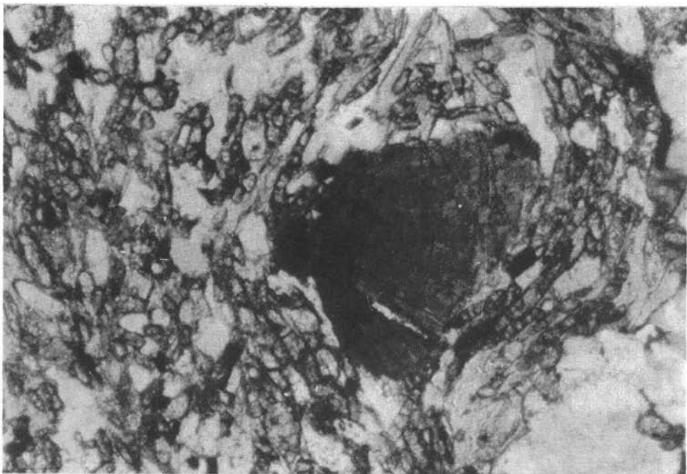
Abb. 4. Turmalinsonne in einem feinkörnigen Metaaschentuffit. // Nicols, Obj. NPL 6.3, Vergrößerung ca. 225fach.
