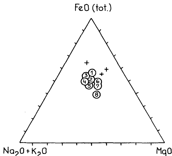
Abb. 1. AFM-Diagramm, umgezeichnet nach LOESCHKE (1973). Analysen von drei Metabasiten aus dem Goldeckgebiet (Kreuzsignatur) im Vergleich mit Basalten und Spiliten anderer Lokalitäten.
