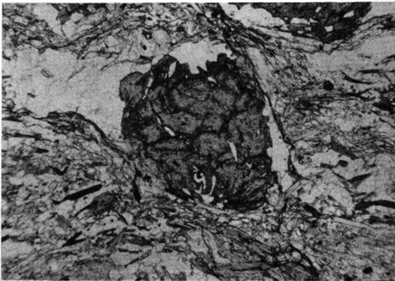
Abb. 4. Granat mit s-förmig gekrümmtem, verlegtem Internegefüge von Quarz und opaken Mineralen aus der Granatglimmerschieferserie. Vergrößerung ca. 120fach.
