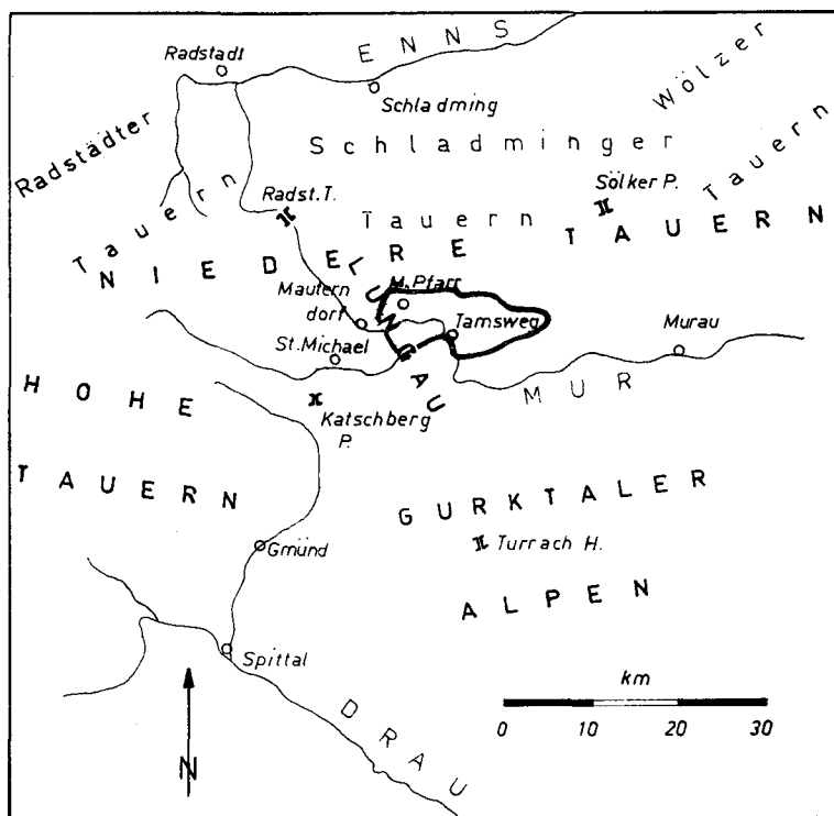
Abb. 1. Die Lage des Arbeitsgebietes und die Gebirgsumrahmung des Lungaus.
