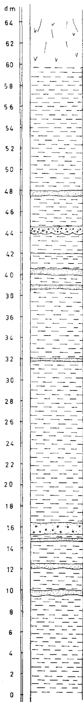
Abb. 11. Schematisiertes Profil durch die Schiefertone der alten Ziegelei Lintsching.
