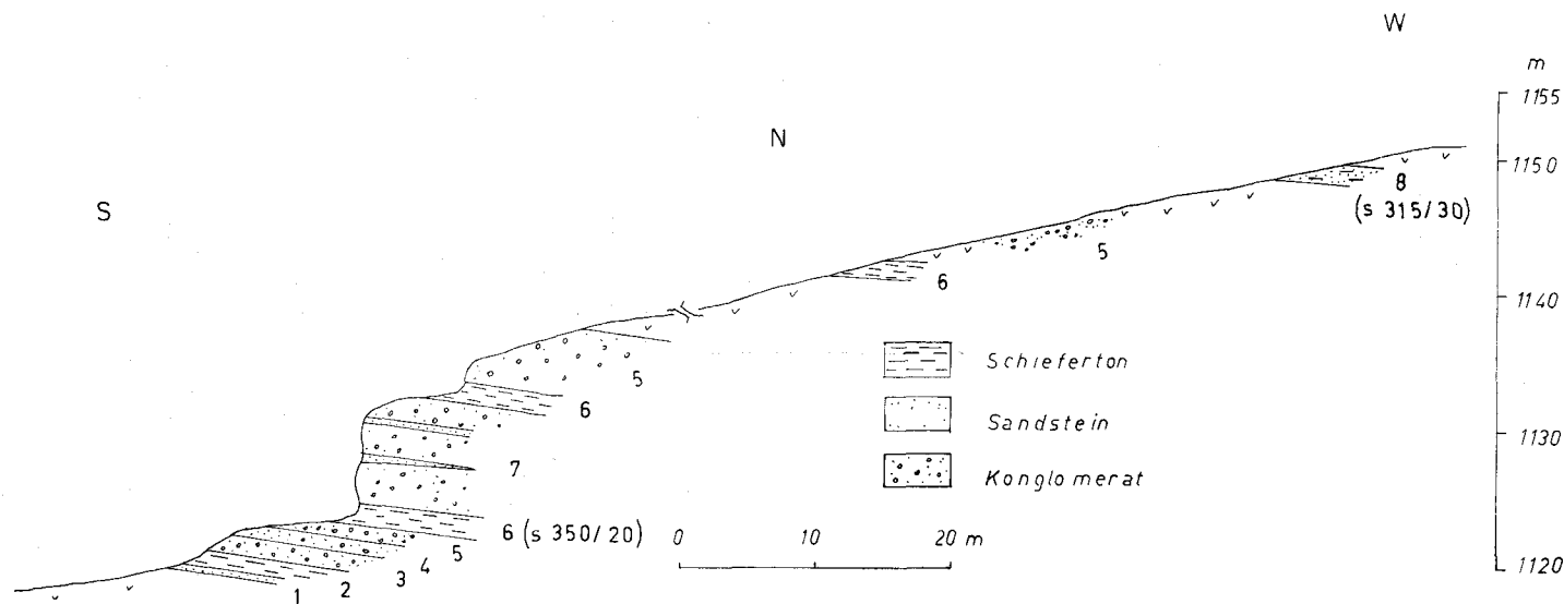
Abb. 10. Schematisierter geologischer Schnitt durch die Serie der Wechsellagerungen im Graben SW Dickbauer.
