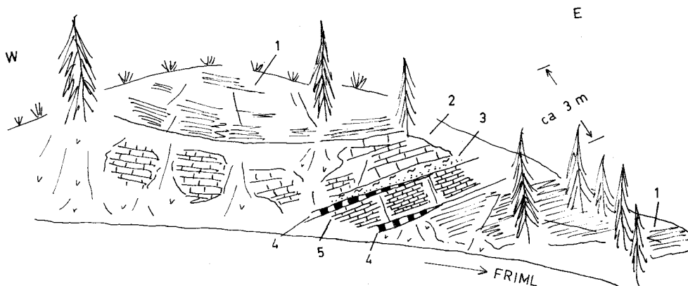
Abb. 3. Aufschlußskizze des Karbonatkomplexes an der Forststraße Unterberg-Pichl, ca. 150 m NW Frimlhof.
