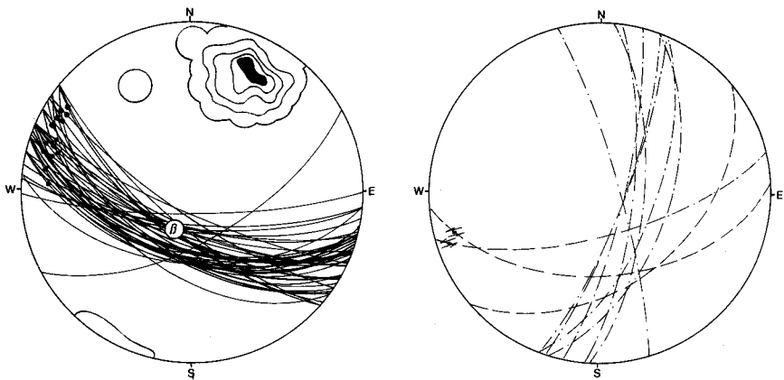
Abb. 8: Diagramm Rohr (links): s-Großkreise mit B-Fältelungsachsen, 42 Lotpunkte statistisch: 28-22-12-4-0%. Schwache Tautozonalität der s-Flächen: \beta -Achse
