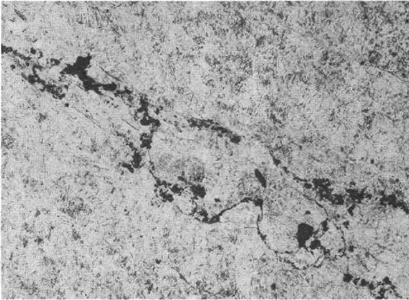
Abb. 18: Kies- und Goldanreicherung (schwarz) im s des Feinquarzits (verschieden grau). Dünnschliff, 1 Nic. Natürliche Größe 3,35 × 2,20 mm
