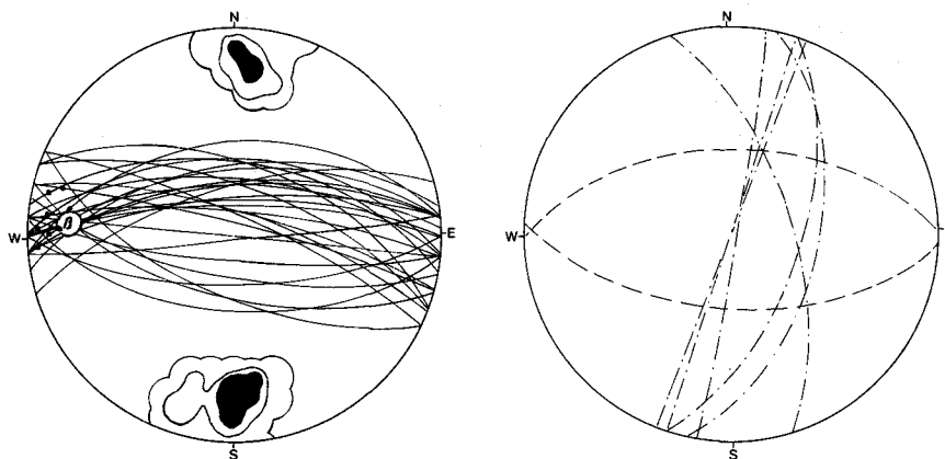
Abb. 10: Diagramm Laimach (links): s-Großkreise mit B-Fältelungsachsen, 29 Lotpunkte statistisch: 37-20-8-0%. B und \beta fallen zusammen
