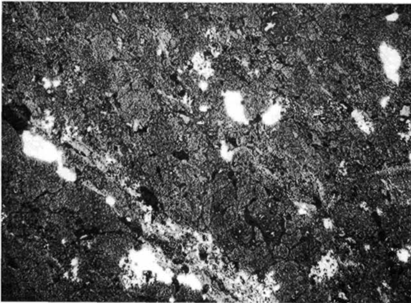
Abb. 21: Feinlagig-inhomogene Verteilung von ged. Gold (weiß) mit Fe- und As-Kieseln (weißgrau) in Quarzit (schwarzgrau, rauh). Goldquarzit, Pol. Anschliff, Nic.//. Natürliche Größe 1,28 \times 0,84 mm
