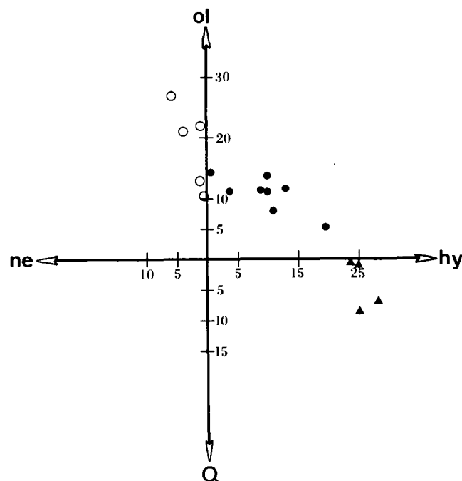
Abb. 8: Normgehalte der analysierten Amphibolite der Buntens Serie, der Monotonen Serie und der Gföhler Einheit (?). ● ol-hy-normativ; ○ ol-ne-normativ; ▲ hy-qu-normativ. Keine Gliederung nach Serien möglich.
