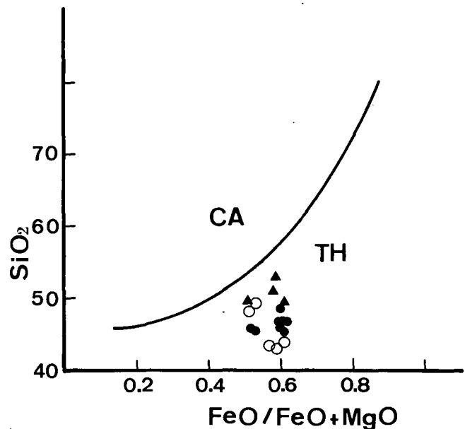
Abb. 10: Korrelationsdiagramm \text{SiO}_2 gegen \text{Fe}/(\text{FeO}+\text{MgO}) . Die Kurve zeigt die Grenze zwischen Tholeiiten und Kalkalkibasalten nach MIYASHIRO (1974). Symbole wie Abb. 8.
