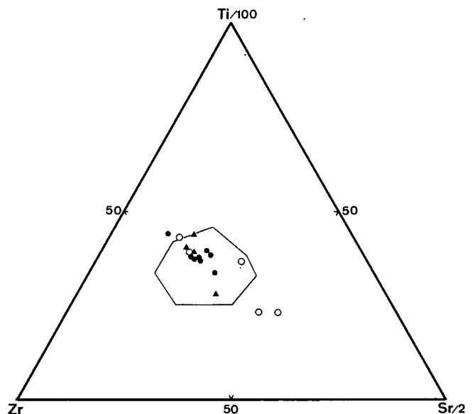
Abb. 13: Diagramm Ti/100-Zr-Sr/2 nach PEARCE & CANN (1973). Symbole wie Abb. 8.
