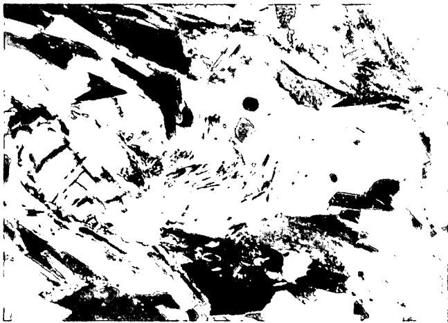
Abb. 4: Cordieritgneis der Monotonen Serie. Cordierit umschließt Biotit und Sillimanit. Beide eingeschlossenen Minerale sind räumlich voneinander getrennt und weisen auf die Reaktion \text{Bio} + \text{Sill} + \text{Qu} = \text{Cord} + \text{Alk} + \text{H}_2\text{O} hin. Nicols gekreuzt, Vergr. ca. 75x.
