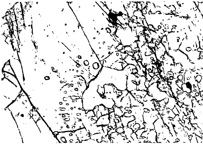
Abb. 1: Teil eines Granats aus einem Granat-Biotit-Sillimanit-Alkalifeldspatgneis der Bunten Serie. Der Zentralteil ist voll von Einschlüssen, der Rand frei davon. Durchlicht, Vergr. ca. 45x.
