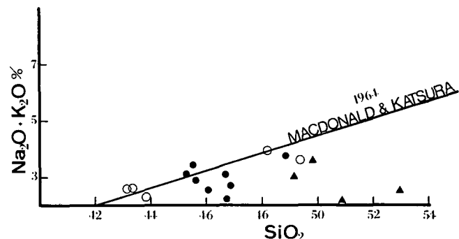
Abb. 9: Korrelationsdiagramm \text{Na}_2\text{O} + \text{K}_2\text{O} gegen \text{SiO}_2 . Die Linie zeigt die Grenze zwischen den tholeiitischen und alkali basaltischen Gesteinen nach MACDONALD & KATSURA (1964). Symbole wie Abb. 8.
