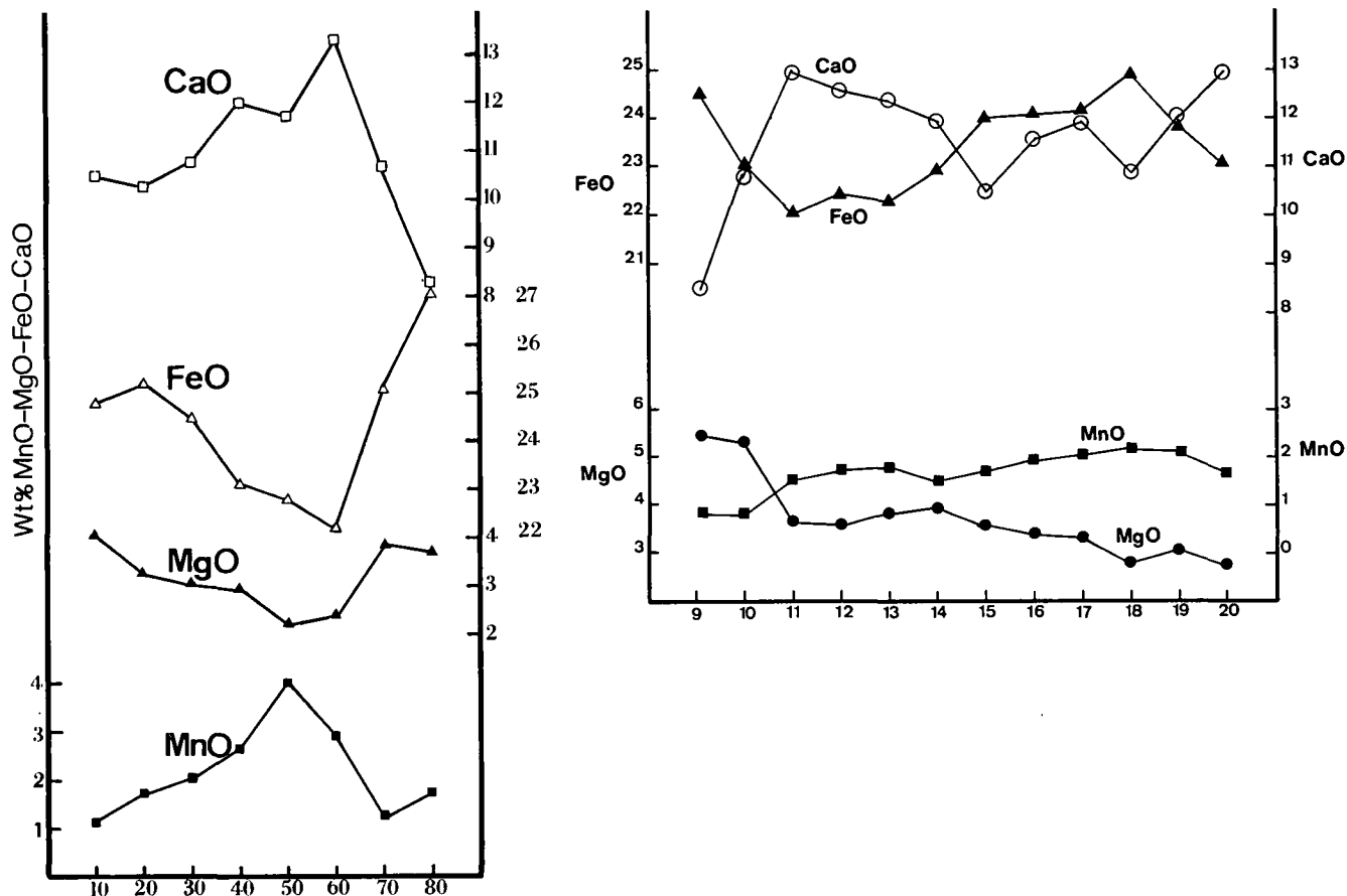
Abb. 15: Granatprofile aus den Amphibolitproben L-3 und P-12. Der Granat der Probe L-3 ist einphasig durch Elementfraktionierung gewachsen, jener der Probe P-12 durch mindestens zweiphasiges Wachstum.
