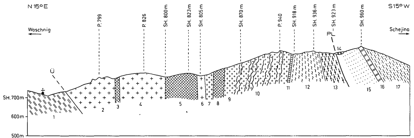
Abb. 1: Profil längs des wasserscheidenden Bergkammes zwischen Vellach und Ebriachbach. PL = Hauptstörung des Periadriatischen Lineamentes; Erläuterung der Signaturen im Text!
