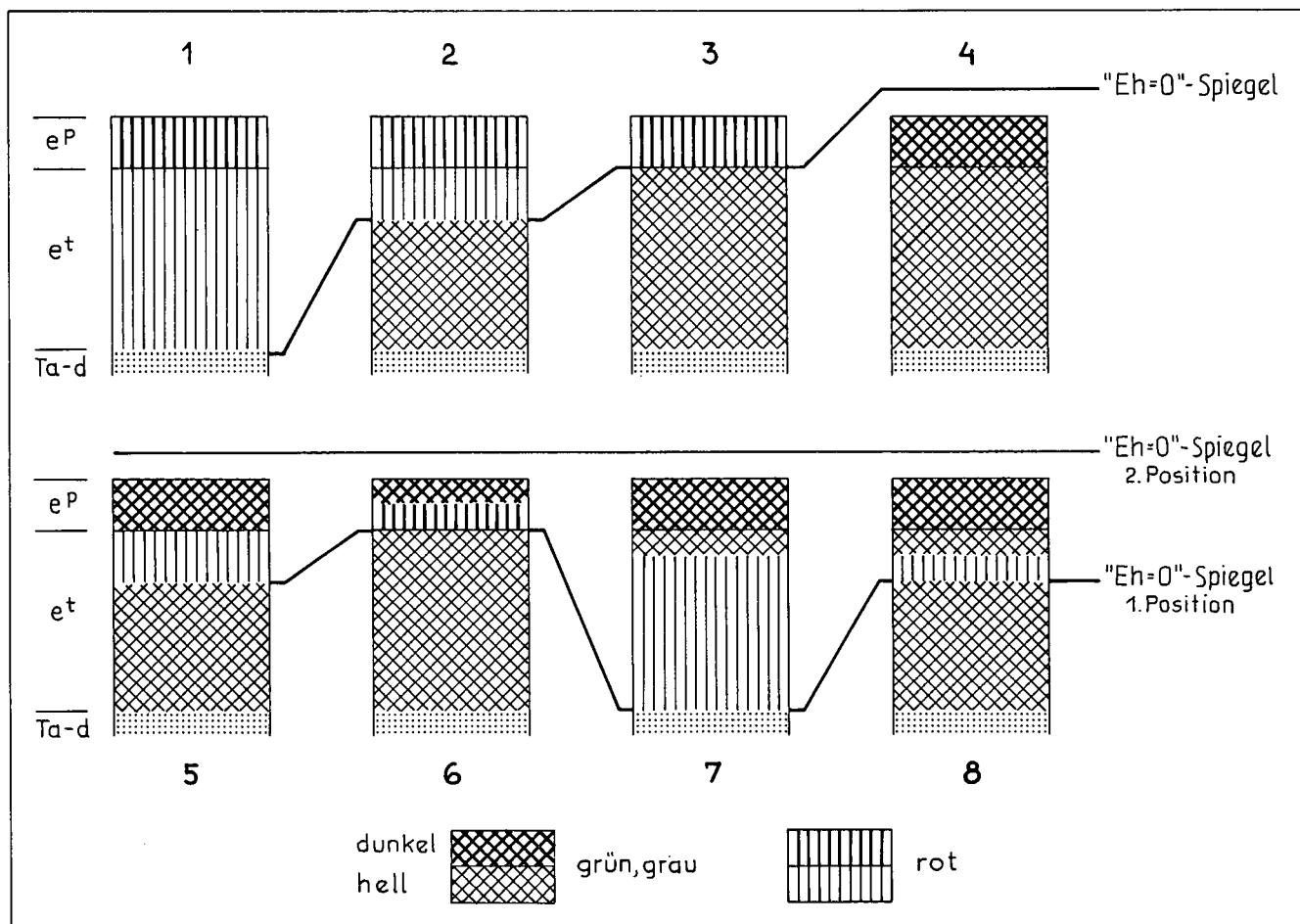
Abb. 13: Schematische Darstellung der Farbabfolgen in den Peliten der Brunnbachschichten. et turbiditischer Pelit (Mergel mit durchschnittlich 40 Gew% CaCO 3 ); eP hemipelagischer Pelit (Tonstein mit durchschnittlich 4 Gew% CaCO 3 ). Vgl. FAUPL & SAUER, 1978.
