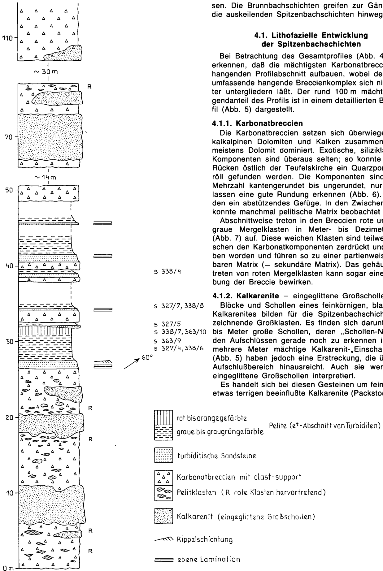
Abb. 5: Detailliertes Bankprofil aus dem liegenden Profilabschnitt der Spitzbachschichten. Spitzbachklamm westlich von St. Gallen.
