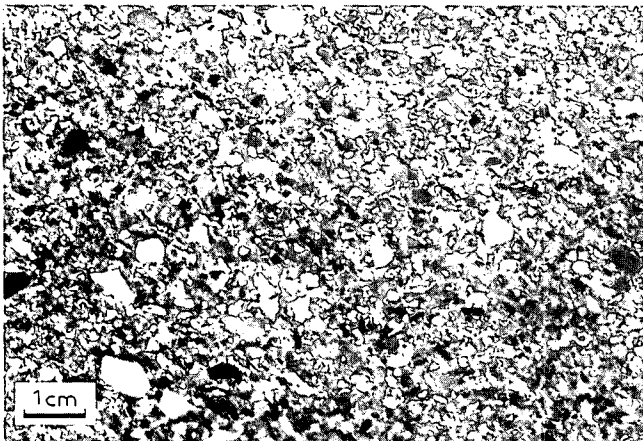
Abb. 17: Polymikte Zusammensetzung der feinbrecciösen Basis einer Turbiditbank aus den Brunnbachschichten (sandstein- und breccienreiche Turbiditfolge). Anschnitt parallel zur Schichtung. Maßstab 1 cm.
