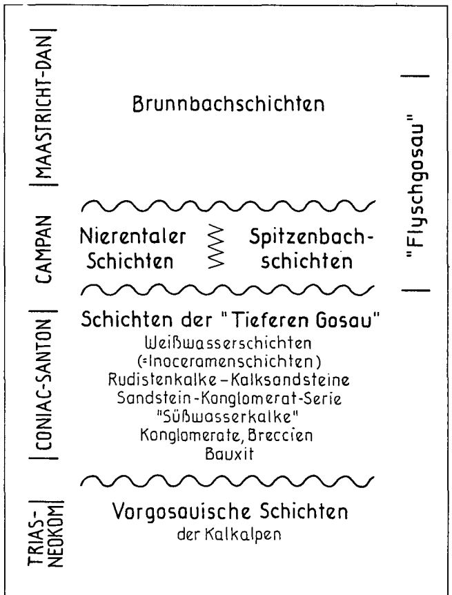
Abb. 2: Die Gliederung der Gosauablagerungen im Gebiet der Weyerer Bögen.
