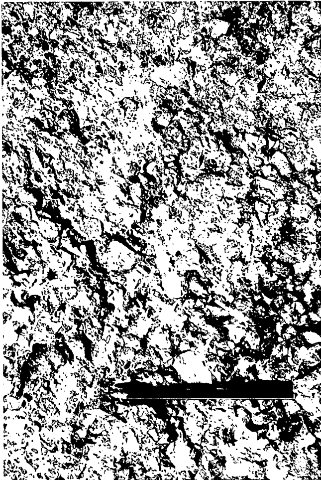
Abb. 6: Karbonatbreccie der Spitzenbachschichten. a) Aufschluß (Maßstab ca. 15 cm) b) Anschliff (Maßstab 1 cm). Spitzenbachklamm.
