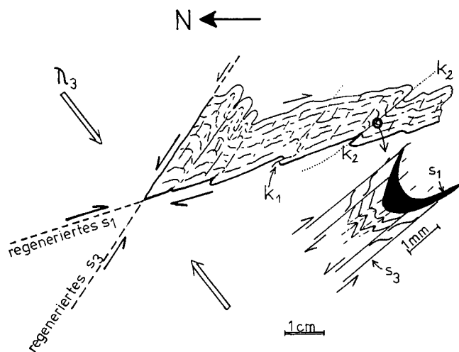
Abb. 7: Plattungsgefüge der 4. Deformationsphase im Handstückprofil (Probe 14). Der Entnahmeort der Probe ist in Abb. 8 mit -I- markiert (Feldspat-Quarz-Glimmerschiefer in der Nähe der Frauenwand).
