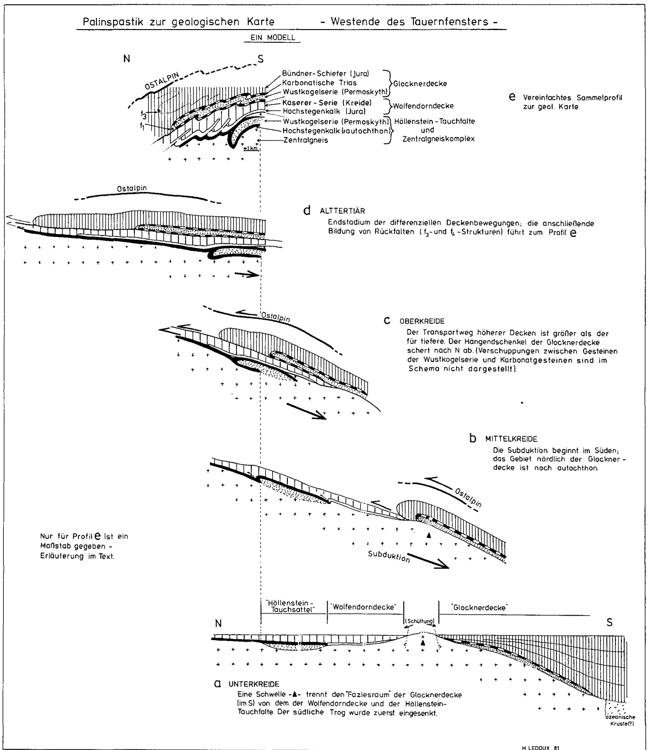
Abb. 4: Palinspastische Profile.
