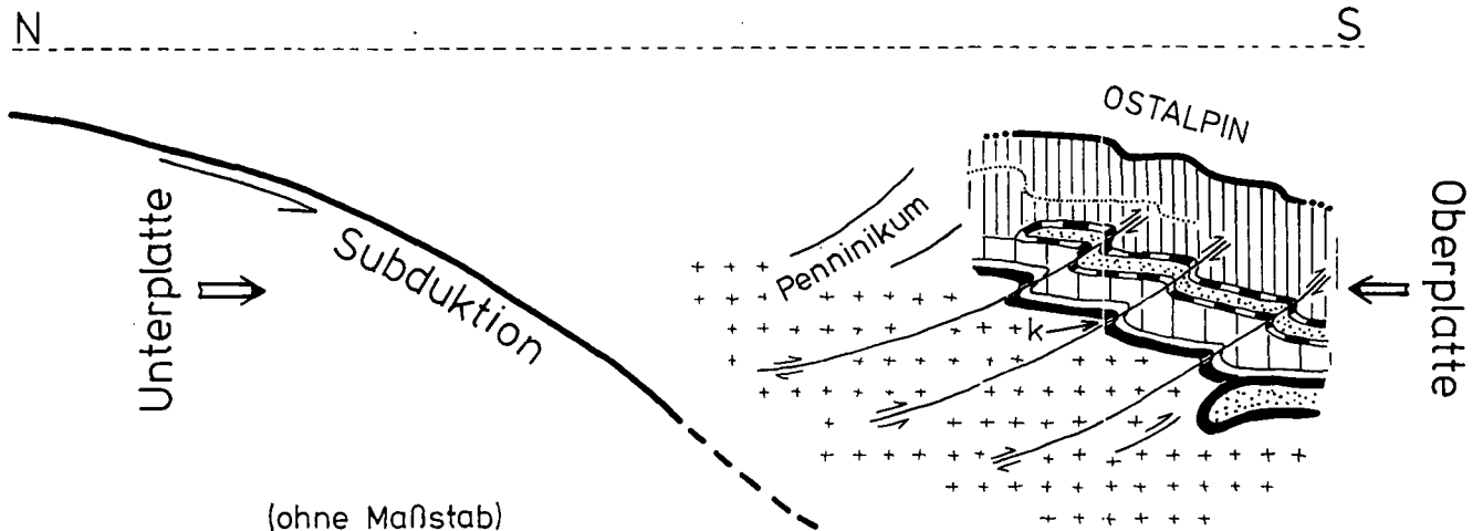
Abb. 6: Modell zur Deutung der südvergenten f_3 -Faltung; das Schema zeigt das Sammelprofil der Abb. 4 e in einem Stadium während der 3. Deformationsphase; Legende der Gesteinseinheiten siehe Abb. 4 e; bei –k– liegt die „zukünftige“ Frauenwand (vgl. Abb. 2).
