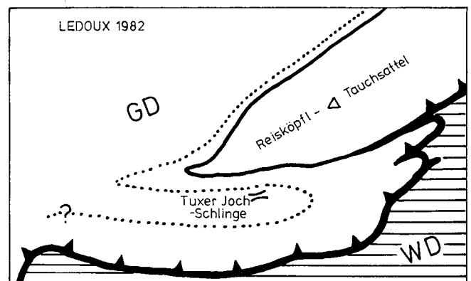
Abb. 5 (a–c): Die geologischen Verhältnisse am Tuxer Joch; schematischer Kartenausschnitt aus Abb. 1 mit verschiedenen Deutungen; GD = Glocknerdecke („Obere Schieferhülle“), WD = Wolfendorndecke („Parautochthone Schieferhülle“, Teil der „Venedigerdecke“), Punktreihe: Metabasalte und deren klastische Begleitserie.
