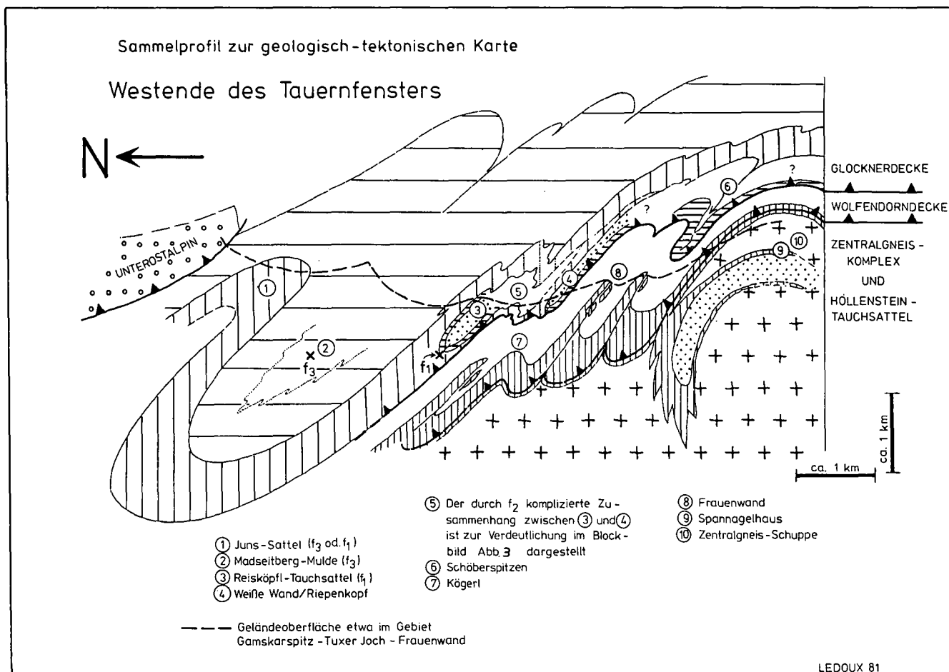
Abb. 2: Schematisches Sammelprofil zur geologischen Übersichtskarte; Legende siehe Abb. 1.
