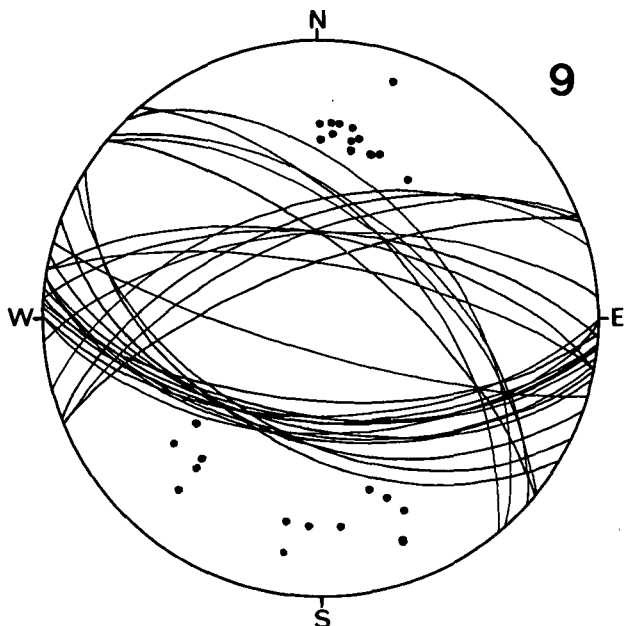
Diagramm 9: Badstuben. Wettersteinkalk und -dolomit, Hauptdolomit. (N- und S-Flügel). 26 s-Flächen. Im Hauptdolomit \beta = W-E, 10^\circ W ; mit Wettersteinkalk \beta = 116^\circ 25^\circ ESE .
