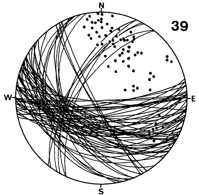
Diagramm 39: Golbitschgraben, Kreuzenbach. Alpinen Muschelkalk, Partnachkalk. 70 s-Flächen. \beta = 240^{\circ}45'WSW .
