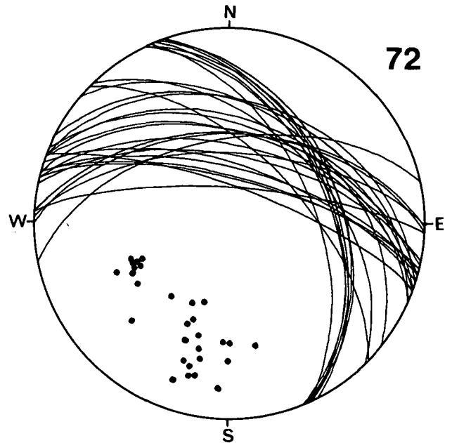
Diagramm 72: Dobratsch-SW, nördl. Lärchgraben. Alpiner Muschelkalk. 29 s-Flächen. W-Abschnitt \beta = 24°40'NE. Ges.- \beta = 58°45'NE.
