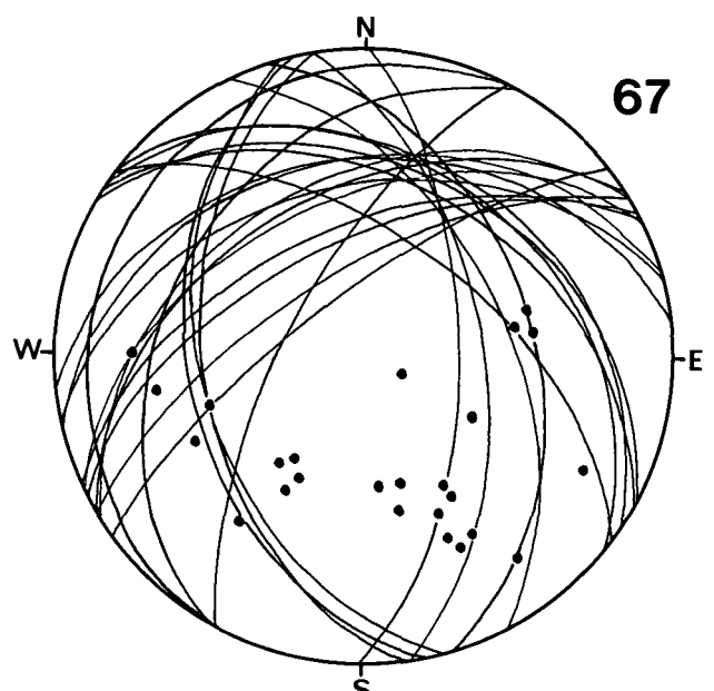
Diagramm 67: Dobratsch-S: Storfhöhe, Pungart-E, Oberfederaun. Wettersteinriffkalk. 25 s-Flächen. \beta = 24^\circ 20' \text{NNE} .
