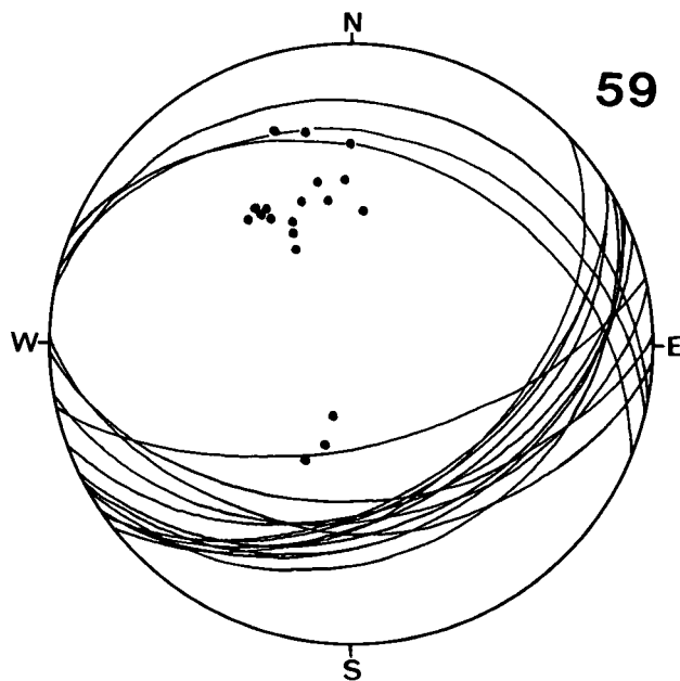
Diagramm 59: Schloßberg. Muschelkalk, Wettersteindolomit und -kalk. 19 s-Flächen, \beta = 84^\circ 14' \text{E} .
