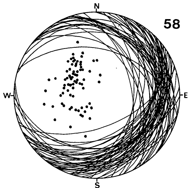
Diagramm 58: Schloßberg-S, -W, -N. Werfener Schichten, Alpiner Muschelkalk, Wettersteindolomit. 76 s-Flächen. \beta = 50^\circ 20' \text{NE} ; \beta = 68^\circ 20' \text{NE} , B lokal = 80^\circ 5' \text{E} . B = 88^\circ 27' \text{E} . Ges.- \beta = \text{W-E} , 28^\circ \text{E} .
