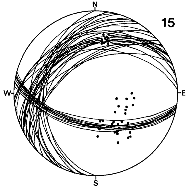
Diagramm 15: Bleibberger Graben-Ost, Kadutschen. Hauptdolomit. 41 s-Flächen. \beta = 262^\circ 25' W .
