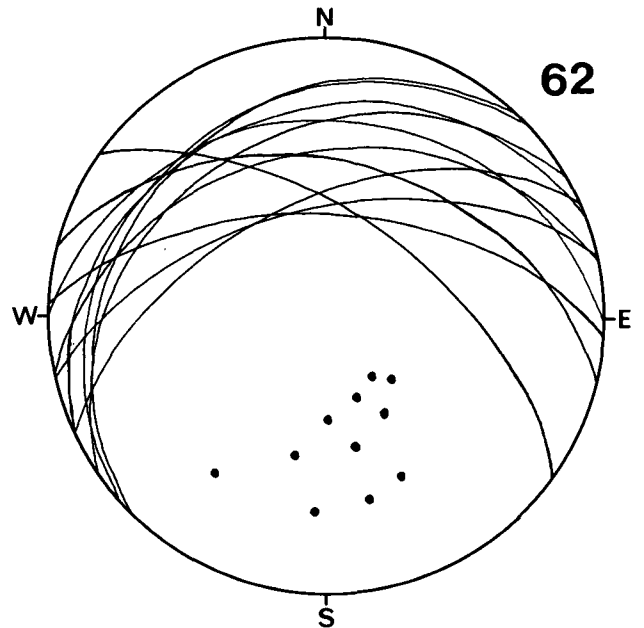
Diagramm 62: Aloisihütte-NW. Wettersteinschichten, Raibler Schichten. 11 s-Flächen. \beta = 89^{\circ}10'E , \beta = 286^{\circ}20'WNW bis 315^{\circ}30'NW gestreut.
