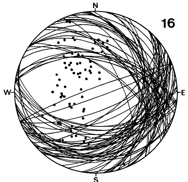
Diagramm 16: Bleibberger Graben-Ost, N und NE von Mittewald. Raibler Schichten, Hauptdolomit. 69 s-Flächen. \beta = 100-118^\circ 20'-25' ESE .
