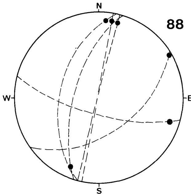
Diagramm 88: Heiligengeister Mulde. Raibler Schichten, Hauptdolomit. 6 Scherklüfte mit Striemung.
