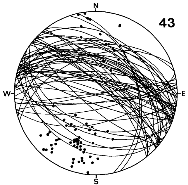
Diagramm 43: Kreuzen – Farchtnersee. Hauptdolomit. 65 s-Flächen. Einzel- \beta = 96^\circ 20'E ; \beta = 273^\circ 10'W ; \beta = 286^\circ 12'W ; \beta = 112^\circ 10'E ; \beta = 97^\circ 50'E ; \beta = W-E, 35^\circ E ; Ges.- \beta = W-E \text{ bis } WNW-ESE, E\text{-Fallen} .
