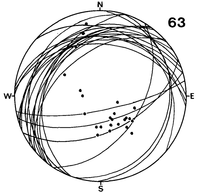
Diagramm 63: Aloisihütte. Raibler Schichten. 24 s-Flächen. Einzel- \beta = 62^{\circ}15'NE , \beta = 246^{\circ}16'WSW , \beta = 321^{\circ}31'NW ; Ges.- \beta = 40^{\circ}10'NE .
