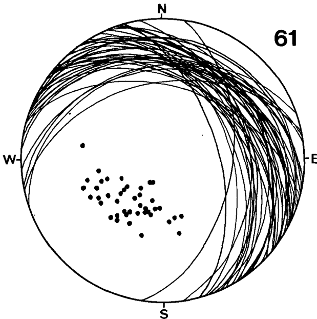
Diagramm 61: Rupagraben-E, Kanzel-Sockel. Grödener Schichten, Alpiner Muschelkalk, Wettersteinschichten. 42 s-Flächen. \beta = 16^{\circ}32'N bis 37^{\circ}30'N gestreut.
