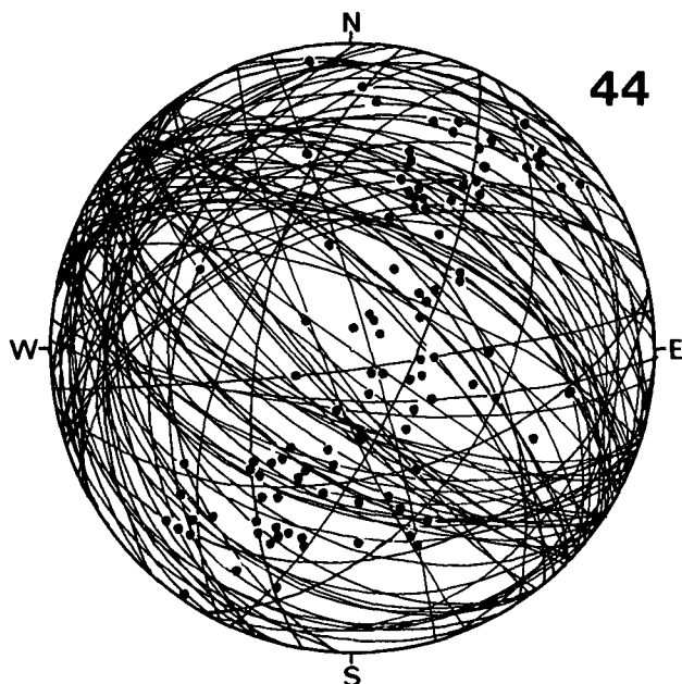
Diagramm 44: Altes Bergbaurevier Kienleiten. Wettersteinkalk, Raibler Schichten, Hauptdolomit. 104 s-Flächen. \beta = 310^\circ 10' - 20^\circ \text{NW} .
