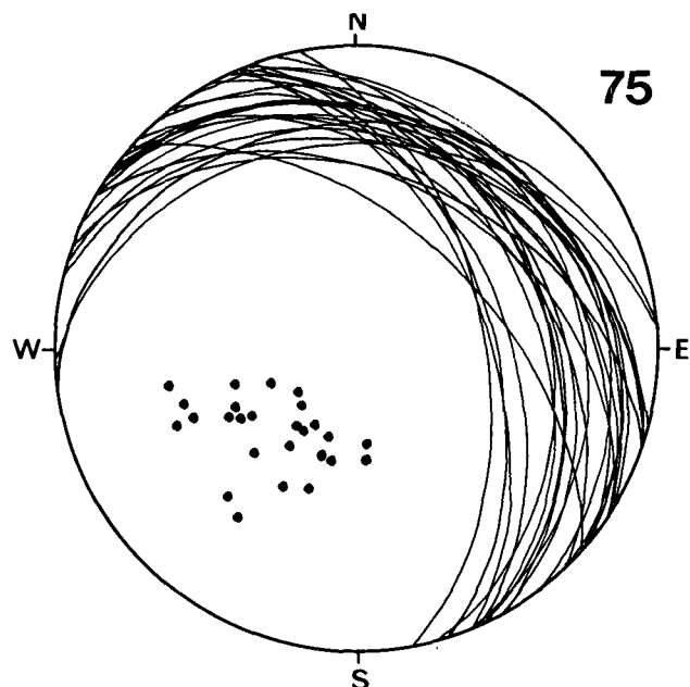
Diagramm 75: Dobratsch: Roßtratte, Zwölfernock-S, Höhenrain. Wettersteinriffkalk. 26 s, \beta = 14^\circ 30' \text{NNE} .
