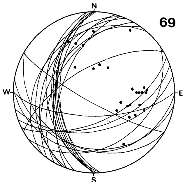
Diagramm 69: Graschlitzen. Wettersteinriffkalk. 24 s-Flächen. \beta = 230^\circ 25' SW .
