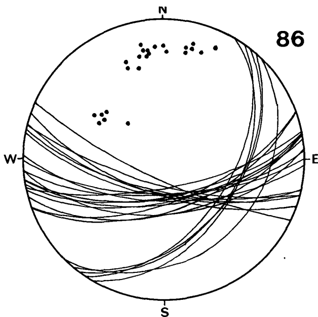
Diagramm 86: Steinbruch Heiligengeist, Mittewald, Obere Fellach. Raibler Schichten. 24 s-Flächen. \beta = \text{ca. } 123^\circ 50' \text{SE} .
