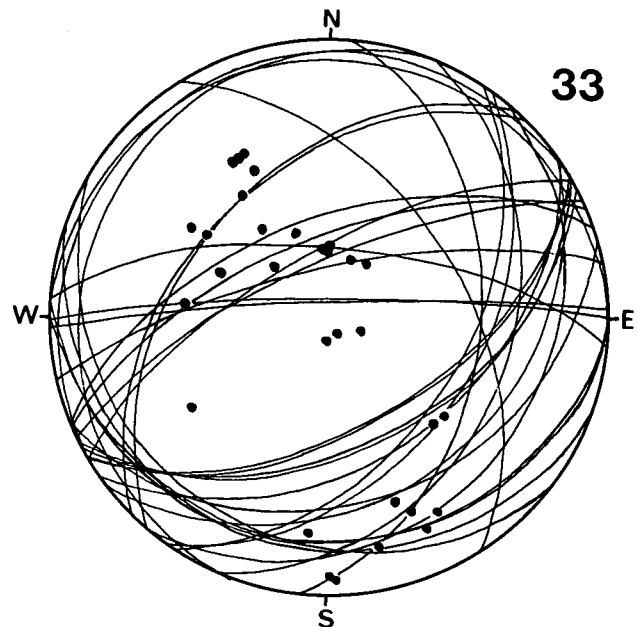
Diagramm 33: Brückelgraben. Alpiner Muschelkalk, Wettersteinkalk. 31 s-Flächen. \beta = B (MK) = W–E, 38^{\circ} W; \beta (WK) = 60^{\circ} , \pm horizontal.
