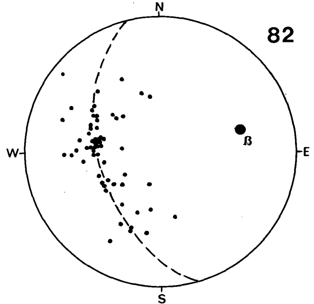
Diagramm 82: Dobratschmassiv: Bleiberger Scharte, Freywald. Wettersteinkalk. 59 s-Flächen. \beta = 75^\circ 38' ENE (Daten Geol. Abt. BBU).
