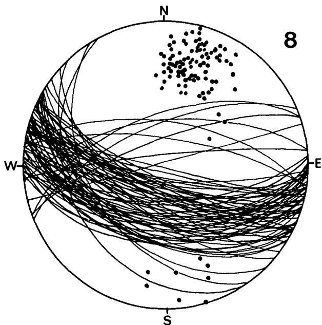
Diagramm 8: Windisches Alpi-Badstuben (mit S-Flügel der Synklinale). Raibler Schichten, Hauptdolomit. 97 s-Flächen. \beta = W-E, 30^\circ W ; \beta = W-E, 20-30^\circ W .
