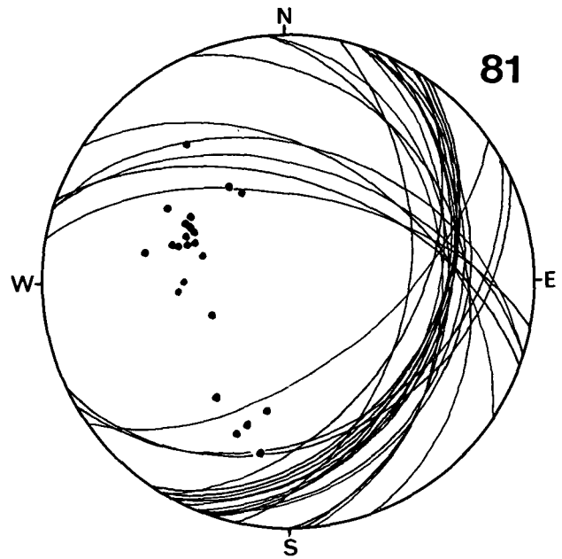
Diagramm 81: Dobratschmassiv: Schlepplift-Mittelstation (Jäger-rast), Freywald. Wettersteinkalk. 23 s-Flächen. \beta = 80^\circ 33' E .
