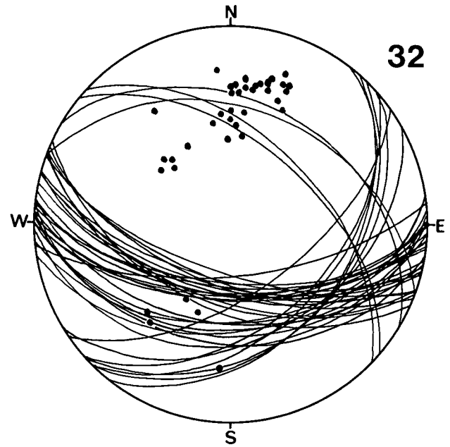
Diagramm 32: Erzberg-Ost: Spitzeck-Nord. Wettersteinkalk und -dolomit. 38 s-Flächen. \beta = 115^{\circ}20' - 40^{\circ} ESE.
