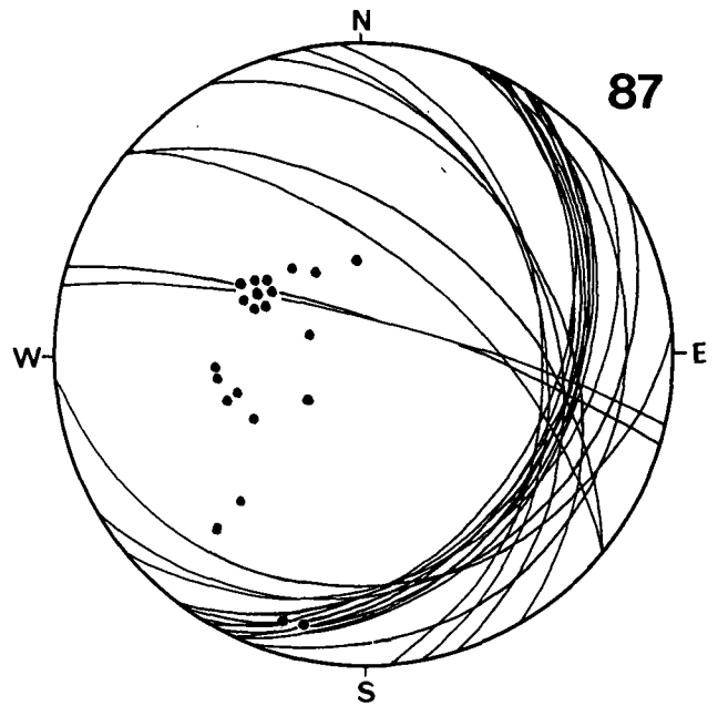
Diagramm 87: Heiligengeister Mulde, Fellachgraben, Pogöriach. Hauptdolomit. 22 s-Flächen. Einzel- \beta = 121^\circ 15' \text{ESE} ; Teufelsgraben: \beta = 120^\circ 20' \text{ESE} . Ges.- \beta = 104^\circ 30' \text{ESE} .
