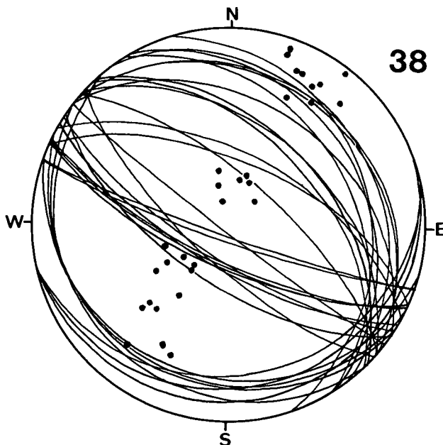
Diagramm 38: Kellerberg NW-Flanke. Alpinen Muschelkalk, Partnachkalk, Wettersteinkalk. 30 s-Flächen. \beta = 117^{\circ}10'ESE ; \beta = 124^{\circ}10'ESE ; \beta = 124^{\circ}18'ESE ; allg. \beta = 117^{\circ}10'ESE .
