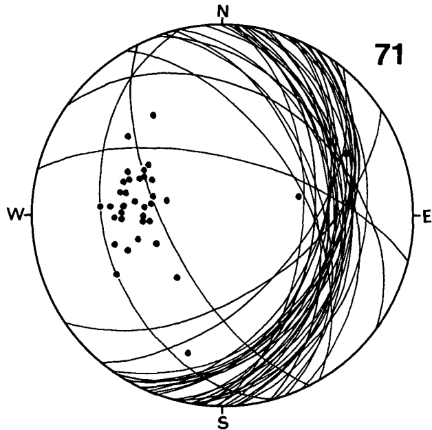
Diagramm 71: Kilzerberg-N, -E, -W. Alpiner Muschelkalk, Wettersteinschichtdolomit. 35 s-Flächen. Einzel- \beta = 326°13'NW. Ges.- \beta = ca. 84°36'E.
