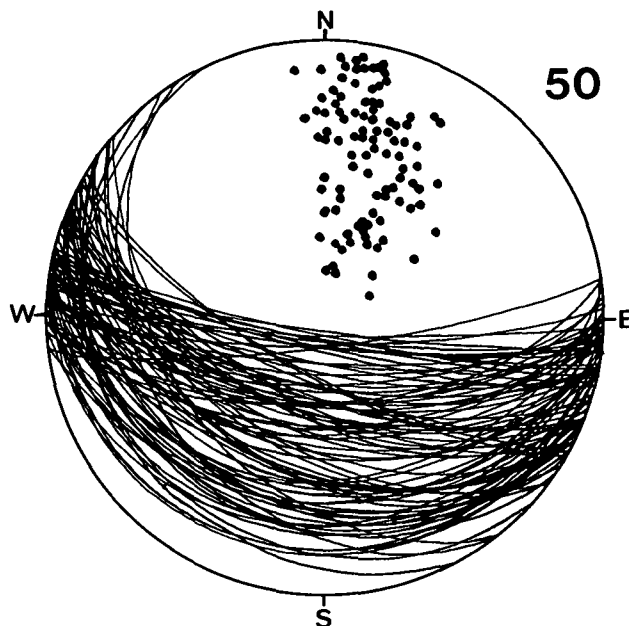
Diagramm 50: Einsiedler, Kellerberg, Auer. Alpiner Muschelkalk, Partnachkalk. 100 s-Flächen. Einsiedler: \beta = \text{W-E, } 30^\circ \text{W} ; Ges.- \beta = 276^\circ 10' \text{W} .
