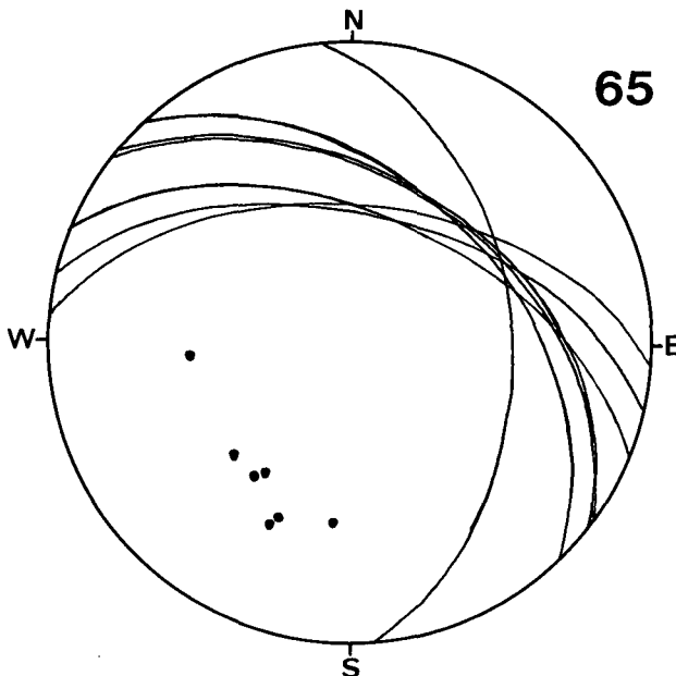
Diagramm 65: Dobratsch-S: Waben, Pungart-W. Alpiner Muschelkalk, Wettersteinriffkalk. 7 s-Flächen. \beta = 60^\circ 41' \text{NE} .
