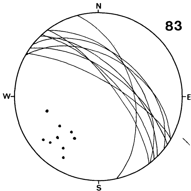
Diagramm 83: Hundsmaierhof, Brochiner, Goritschach, Villacher Sprungschanze. Wettersteinlagunenkalk. 9 s-Flächen.
