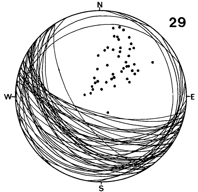
Diagramm 29: Erzberg-Nord: Sattlernock – Sonnblick – Mittagssnock – Hachelnock (ca. Kakstörung bis Kreuzenstörung). Wettersteindolomit. 45 s-Flächen. \beta = 280^\circ 10' W .
