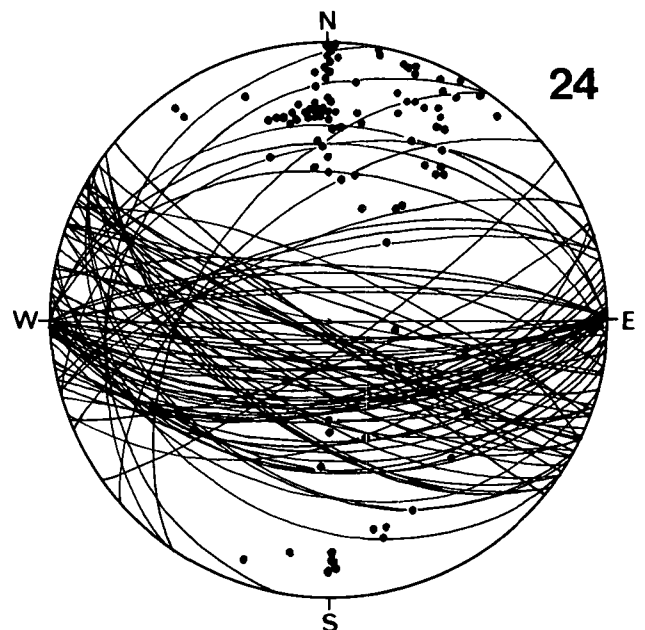
Diagramm 24: Rublandstollen: km 2.3 bis km 0.5. Nördlich Grenzkluft. Rubland-Einheit. Oberer Wettersteinkalk, Raibler Schichten, Hauptdolomit (Synklinale). 99 s-Flächen \beta = W-E, horizontal. \beta = ca. 290^{\circ}20' - 30^{\circ}WNW .
