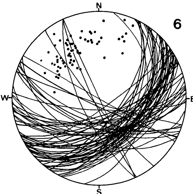
Diagramm 6: Höherer Sattlergraben, höherer Maurergraben, höherer Schneidergraben bis Windisches Alpl. Wettersteinkalk. 72 s-Flächen. \beta = 144^{\circ}35' - 40^{\circ}SE , \beta = 114^{\circ} - 126^{\circ}30' - 40^{\circ}SE .
