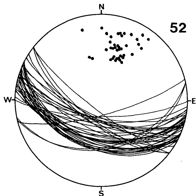
Diagramm 52: Stadelbach – Töplitsch – Weißenbach. Alpinen Muschelkalk, Partnachkalk, Wettersteinkalk. 40 s-Flächen. \beta = 128^{\circ}25'SE .
