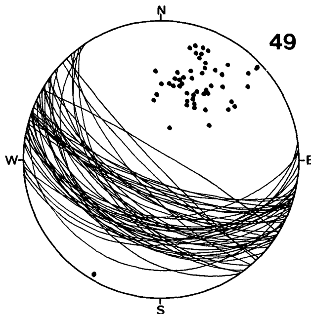
Diagramm 49: Pöllaner Höhe. Alpiner Muschelkalk, Partnachkalk, Wettersteinkalk. 50 s-Flächen. \beta = 140^\circ 20' \text{W} ; \beta = 280^\circ 30' \text{W} ; Ges.- \beta = \text{WNW-ESE} , \pm \text{horizontal} .
