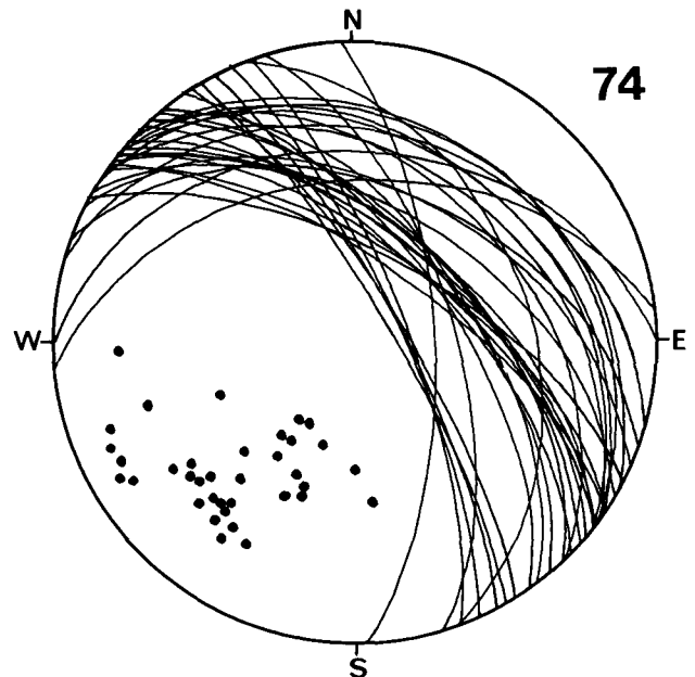
Diagramm 74: Dobratsch: Gipfel, W-Flanke bis Emilhütte. Wettersteinriffkalk. 36 s-Flächen. \beta = 50^{\circ}30'\text{NE} , Bereich Emilhütte \beta = 6^{\circ}30'\text{NE} ; Ges.- \beta = 35^{\circ}35'\text{NE} .
