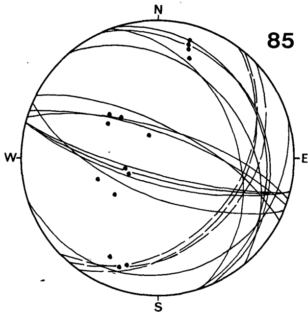
Diagramm 85: Südlich oberhalb und östlich unterhalb Mittewald, westlich Heiligengeist. Oberer Wettersteinkalk. 15 s-Flächen. \beta = 108^\circ 18' \text{ESE} . Ges.- \beta = \text{ca. } 102^\circ 30' \text{ESE} .
