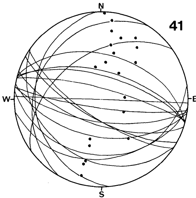
Diagramm 41: Peilgraben, Kreuzenbach. Hauptdolomit. 20 s-Flächen. Einzel- \beta = B = 101^\circ 10'E = 259^\circ 23'W ; = 287^\circ 3'W ; = 292^\circ 24'WNW ; = 300^\circ 22'NW . Ges.- \beta = \text{ca. W-E, } 22^\circ W .
