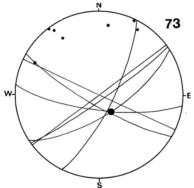
Diagramm 73: Semmler Alm-E. Alpiner Muschelkalk, Schiefer-ton. 7 s-Flächen. \beta = B = 140°70'SE.
