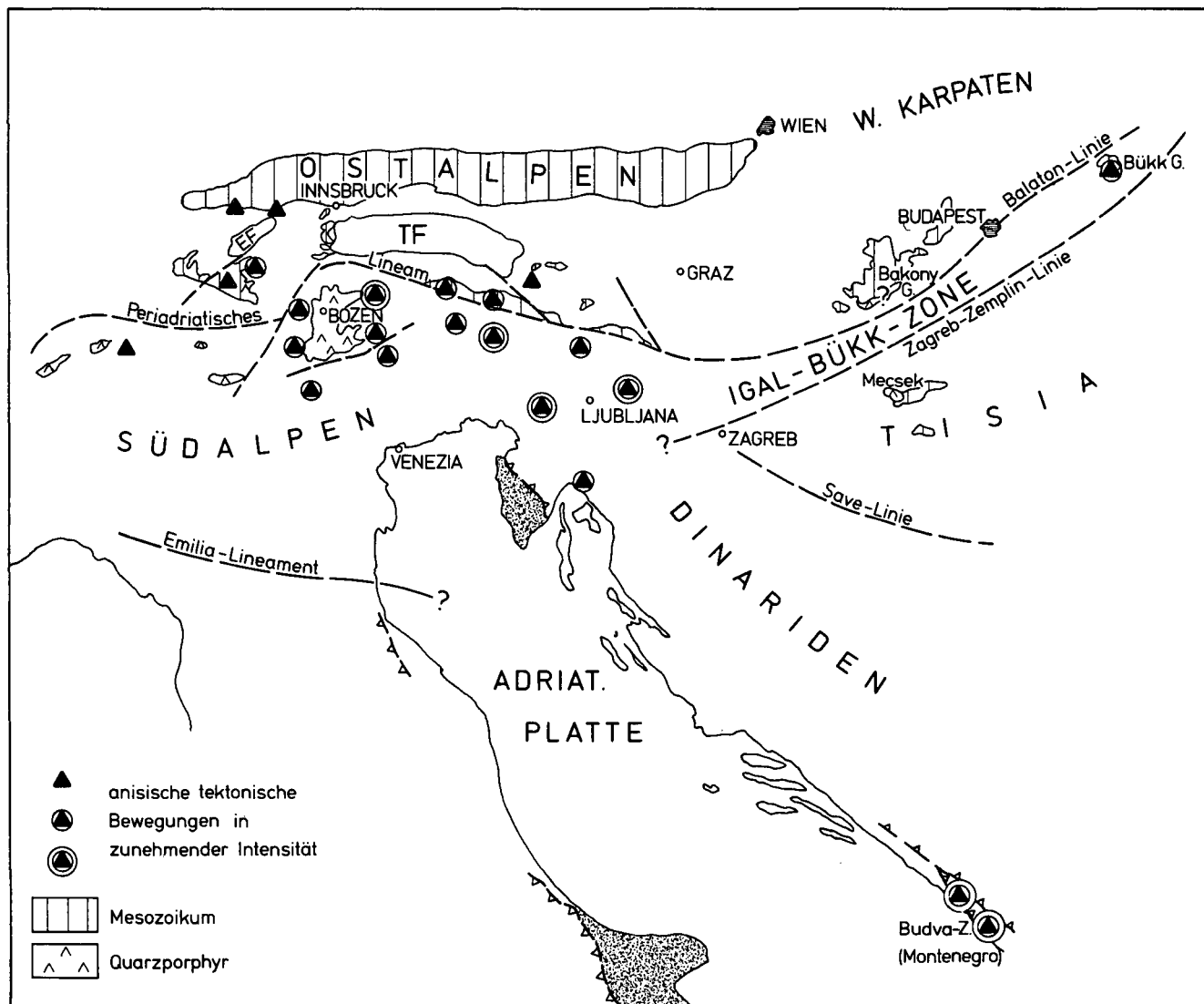
Abb. 22: Räumliche Verteilung von anisischen tektonischen Bewegungen auf der geringfügig veränderten Kartengrundlage nach FLÜGEL (1975), KOVACS (1982) und BOSELLINI (Emilia-Lineament). Deutlich ist der Schwerpunkt der tektonischen Bewegung am N- und E-Rand der Adriatischen Platte zu erkennen.
