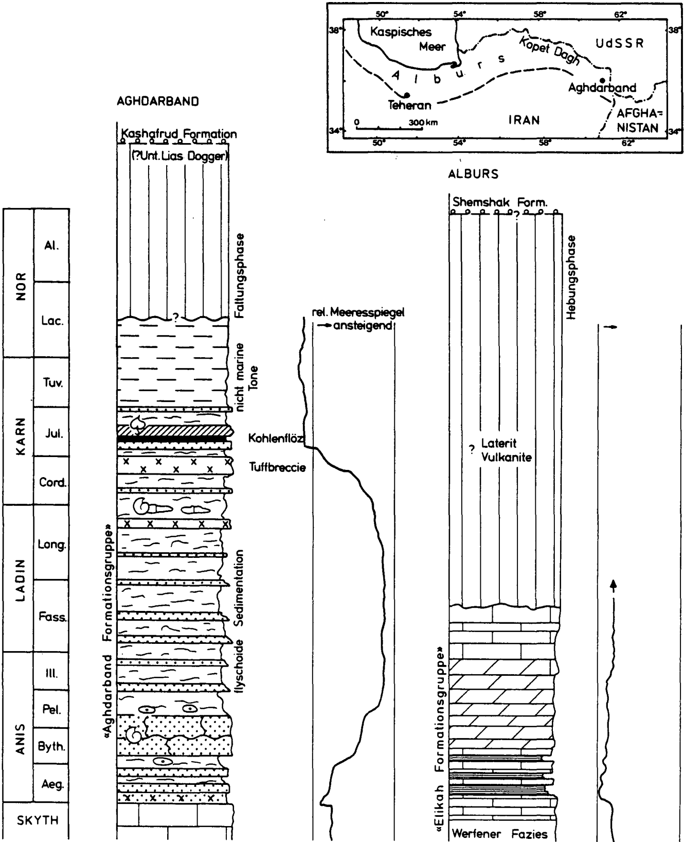
Abb. 5: Gegenüberstellung von Sedimentationsabfolgen mit relativen Meeresspiegelkurven des Tethysnordrandes (Aghdarband) und der zentraliranischen Platte (Alburs); nach RUTHNER (1980), STAMPLI et al. (1976) und eigenen Aufnahmen.
