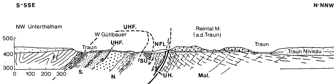
Abb. 2: Profil durch das Ultrahelvetikum-Fenster von Ohlsdorf–Oberweis im Bereich des Ohlsdorfer Grabens.
