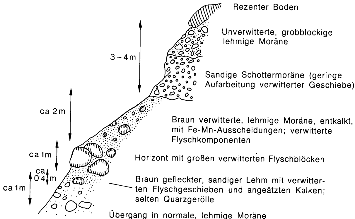
Abb. 4: Verwitterungshorizont zwischen Moränen am Bergvorsprung 750 m östlich P. 538 m (Ohlsdorf). Nach einer Skizze von S. PREY (1946)
