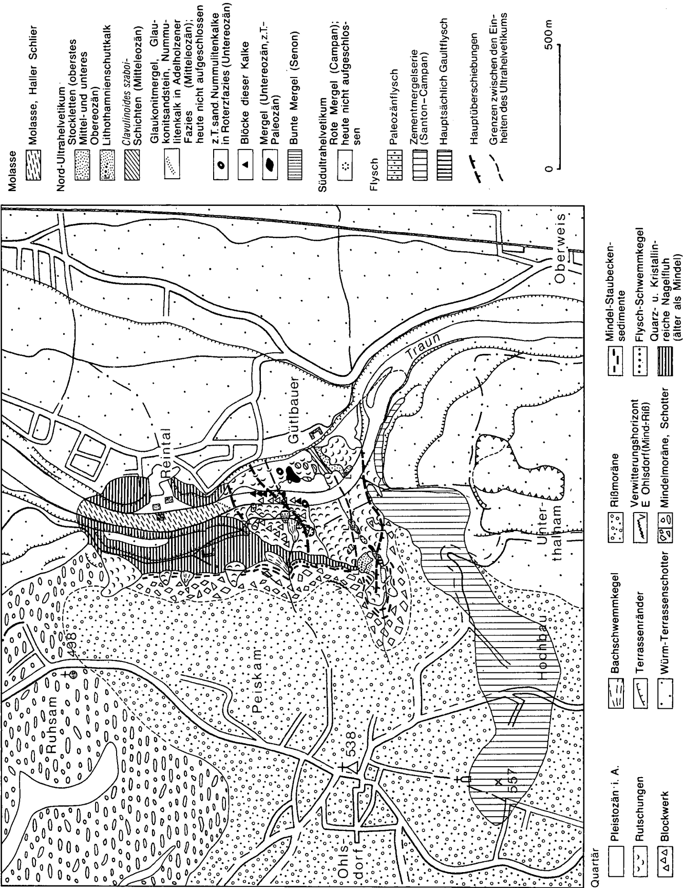
Abb. 1: Geologische Karte des Fensters von Ohlsdorf–Oberweis.
