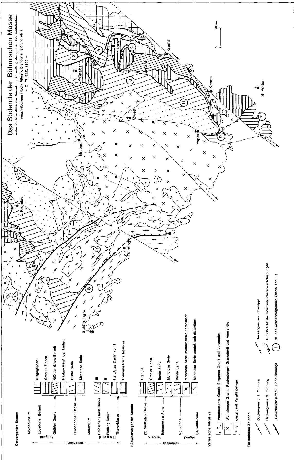
Abb. 2: Tektonische Skizze des Süden der Böhmisches Masse unter Zurücknahme der Versetzungen entlang der großen, linksseitig versetzenden Horizontal-Seitenverschiebungen (Rodl-, Vitiser-, Diendorfer Störung etc.). In der Legende ist „Loosdorfer Einheit“ auf „Loosdorfer Komplex“ zu berichtigen.
