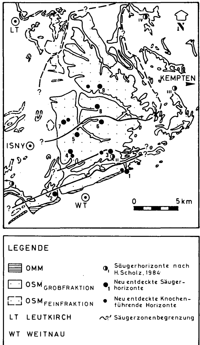
Abb. 9: Übersicht über die Säugetierfundstellen in der OSM und angrenzender OMM der Adelegg.
