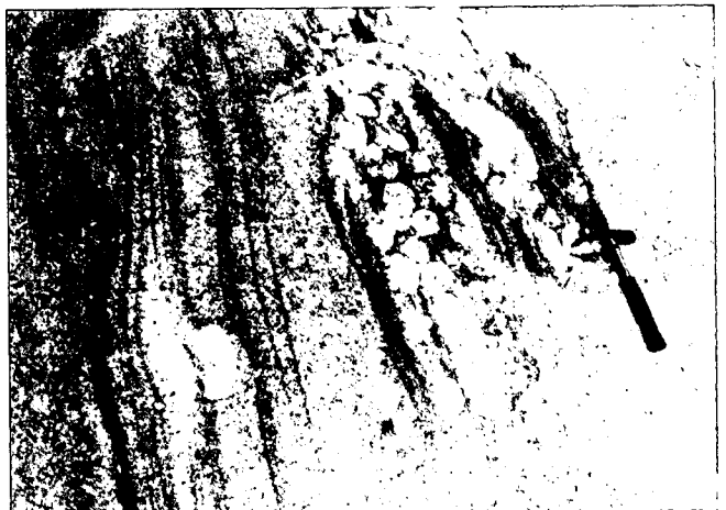
Abb. 7: Magmatische Bänderung und Ansammlung von Orbikuliten im Dach eines granitischen Endoplutons innerhalb der Zentralgneise (Nevestal).
