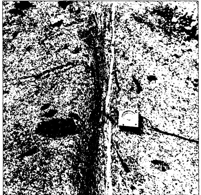
Abb. 13: Duktile Scherzone im Zentralgneis (Hornkees).
