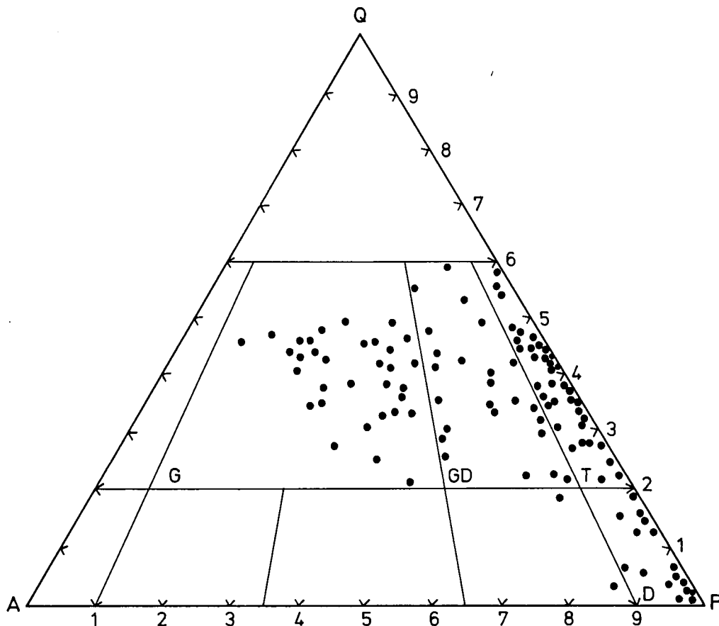
Abb. 6: Nomenklaturdreieck für Plutonite (nach STRECKEISEN, 1976) mit darstellenden Punkten von Zentralgneisen.
