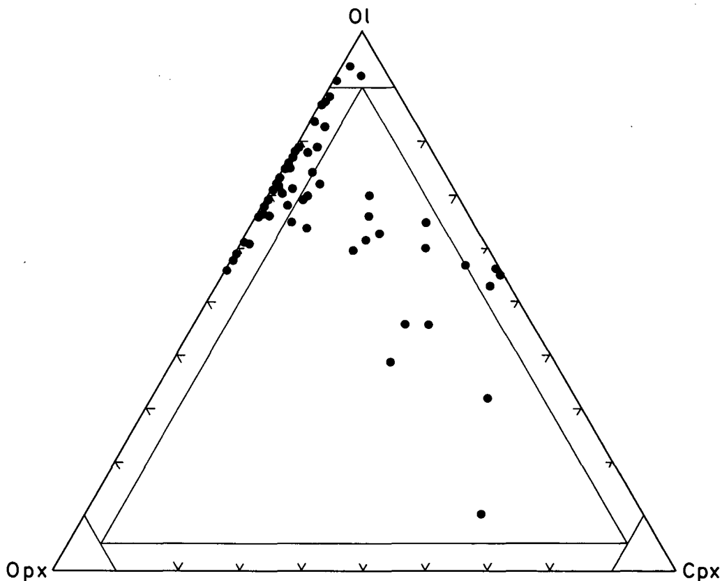
Abb. 5: Nomenklaturdiagramm Ol – Opx – Cpx für Ultramafite nach STRECKEISEN (1976) mit darstellenden Punkten für den Serpentinitt des Ochsner-Rotkopf-Massives aufgrund von CIPW-Normmineralberechnungen.
