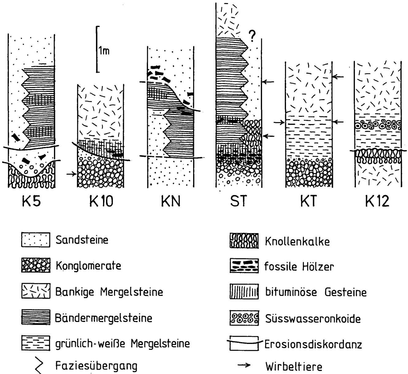
Abb. 5: Sechs etwas generalisierte Profile durch Mergelsteine innerhalb der OSM, die unter dauernder Wasserbedeckung, größtenteils in altwasserartigen Rinnen abgelagert worden sind.
