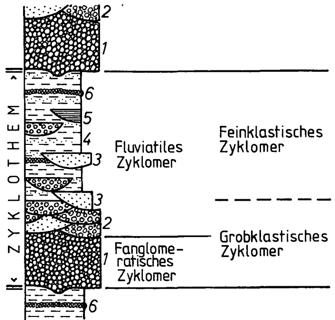
Abb. 2: Schematisches Profil durch die OSM der Adelegg. Zwei mögliche Untergliederungen des Zyklothems in Zyklothem (Zyklothemteile): links nach genetischen, rechts nach lithologischen und morphologischen Gesichtspunkten. 1 = fanglomeratische Konglomerate; 2 = fluviatile konglomeratische Rinnenfüllungen; 3 = sandige Rinnenfüllungen; 4 = Bankige Mergelsteine (Hochwassersedimente); 5 = mergelige Rinnenfüllungen (Altwassersedimente); 6 = Knollenkalke (albsteinartige Bildungen).
