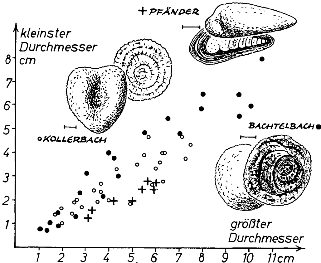
Abb. 9: Morphologie und Schnittbilder von Onkoiden aus der OSM vom Kollerbach (bei Kempten) und Pfänder (bei Bregenz) mit Brodia sp. als Kern. Zum Vergleich ein mehrphasig gewachsenes Onkoid mit internen Diskordanzen aus einem Sandstein-Erratiker, wahrscheinlich aus den terrestrischen Äquivalenten der OMM (vgl. SCHOLZ, 1985) vom Bachtelbach bei Kempten. Der abgebildete Maßstab ist jeweils 1 cm lang. Diagramm mit den größten und kleinsten Durchmessern aus diesem Vorkommen.
