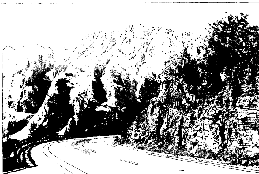
Abb. 10. Blick von der Roßfeldringstraße zum Hohen Göll. Rechts neben der Straße sind Roßfeldschichten aufgeschlossen. Sie wurden wahrscheinlich nie über 100°C erwärmt, da das Apatit-Spaltspurenalter der Probe 15 wesentlich höher als deren Sedimentationsalter ist. Probe 15 wurde ca. 4 km östlich von dem hier abgebildeten Aufschluß aus den Roßfeldschichten entnommen.
