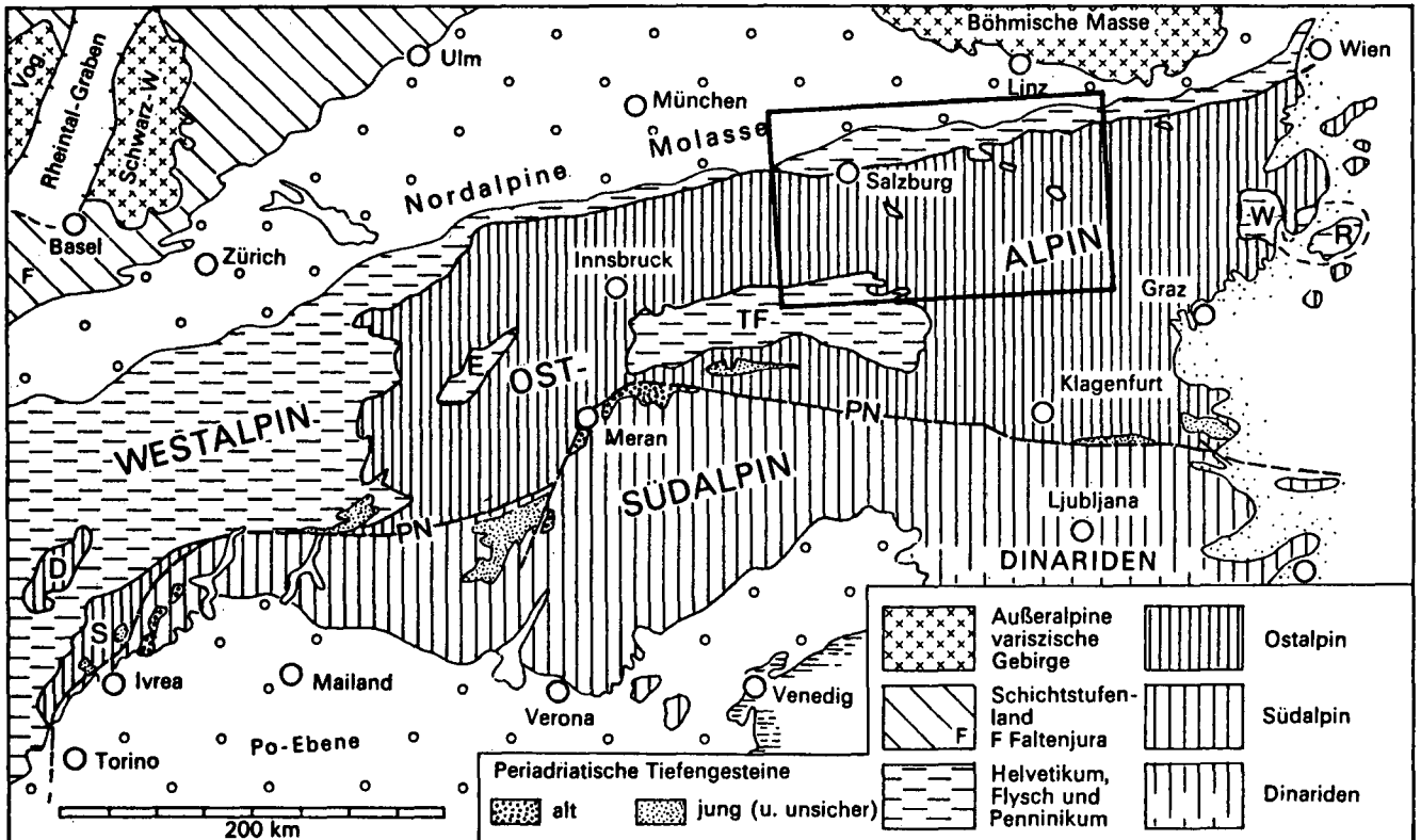
Abb. 2. Tektonische Übersichtskarte der Ostalpen (nach H. BÖGEL & K. SCHMIDT, 1976) mit Lage des Arbeitsgebietes (rechteckig umrahmt).
