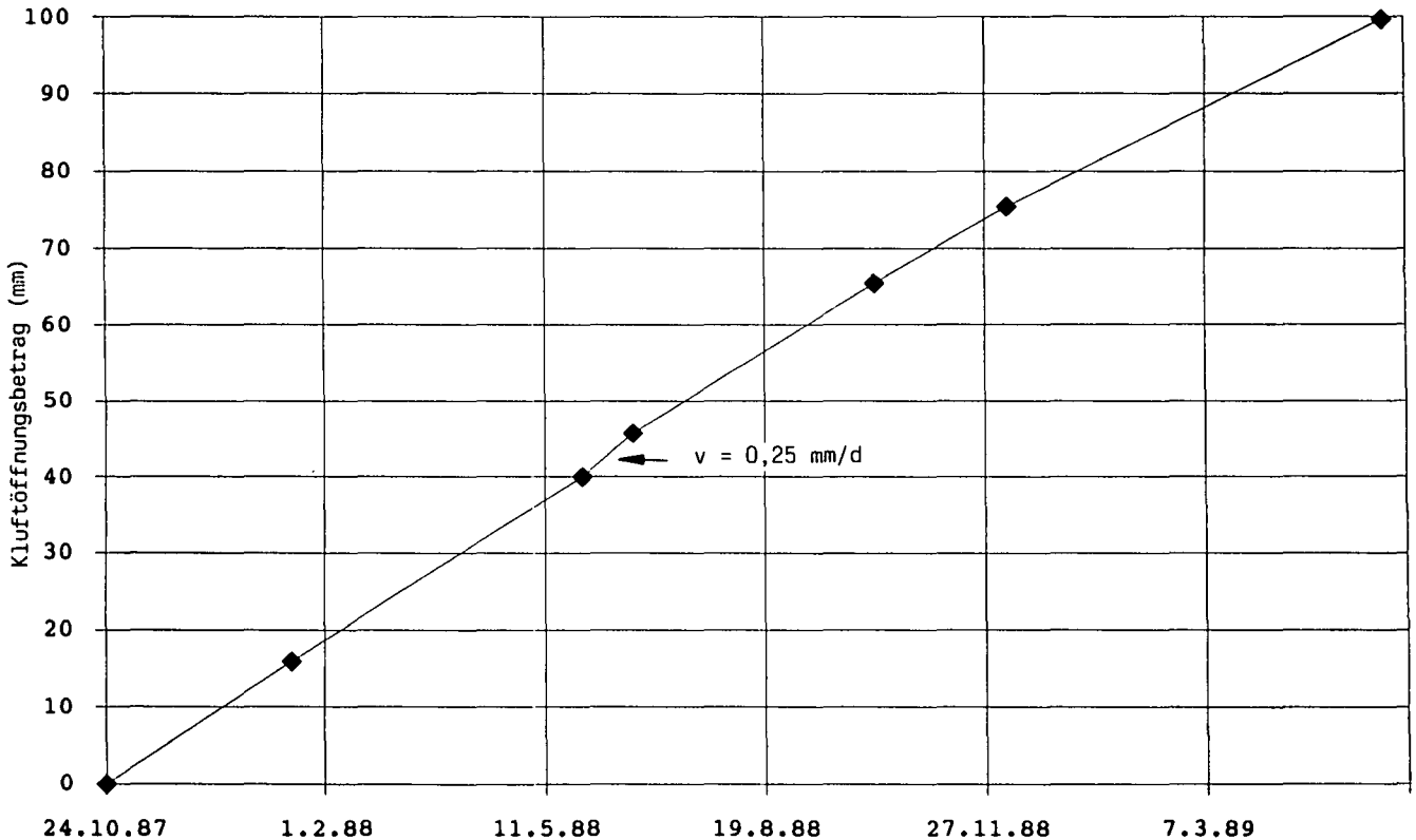
Abb. 6. Ergebnisse der Stahlband-Extensometermessungen an der Großkluff des Blockes 1. Die Meßpunkte sind als Rauten dargestellt.
