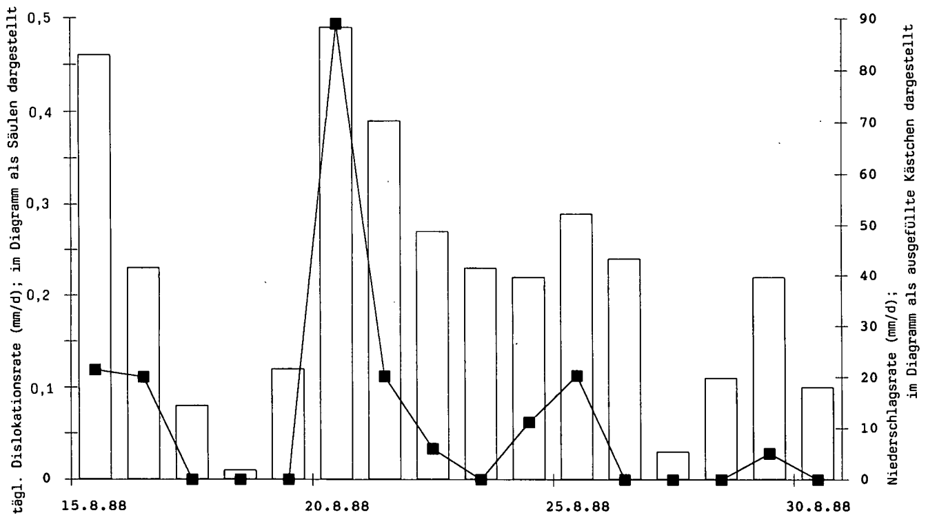
Abb. 10. EDV-gestützte ausgewertete Meßergebnisse der Präzisionsexensometer-Messungen und der Niederschlagsmessungen der meteorologischen Station am Naßfeldpaß. a) Zeitraum vom 23. 06. 1988 - 30. 11. 1988. b) Zeitraum vom 15. 08. 1988 - 30. 08. 1988.
