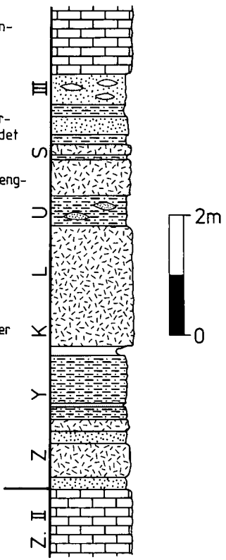
PROFIL DER 'KLASTISCHEN', BASALEN ABFOLGE DES ZYKLUS 3 DER UNTEREN PSEUDOSCHWAGERINEN-SCHICHTEN (UPK)
