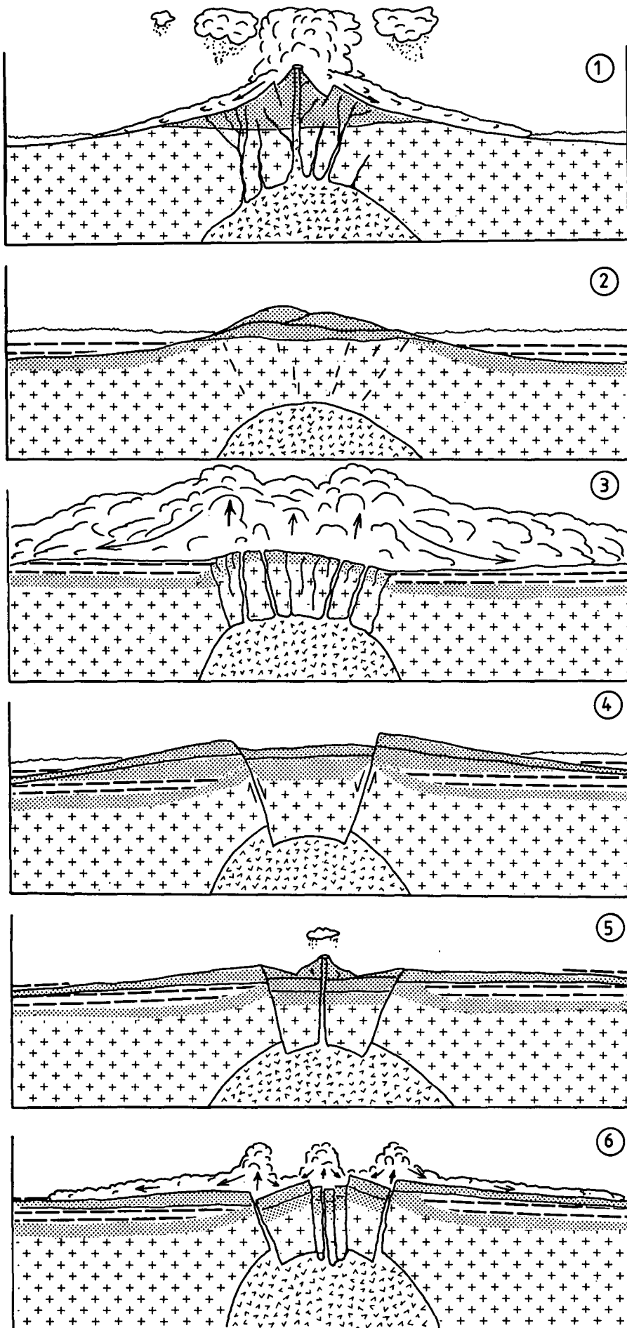
Abb. 18. Vulkanologisches Modell für die Bildungs- mechanismen der Meta-Pyroklastite unter dem Blasseneck-„Porphyroid“ (1), der Meta- Klastite (2), des Blasseneck-„Porphyroids“ (3 und 4) und der Meta-Pyroklastite über dem Blasseneck-„Porphyroid“ (5 und 6). Nähere Erläuterung siehe Text.
