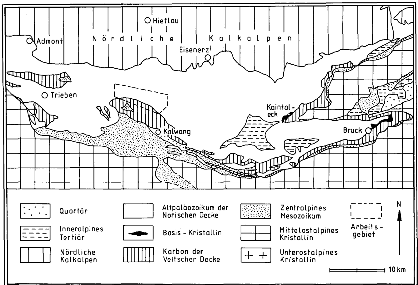
Abb. 1. Geologische Karte der Umgebung des Untersuchungsgebietes. Vereinfacht nach SCHÖNLAUB (1982).
