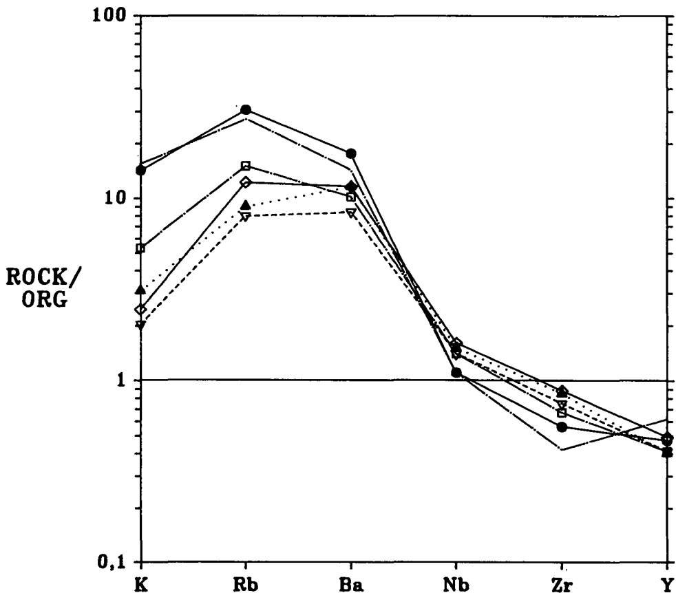
Abb. 16. K-, Rb-, Ba-, Nb-, Zr- und Y-Werte von 6 ausgewählten Proben des Blasseneck-„Porphyroids“, normiert mit entsprechenden Werten von Graniten mittelozeanischer Rücken („Rock/ORG“) nach PEARCE et al. (1984).
