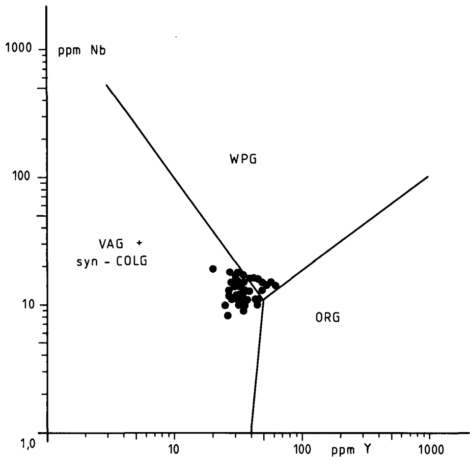
Abb. 15. 42 Analysen des Blasseneck-„Porphyroids“ mit mehr als 60 % SiO 2 in einem Nb-Y-Diagramm nach PEARCE et al. (1984), mit dessen Hilfe man Granitoide unterschiedlicher geotektonischer Positionen unterscheiden kann. ORG = „Ocean Ridge Granite“; WPG = „Within Plate Granite“; VAG + syn-COLG = „Volcanic Arc Granite“ und „syncollisional Granite“.
