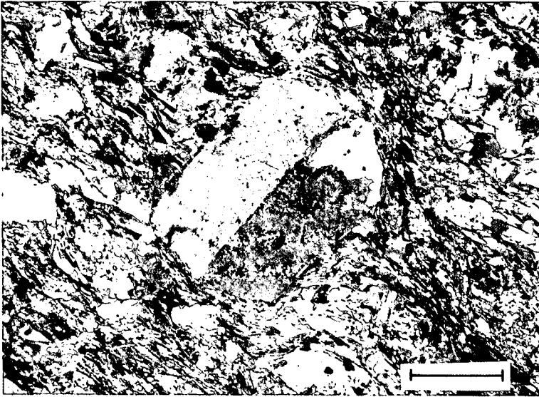
Abb. 7. Dünnschliff-Photographie des Biotit-Gneises. Einsprengling eines großen Kalifeldspates in einer Grundmasse aus Quarz, Feldspat und Biotit. Maßstab = 1 mm. Lokalität: Nördliche Flanke des Kurzteichenbachtals 500 m E Jagdhaus Don.
