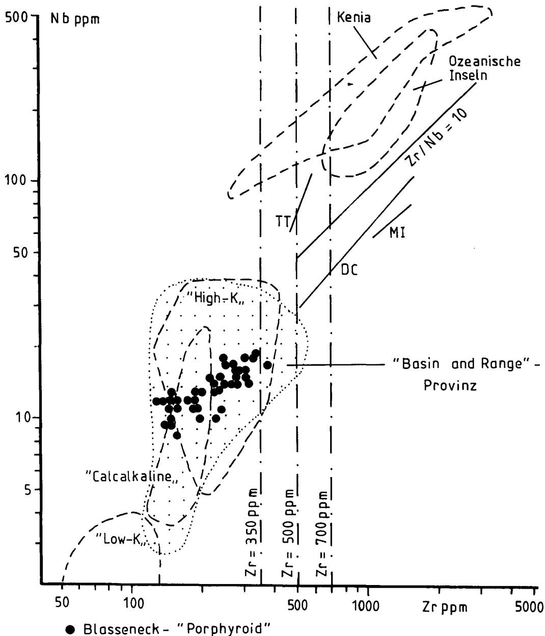
Abb. 14. Nb-Zr-Diagramm nach LEAT et al. (1986), das die Streubreite intermediärer und saurer Vulkanite mit mehr als 60 % \text{SiO}_2 zeigt. Punkte = 42 Analysen des Blasseneck-„Porphyroids“; Punktfeld = Analysen oligozäner und miozäner Vulkanite aus der „Basin and Range“-Provinz nach BEST et al. (1989); MI = Vulkanite von Mayor Island (Neuseeland) nach EWART (1968); DC = Vulkanite von Devine Canyon (Oregon/U.S.A.) nach GREENE (1973); TT = Vulkanite des Tala Tuff (Mexiko) nach MAHOOD (1981).
