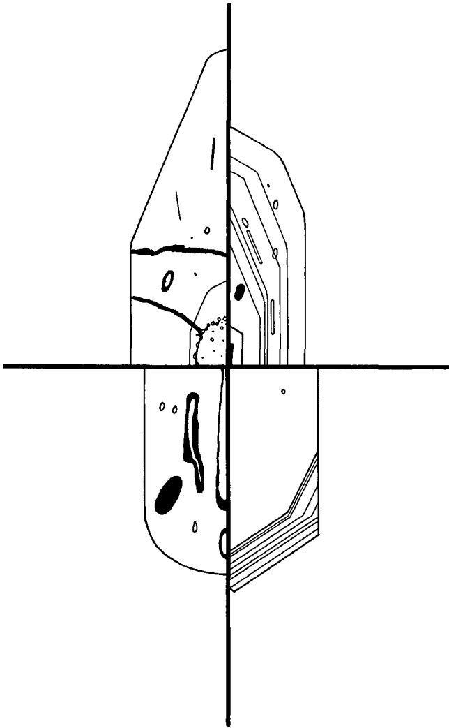
Abb. 14. Granodioritporphyritzirkone (9953).
