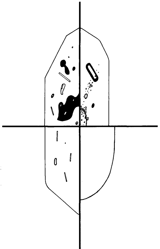
Abb. 11. Tonalitporphyritzirkone (10174).
