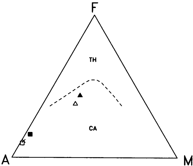
Abb. 2. AFM-Diagramm (nach IRVINE & BARAGAR, 1971) der untersuchten Gesteine. x = Flasergneis, Sesvennagruppe; Δ = Tonalitporphyrit, Töll; □ = Tonalitporphyrit, Iseltal; □ = Mikrogranitporphyr, Sesvennagruppe; ■ = Granodioritporphyrit, Sesvennagruppe; - - - = Grenzlinie zwischen kalkalkalischen (CA) und tholeiitischen (TH) Trends (nach RICKWOOD 1989).
