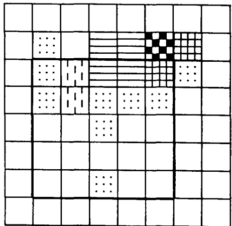
6 (n = 101) Flaserigneis
