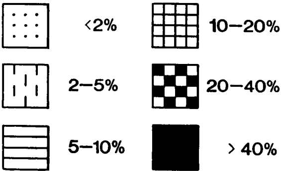
9953 (n = 26) Granodioritporphyrit
