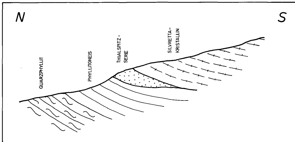
Abb. 1. Darstellung der geologischen Verhältnisse im Grenzbereich Phyllitgneiszone-Silvretakristallin nach L. KRECZY (1981, Abb. 79). Das Silvretakristallin liegt schüsselförmig über dem Alpenen Verrucano (Thialspitzserie) und den Gesteinen der Quarzphyllit- und Phyllitgneiszone.
