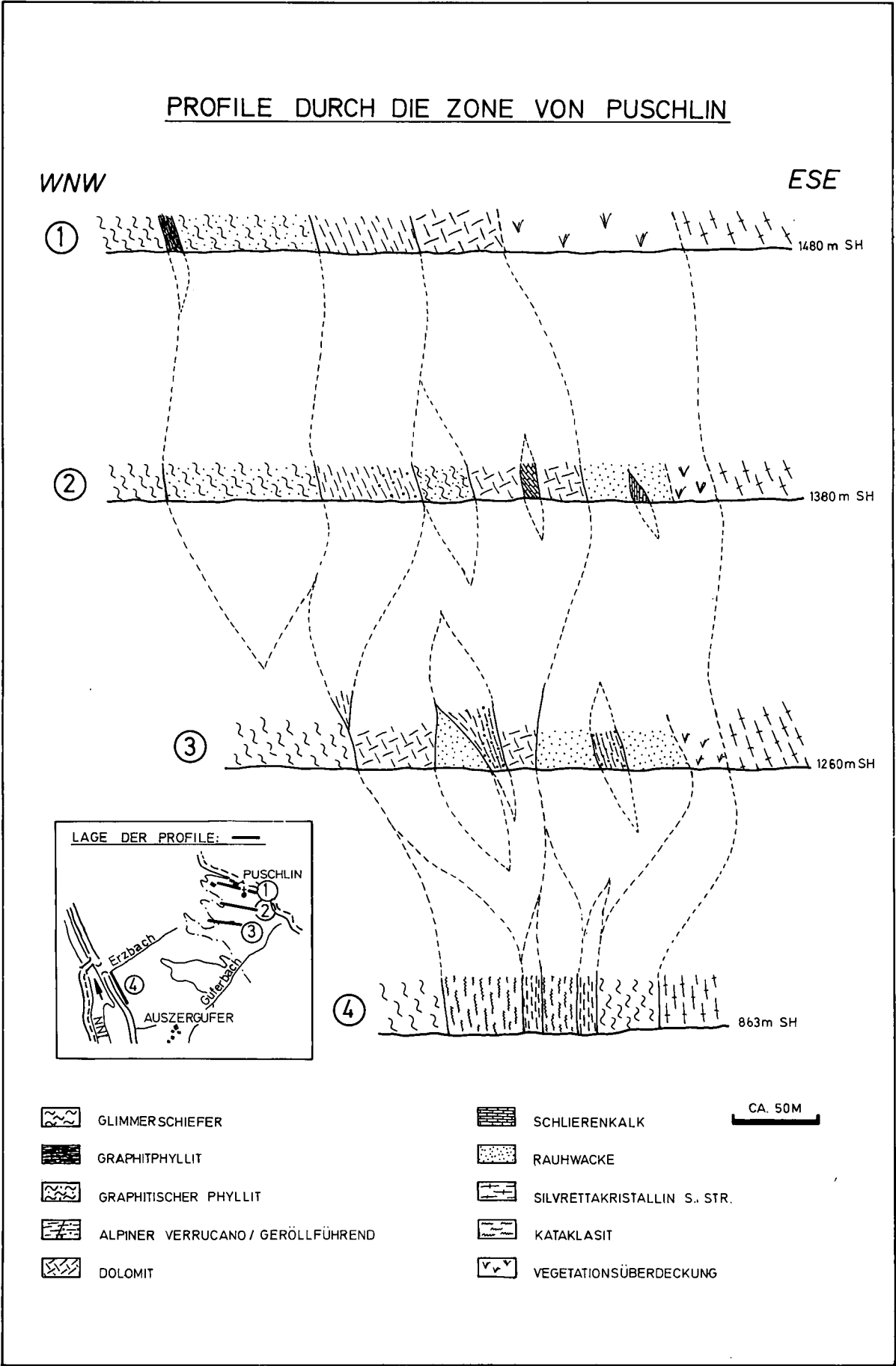
Abb. 2. Die alpidisch schwach metamorph überprägten Gesteine dieser Zone liegen in Form isolierter Linsen vor, deren stratigraphischer Zusammenhang im Zuge der Tektonik verloren ging.
