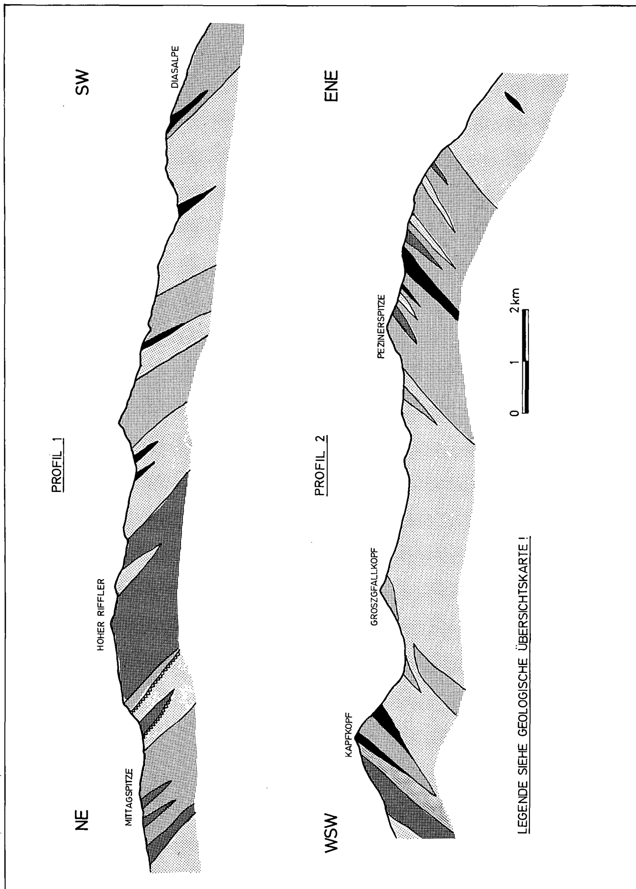
Abb. 7. Profile durch die nordöstliche Ferswallgruppe. Die Legende und die Lage der Profile sind aus Abb. 6 ersichtlich.
