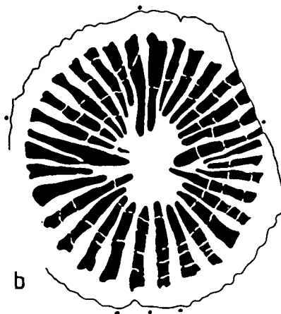
Abb. 11. Rotiphyllum rushianum major n.ssp. a,b) 63 JE 13/10, 4,8°.
