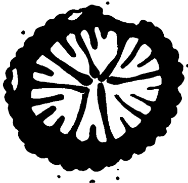
Abb. 21. Ufimia sp. Gruppe U. inaequale SCHINDEWOLF, 1940. 65 AR 233/17; 2,1x.
