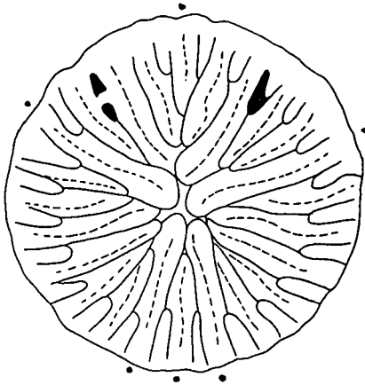
Abb. 17. Ufimia aff. infracarbonica SCHINDEWOLF, 1942. 66 HF 78/5; 4,8x.
