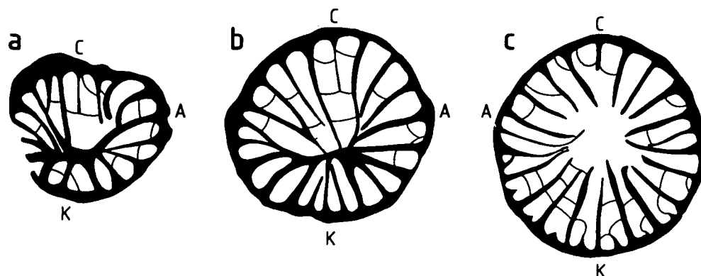
Abb. 8. Ontogenetisch unterschiedliche Stadien bei Zaphrentites genis HUDSON nach HUDSON (1944). a) Zaphrentoides Stadium. b) Allotrophyloides Stadium. c) Amplexoides Stadium.
