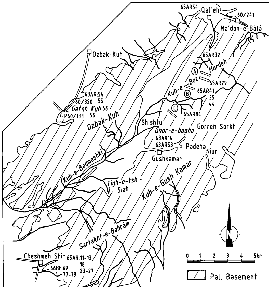
Abb. 3. Position der Fundpunkte auf Blatt Ozbah-Kuh. Genze des paläozoischen Grundgebirges nach A. RUTTNER (unveröffentlicht). In Abb. 3–6 wurden sämtliche Fundpunkte der Sadar-Fm. verzeichnet, aus denen Material zur Bearbeitung vorliegt).
