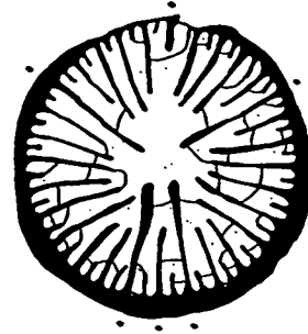
Abb. 22. Ufimia cf. longiseptata (FRECH, 1889). 66 HF 78/2A; 2,1x.
