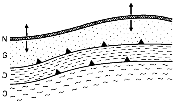
Fig. 4. Schema der Entwicklung der südöstlichen Böhmisches Masse im Ordoviz-Silur.
