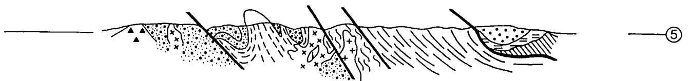
Abb. 3. Profil durch das Bavarikum in Oberösterreich (FUCHS, 1990).
