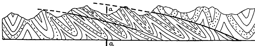
Fig. 8. Schematische Darstellung der zwei rhätischen Überschiebungen ohne Berücksichtigung der späteren bei a-a eingetretenen Störung.
