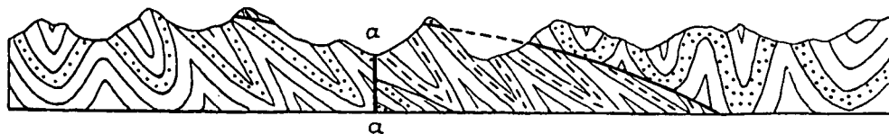
Fig. 9. Schematische Darstellung der späteren Störung (Absinken des Gebirges rechts der Spalte a-a) die im Rheinthal zwischen Chur und Bodensee eingetreten ist.
