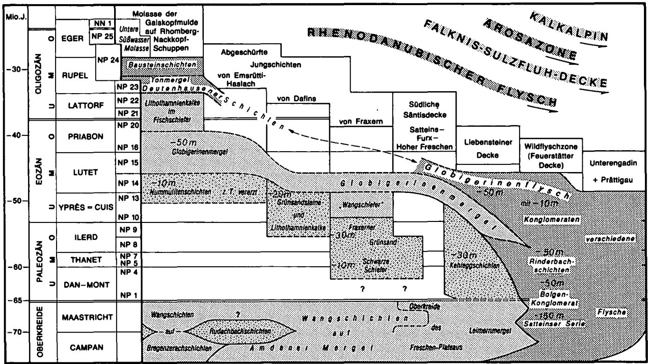
Abb. 4. Die Schichtfolge der höchsten Oberkreide und des Alttertiär im Helvetikum und nördlichen Penninikum in Vorarlberg unmittelbar vor ihrer nordvergenten Tektonisierung zur Molassezeit, mit aufliegendem, vorher bis zum Ypres (Cuis) westvergent bewegtem, südpenninisch-ostalpinem Deckel.
