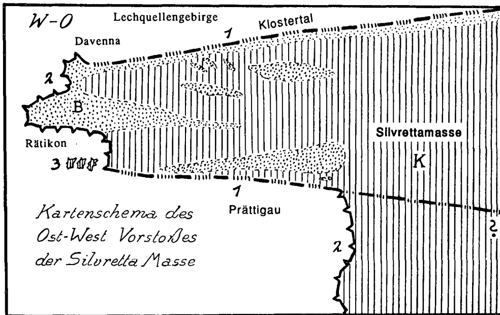
Fig. 14. 1 = steilstehende Verschiebungsbahn. 2 = flachliegende Schubfläche. 3 = Schubschollen. K = Silvrettakristallin. B = Auflagerungen von Verrucano-Buntsandstein und jüngeren Schichten. Zu Fig. 14 stellt Fig. 15 einen schematischen Längsschnitt dar.
