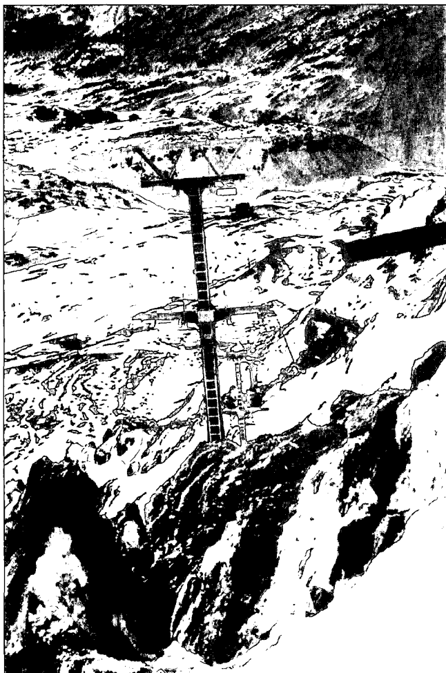
Abb. 14. Doppelsesselbahn Schindlergrat St. Anton a. A. Ansicht der verankerten Stützen in den Arlbergschichten der Südostwand.
