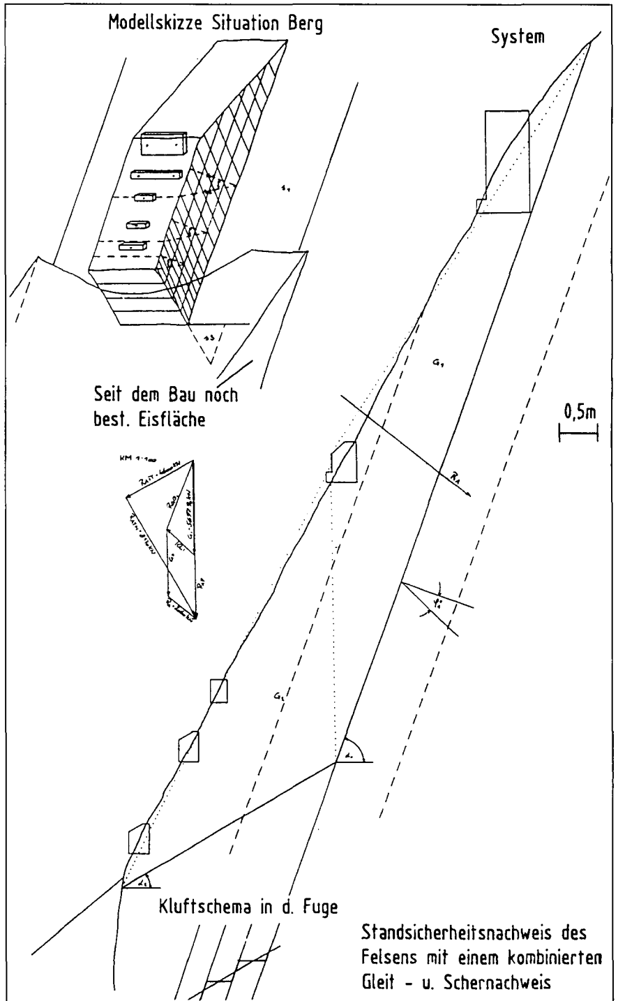
Abb. 18. Gletscherschlepplift Dauferner II (Stubai Gletscher-Schigebiet). Modellskizze, Kluff-, Lage- und Kräftesystem der Standsicherheitsuntersuchung der Antriebs- und Abspannstation Berg.
