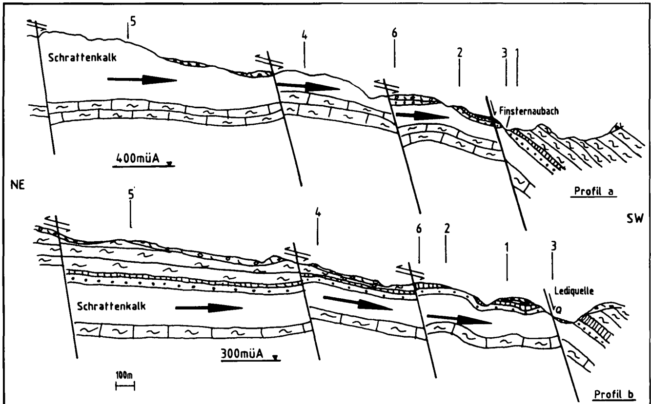
Abb. 6. Lediquellen Hohenems: Achsialschnitte der Alimentationswege durch die verkarsteten Schraffenkalkschenkel des Ranzenberg-Staufenspitz- und des Götznberg-Strahlkopf-Bocksbergsgewölbes.
