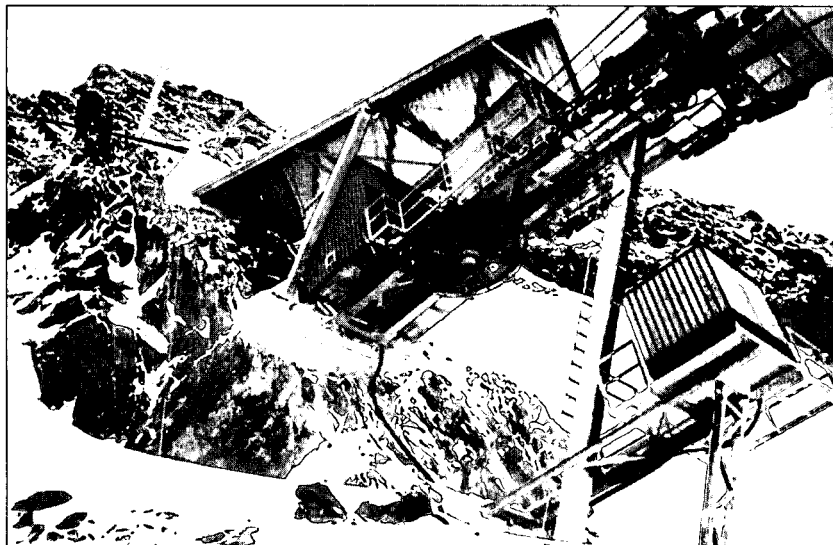
Abb. 19. Gletscherschleplift Daunferner II (Stubai Gletscher-Schigebiet). Horizontal verankerte Bergstation mit Antrieb, Ab- spannung und Trafo.
