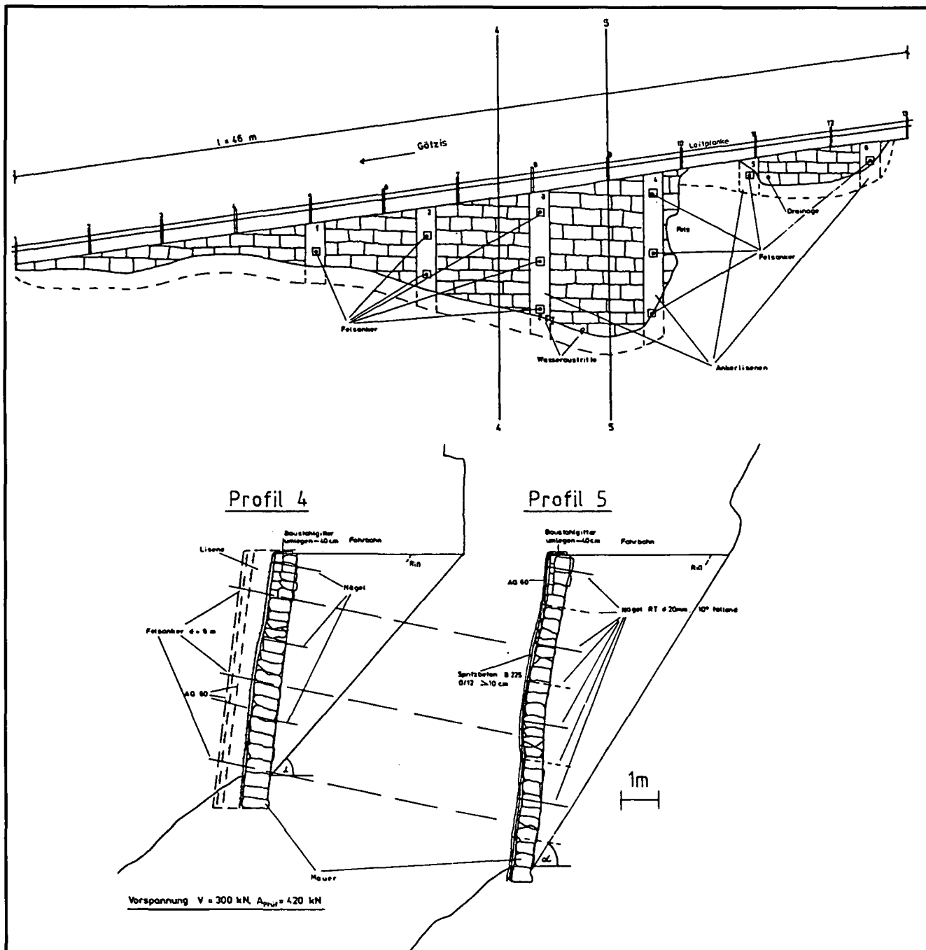
Abb. 9. Meschach-Götzis. Ausführungspläne der Maueranierung „Fuchsfalle“ mit Baustahlgitter, Microsilika-Spritzbeton, Mauernägeln und Dauerankern.
