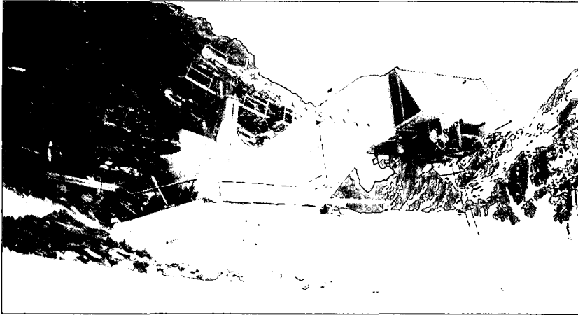
Abb. 17. Doppelsesselbahn Dauferner I (Stubai Gletscher-Schigebiet). Horizontal im Quarzitzgneis über die Randkluft aus- ragend geankerte Talstation.
