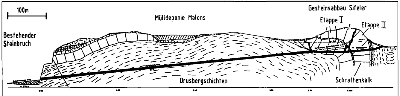
Abb. 10. Sifeler-Weiler/Röthis. Erschließungstunnel vom bestehenden Steinbruch Röthis aus und Kalkgesteinsabbau Etappe I kesselförmig hinter einer Abschirmrippe sowie Endabbauabschnitt II.
