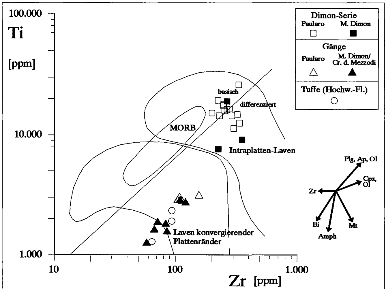
Abb. 16. Ti-Zr-Diagramm nach PEARCE (1982) zur Unterscheidung von Vulkaniten unterschiedlicher plattentektonischer Stellung angewandt auf spilitisierte Basalte und Basalt-Tuffe der Dimon-Serie, Aschentuffe des Hochwipfelflysches und spät- bis postvariskische Gänge, die die Dimon-Serie und den Hochwipfelflysch durchschlagen.
