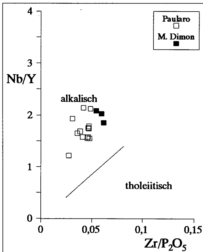
Abb. 11. Nb/Y-Zr/P 2 O 5 -Diagramm zur Unterscheidung alkalischer und tholeiitischer Basalte nach FLOYD & WINCHESTER (1975) für die spilitisierten Basalte und Basalt-Tuffe der Dimon-Serie. Die Trennungslinie ist von WINCHESTER & FLOYD (1976) übernommen.
