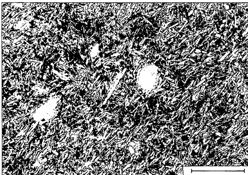
Abb. 10. Dünnschliff-Photographie eines spilitisierten Alkali-Basaltes aus der Dimon-Serie. Leicht fluidal eingeregelter Plagioklase liegen in einer Grundmasse aus Chlorit und Erz. Lokalität Torrente Chiarzò. Gekreuzte Nicols. Maßstab 2 mm.
