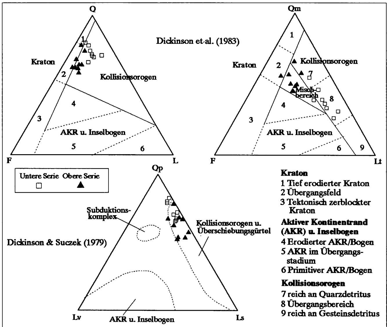
Abb. 8. Modaler Mineralbestand der Grauwacken des Hochwipfflylsches („Untere“ und „Obere Serie“, siehe Text) in Diagrammen nach DICKINSON et al. (1983) und DICKINSON & SUCZEK (1979). Qm = Monokristalliner Quarz, Qp = Polykristalliner Quarz, Q = Qm + Qp, F = Feldspäte, Ls = (Meta-) Sedimentäre Gesteinsbruchstücke, Lv = (Meta-) Vulkanische Gesteinsbruchstücke, L = Lv + Ls, Lt = Lv + Ls + Qp.
