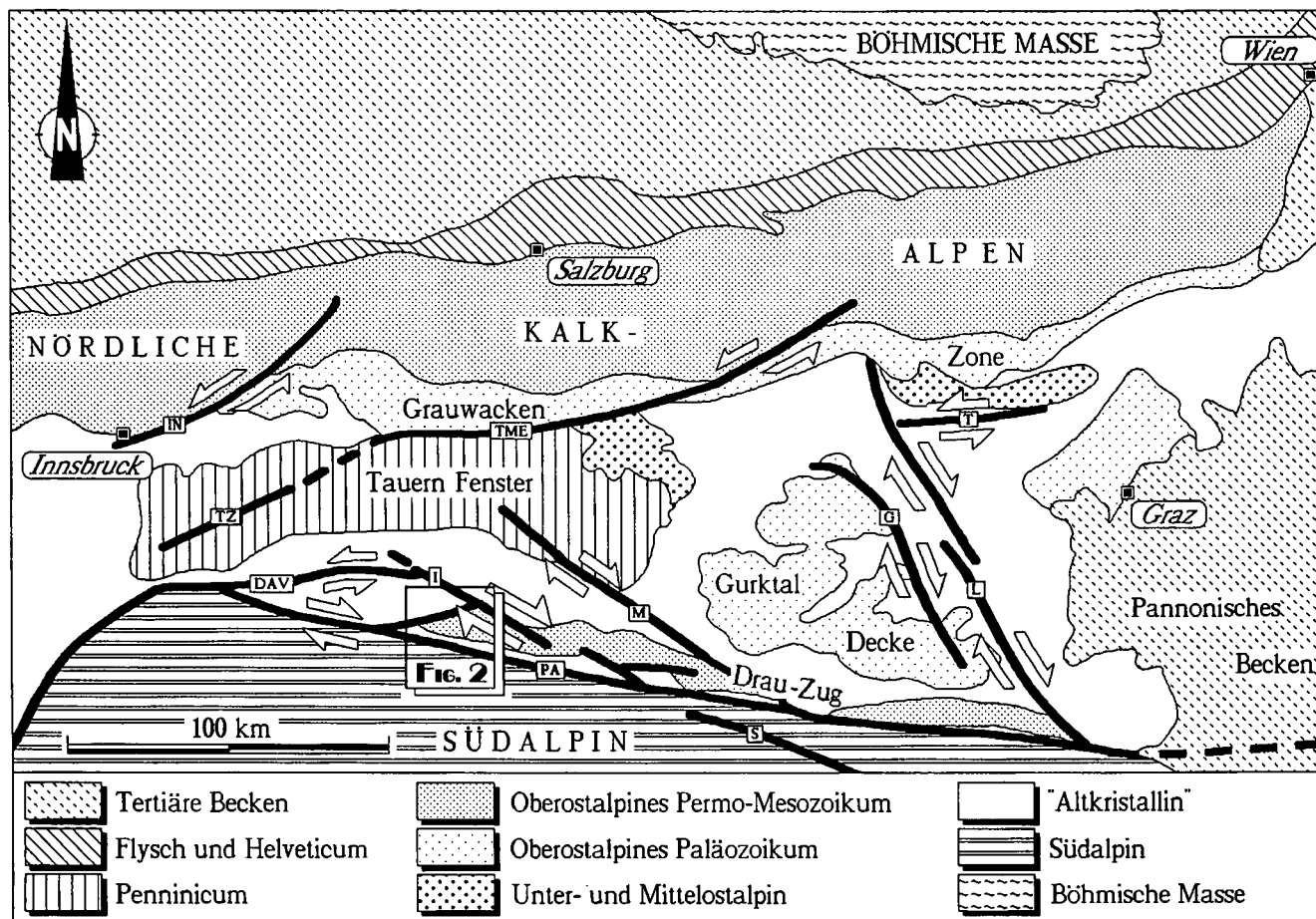
Abb. 1. Vereinfachte tektonische Übersichtskarte der Ostalpen mit den wichtigsten tertiären Blattverschiebungen (abgeändert nach NEUBAUER, 1988 und CHANNELL et al., 1990).
