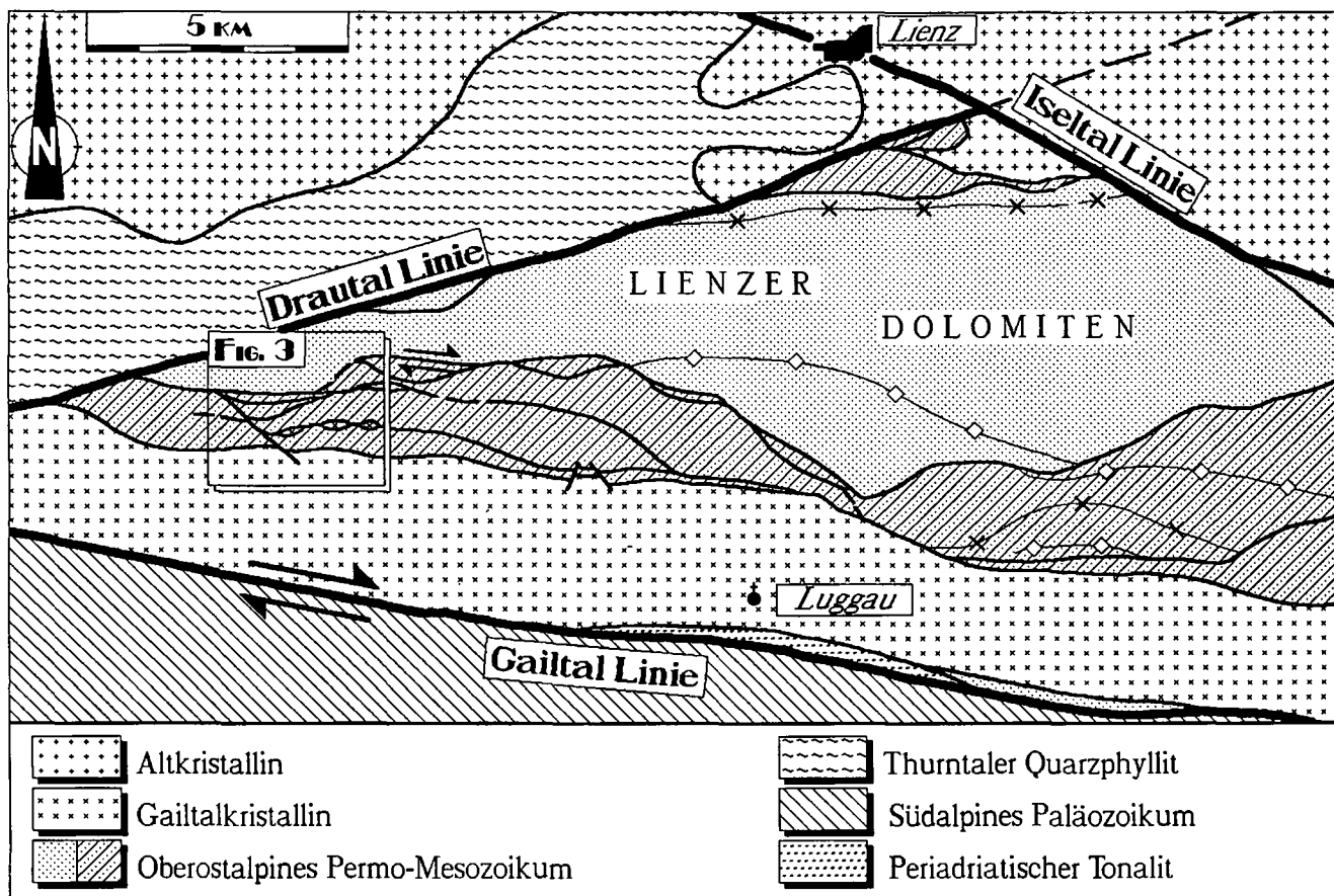
Abb. 2. Tektonische Übersichtskarte der Lienzer Dolomiten. Deutlich wird der zusammenhängende Zentralteil (punktiert), dem verschiedene tektonostratigraphische Einheiten im N und S (schrägschraffiert) gegenüberstehen. Diese sind in Bezug auf den Zentralteil als allochthon anzusehen. Zu beachten ist auch das eingeschuppte Permo-Mesozoikum an der Gaital-Linie (abgeändert nach VAN BEMMELN & MEULENKAMP, 1965; SCHLAGER, 1963; ZANFERRARI, 1976, sowie eigenen Geländedaten).
