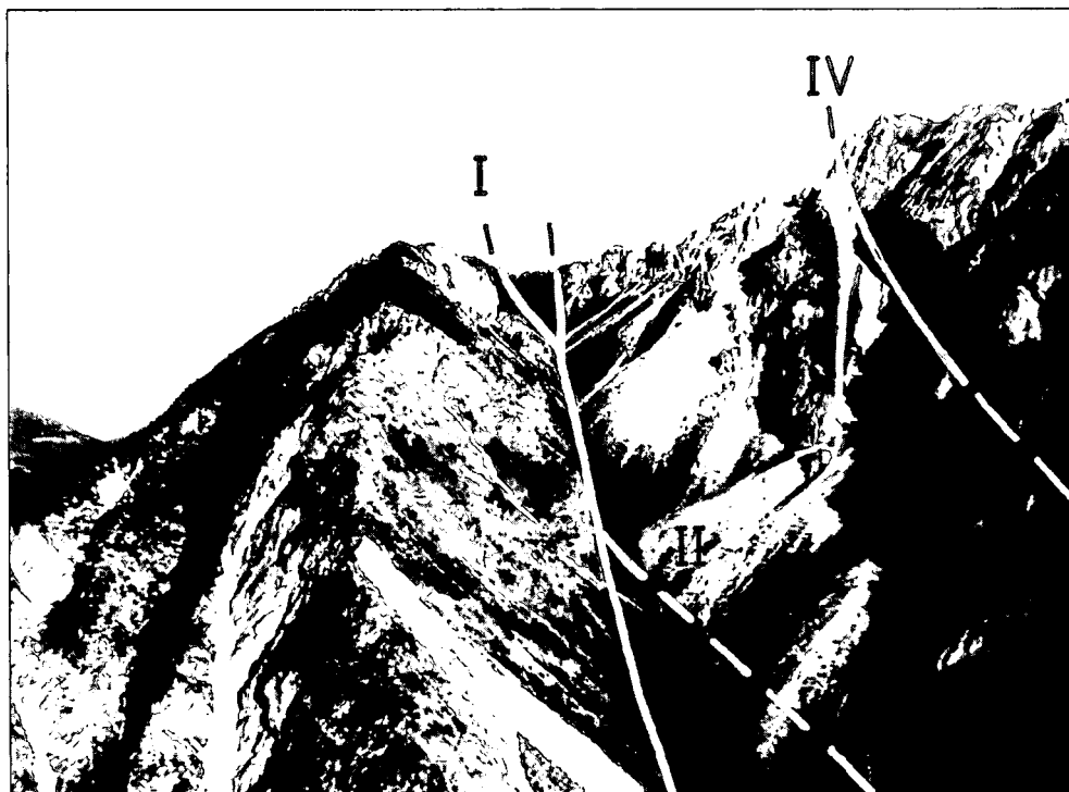
Abb. 5. Blick vom Rainer Berg nach E in die Schlucke. Die Nummern der Störungen entsprechen den Nummern von Abb. 3.
