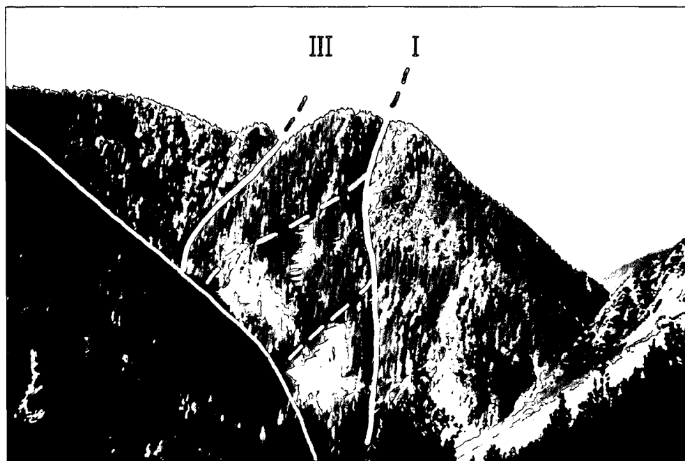
Abb. 7. Blick vom Schluckenriegel im E auf die Blumenstruktur im Rainer Berg vgl. auch Profil Abb. 4. Die Nummern der Störungen entsprechen den Nummern von Abb. 3.
