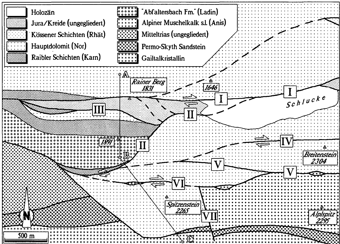
Abb. 3. Vereinfachte geologische Karte der westlichen Lienzer Dolomiten zwischen Jochbach im W und Sturzelbach im E (Lokation siehe Abbildung 2).
