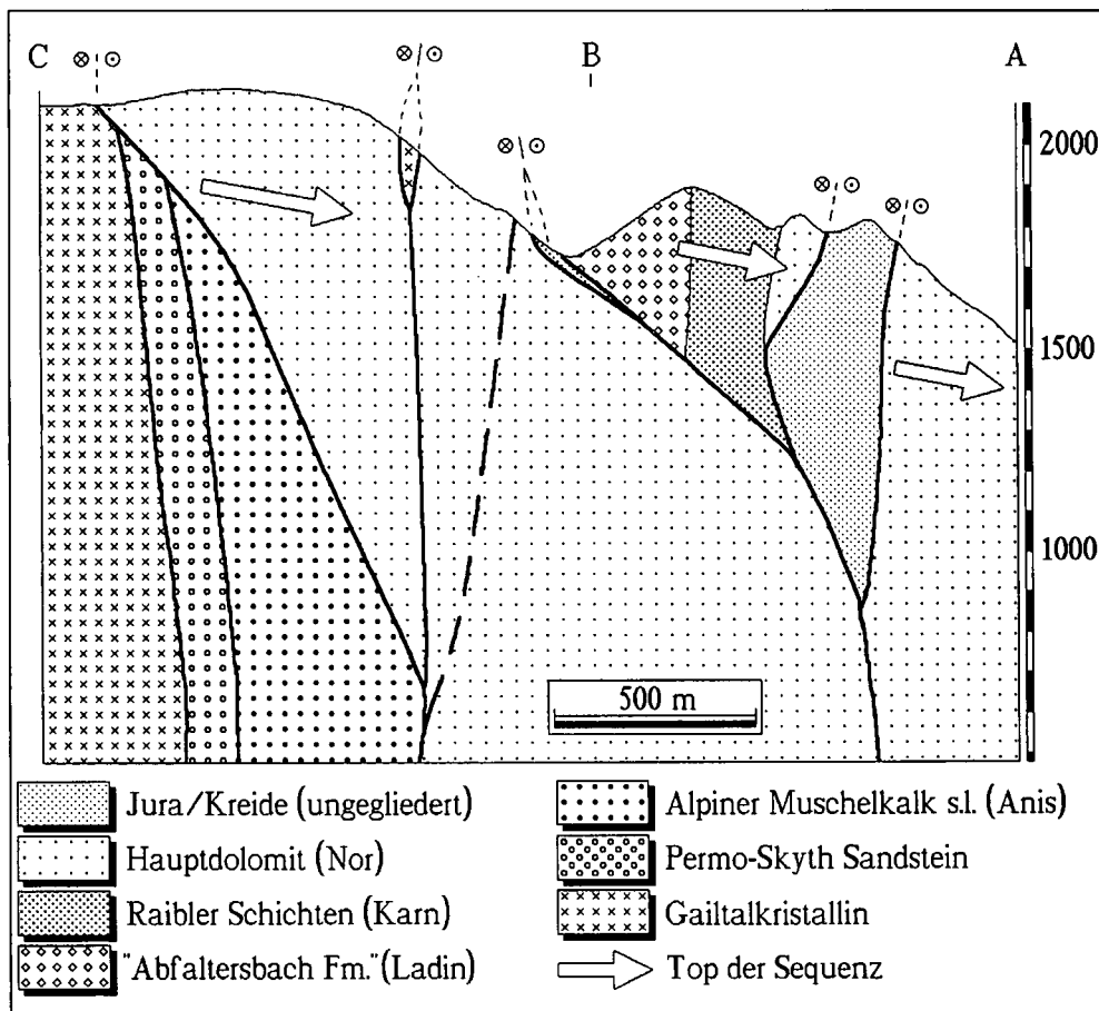
Abb. 4. Profil durch die positive Blumenstruktur am Rainer Berg entsprechend der Profillinie in Abb. 3.
