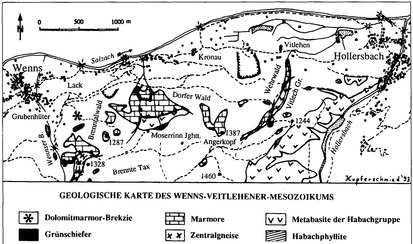
Abb. 2. Geologische Karte des Wenns-Veitlehener-Mesozoikums.
