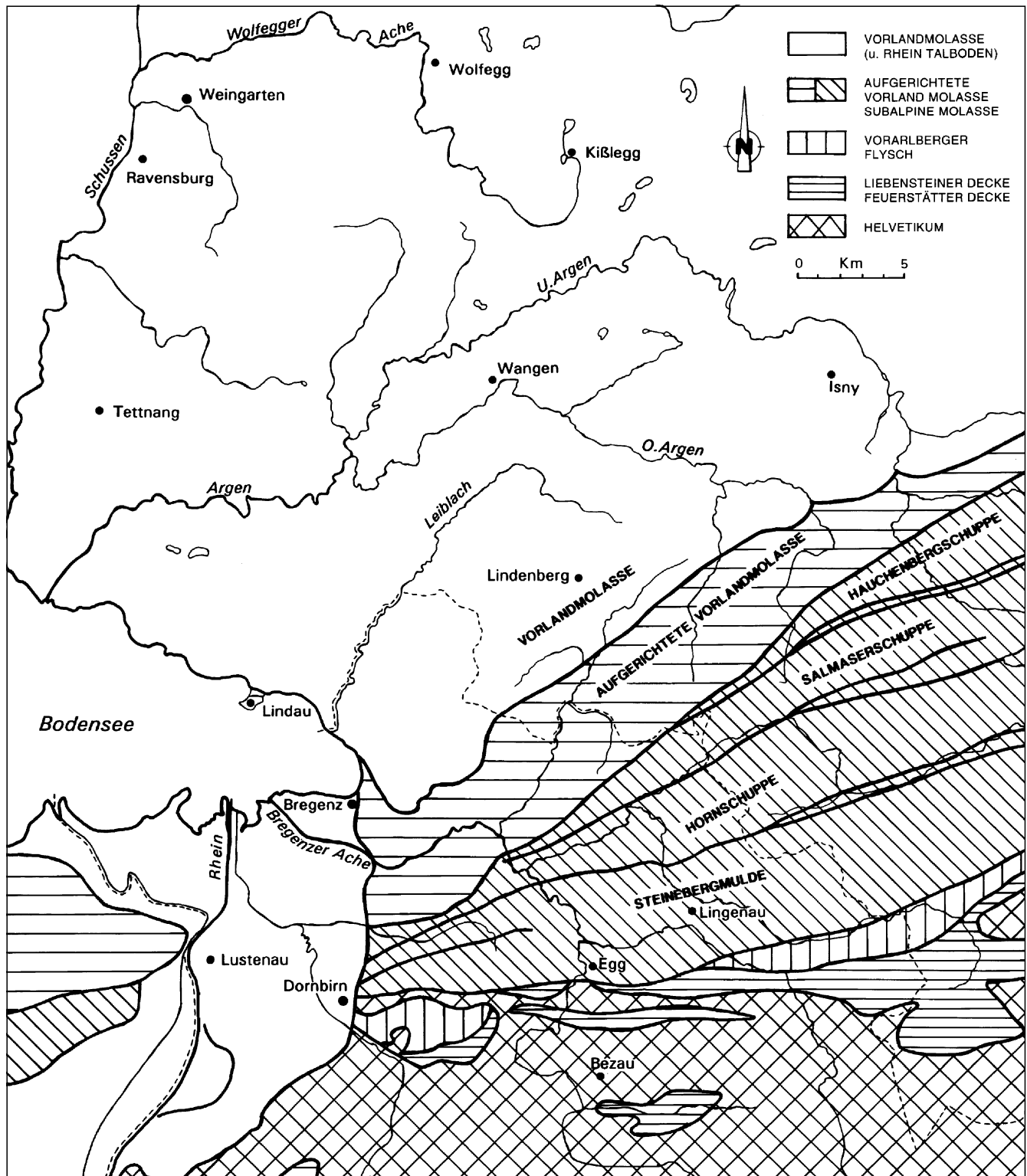
Abb. 3. Geologische Übersicht (nach GWINNER, 1978).
