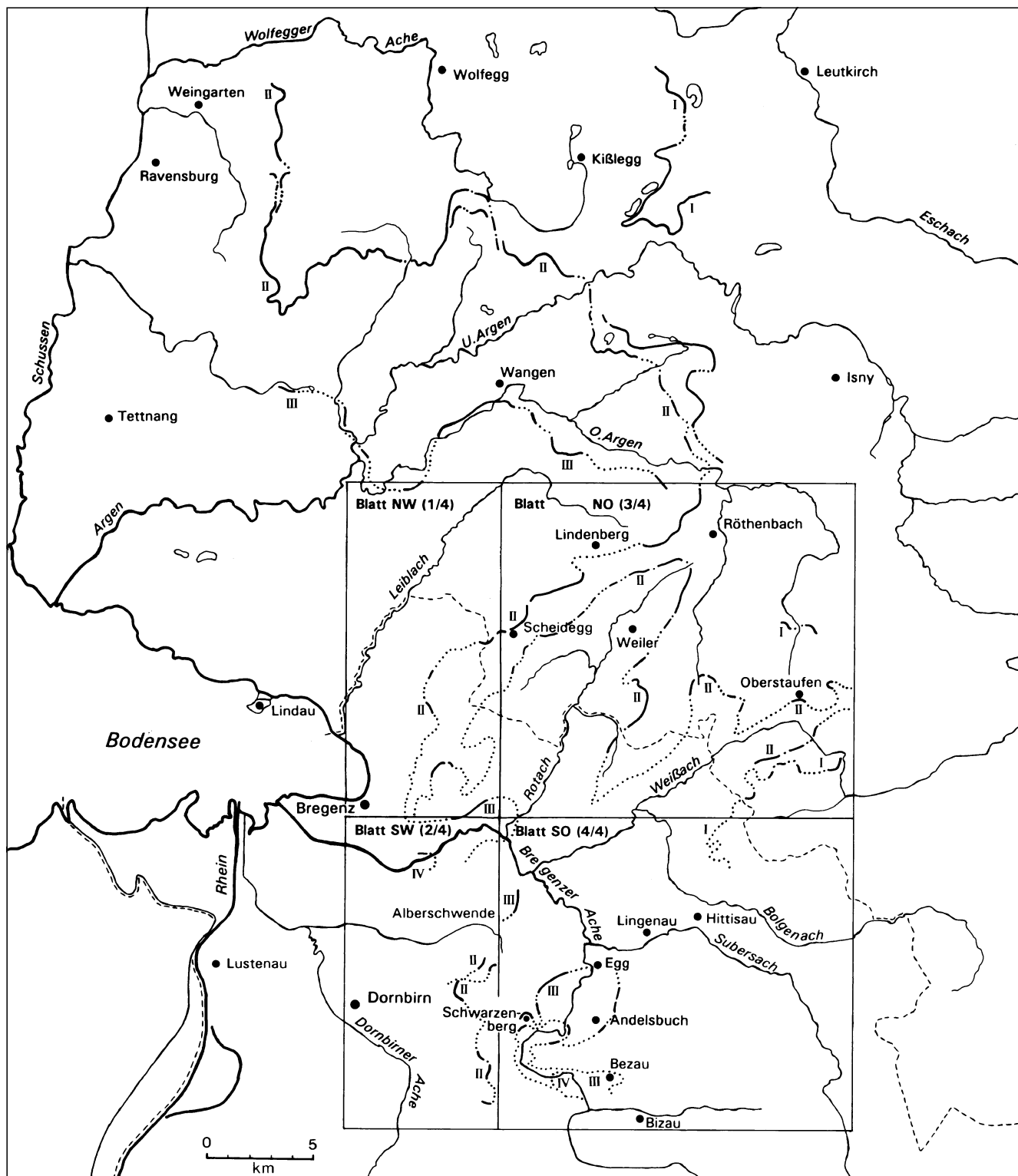
Abb. 1. Jüngste Teilstadien der vier Rückzugskomplexe und Lage der vier Kartenblätter mit globaler Umgrenzung des untersuchten Gebietes.
