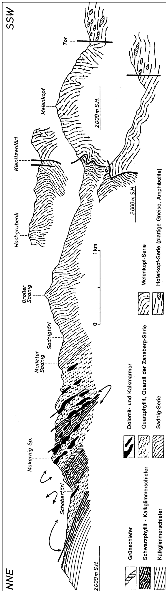
Abb. 4. Profil Makernig – Sadnig – Melenkopf.
