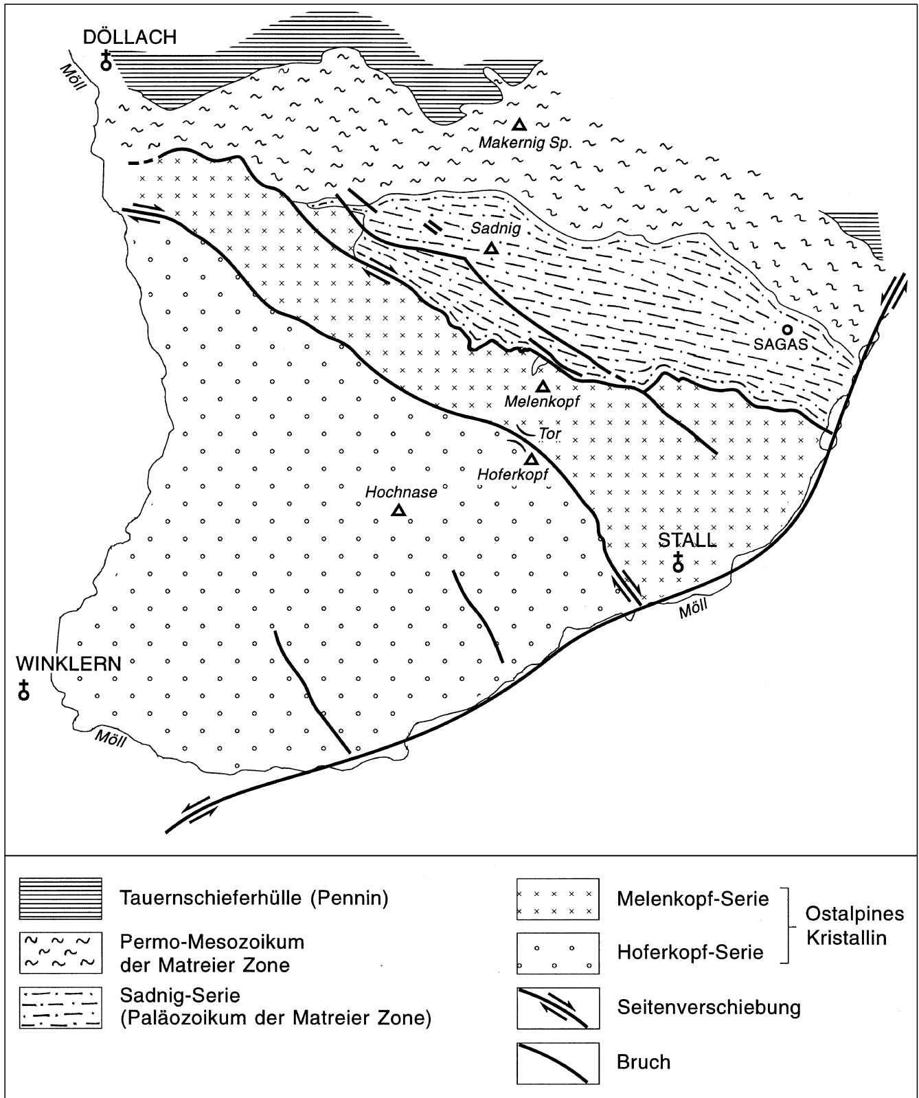
Abb. 3. Tektonische Übersicht der Sadnig-Gruppe.
