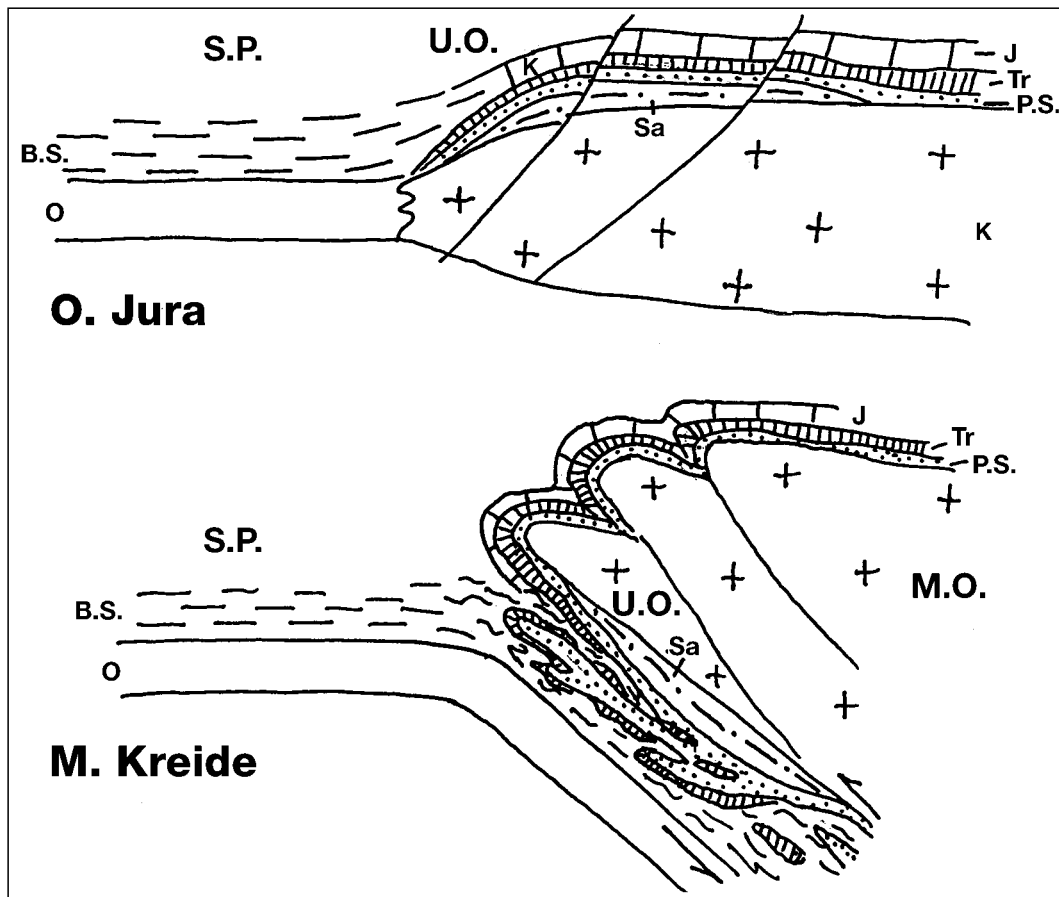
Abb. 5. Die frühalpide Entwicklung am Südrand des Südpenninischen Troges (S.P.).
